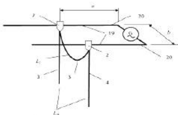
Рисунок 7с – Для испытательных устройств в соответствии с рисунками 2б и 2в
