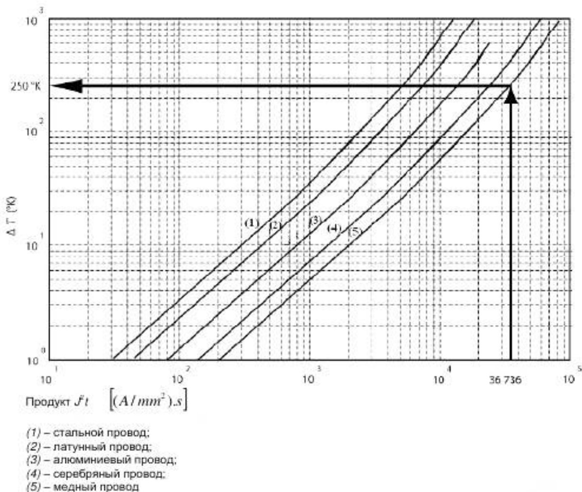
Рисунок С.2 – Определение температуры проводника в результате нагрева
