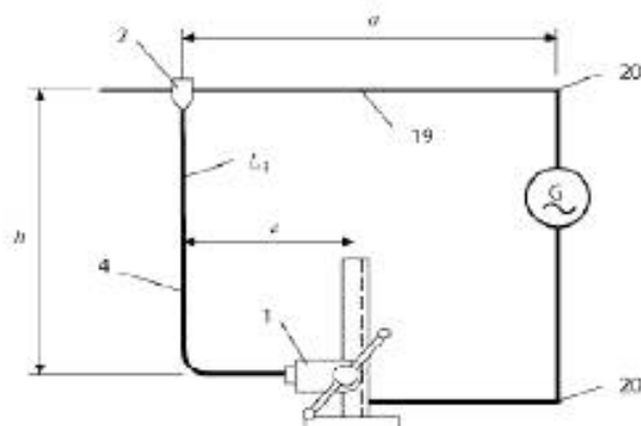
Рисунок 8а – Схема испытаний однополюсных устройств для подвесных линий однофазных систем и для открытых подстанций в соответствии с рисунком 2f
