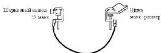
Рисунок 5а – Комбинация шарикового вывода и шины максимального размера
