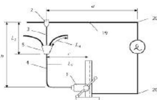
Рисунок 7d – Для испытуемого заземляющего кабеля в соответствии с рисунком 2а
