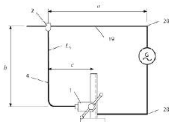
Рисунок 6f – Для испытуемых кабелей заземления согласно рисунку 3
