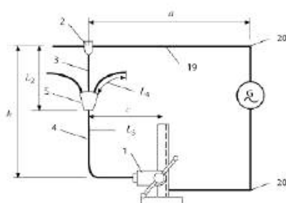
Рисунок 6f1 – Для испытуемых кабелей заземления согласно рисунку 2а
