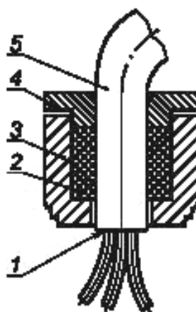
1 — точка разветвления проводников; 2 — уплотнительное кольцо; 3 — тепло кабельного ввода; 4 — зажимное кольцо с изогнутой хромкой; 5 — кабель
