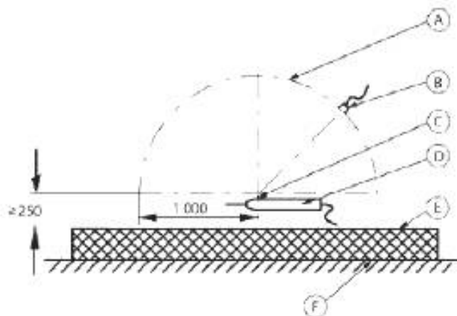
Рисунок 7а – Расположение индикатора напряжения в испытательном устройстве
