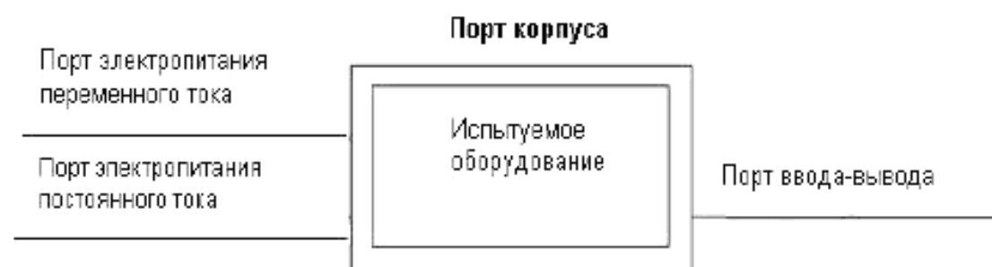
Рисунок 1 — Примеры портов оборудования
