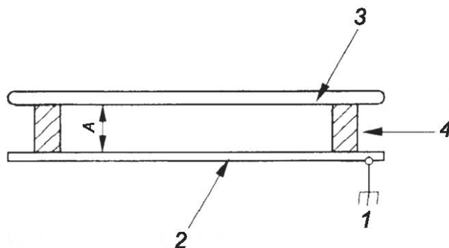
1 — линия заземления; 2 — заземленная поверхность со сторонами более 150 мм; 3 — проводящая пластина (номинальные размеры 150 \times 150 мм); 4 — изолирующие опоры
