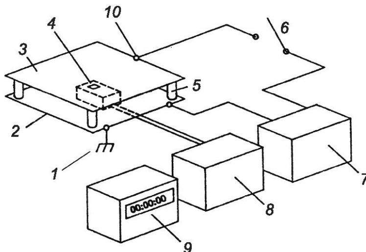
1 — линия заземления; 2 — заземленная поверхность со сторонами более 150 мм; 3 — проводящая пластина (например, с номинальными размерами 150 \times 150 мм); 4 — электрод; 5 — изолирующие опоры (сопротивление к заземлению более 10^{14} Ом); 6 — переключатель; 7 — высоковольтный источник питания с ограничителем тока; 8 — измеритель поля или соответствующее оборудование; 9 — таймер; 10 — высоковольтный контакт с пластиной
