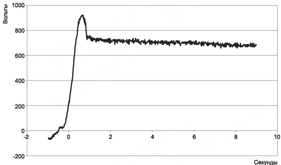
Рисунок В.2б — Электрическое напряжение тела, измеренное во время вставания с сиденья поочередно каждой ногой
