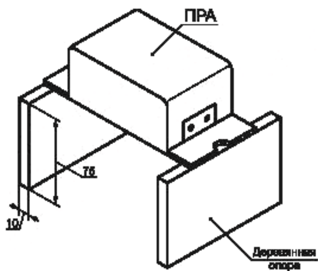
Рисунок Н.1 — Устройство для тепловых испытаний
