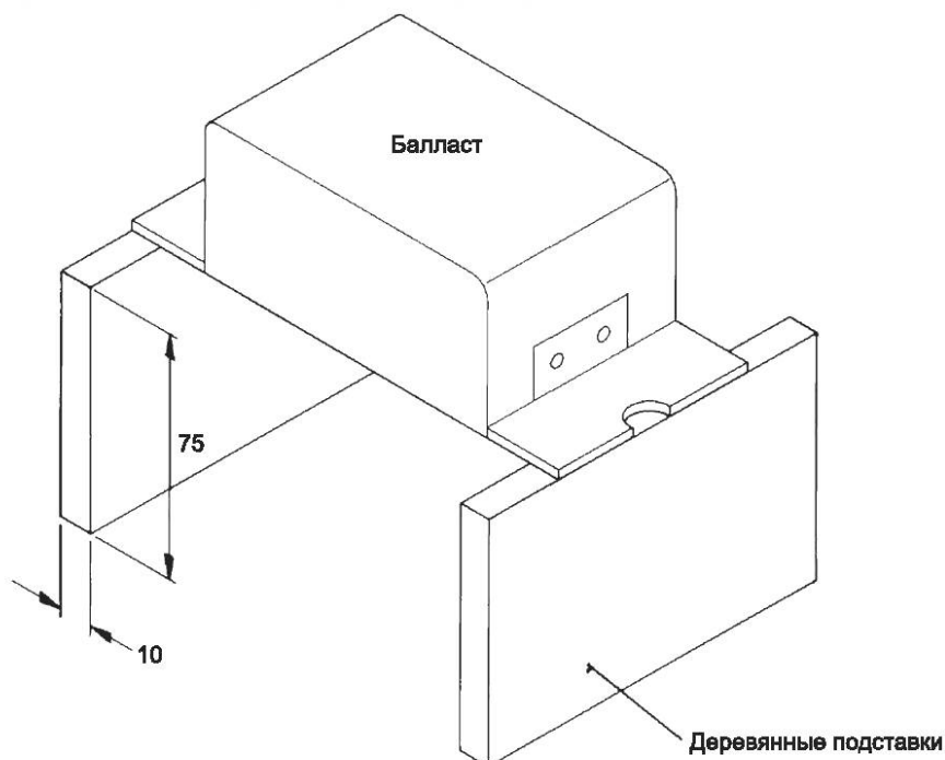
Рисунок Н.1 — Приспособление для испытания на нагрев
