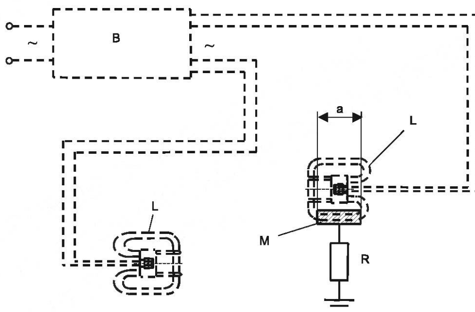
Рисунок I.1f — Схема испытаний для ламп с ILCOS FSS... и цоколем GR10q
