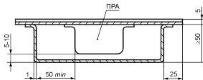
Рисунок J.1 — Испытательный кожух для тепловых испытаний ПРА
