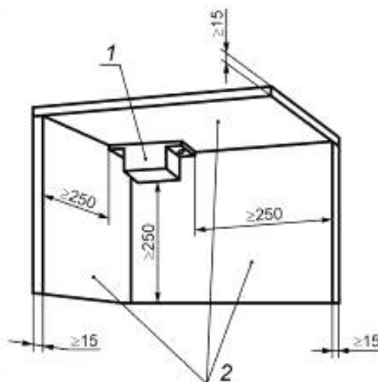
1 — ПРА; 2 — доски, покрытые матовой черной краской
