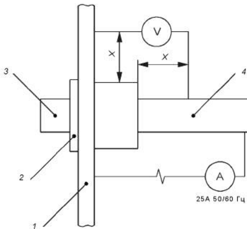
Рисунок 102 — Калибр для проверки минимального диаметра трубной системы после испытания на удар и на теплостойкость
