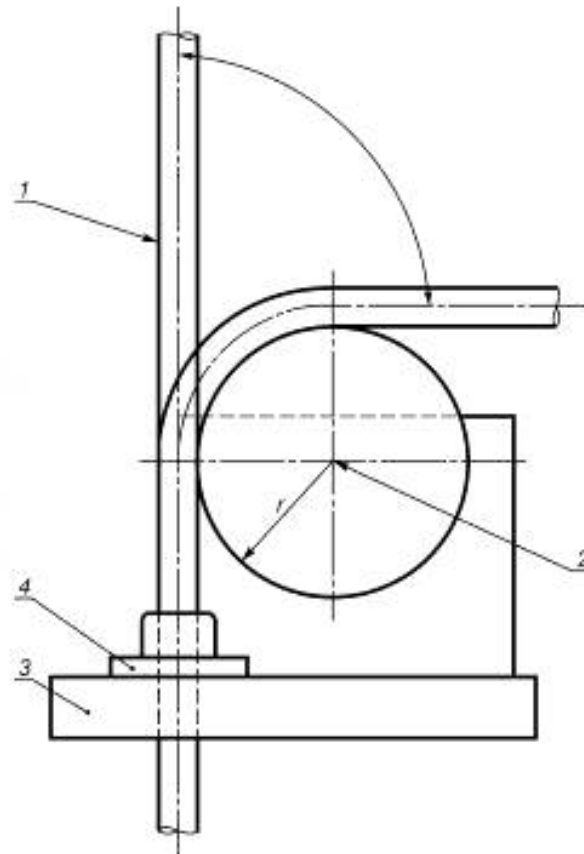
Рисунок 102 — Установка для испытаний на изгиб
