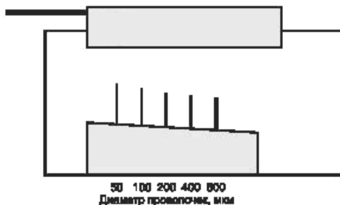
Рисунок В.3 — Тест-объект из проволоочек с плоскими торцами для определения локального динамического диапазона
