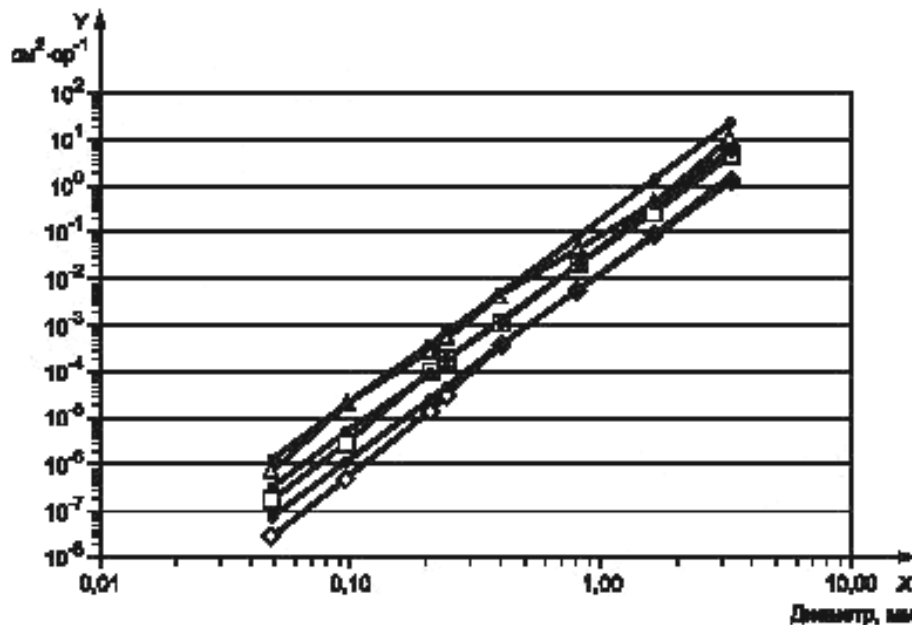
Рисунок В.4 — Зависимость экспериментально полученных значений площади поперечного сечения обратного рассеяния от плоского торца проволок из нержавеющей стали от их диаметра на частотах 9,6 МГц (Δ), 4,8 МГц (□) и 2,4 МГц (◇) [29]
