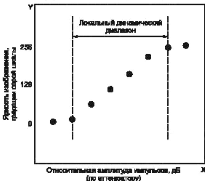
Рисунок 5 — Значения яркости оцифрованного изображения в зависимости от параметров attenuатора при измерении локального динамического диапазона с помощью внешнего акустического сигнала
