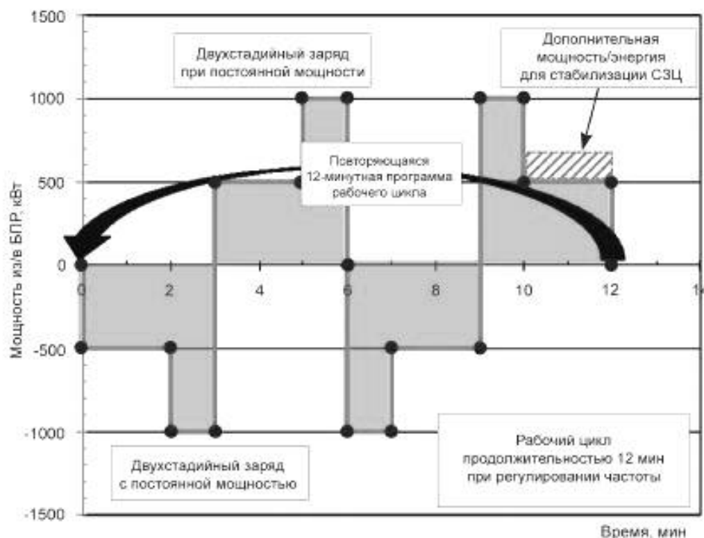
Рисунок 6 — Профиль программы работы в режиме регулирования частоты (см. 6.2) — профиль а
