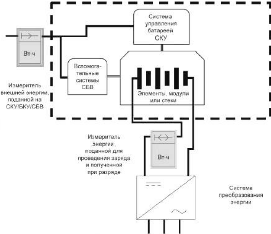
Рисунок 18 — Схематичное представление расположения двух точек измерения энергии (энергии, поданной вспомогательным системам, и энергии, поданной в батарею) для определения потребностей в ней в период режима ожидания батареи
