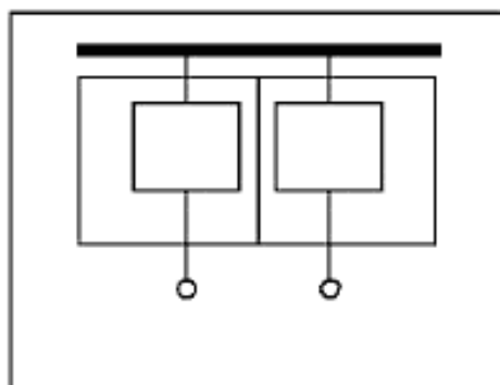
Вид 3a — Зажимы не отгорожены от шин
