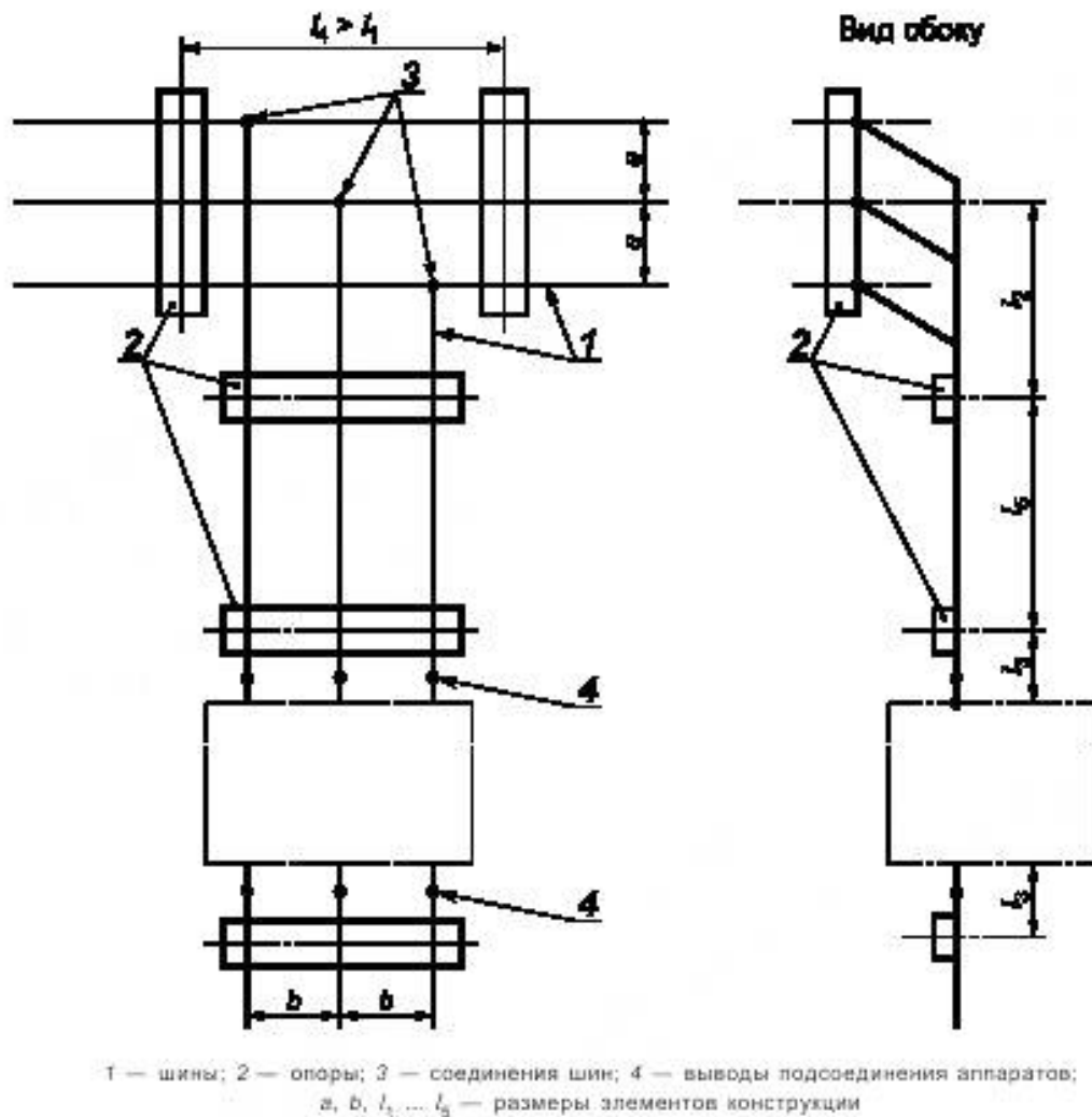
Рисунок Р.2 — Не испытанная конструкция шин (НИК)
