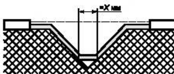
Рисунок F.1c) — Пример 2
