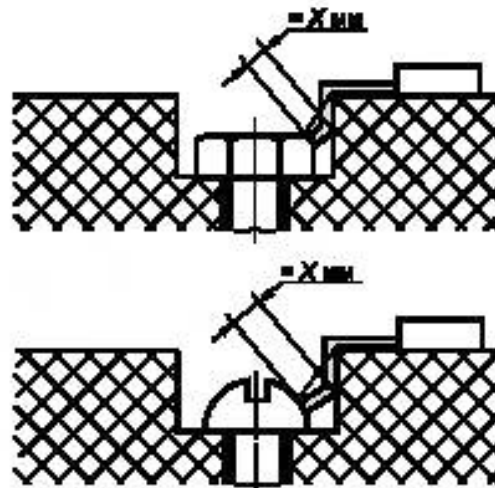
Рисунок F.1j) — Пример 9
