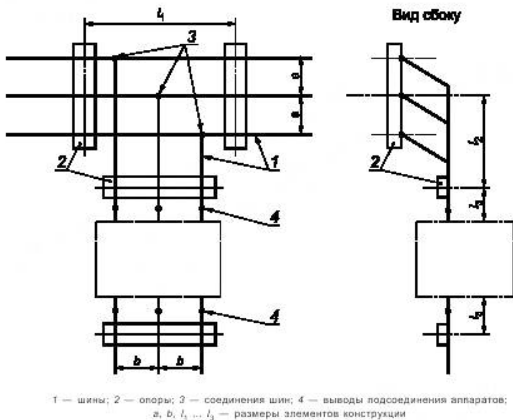
Рисунок Р.1 — Испытанная конструкция шин (ИК)
