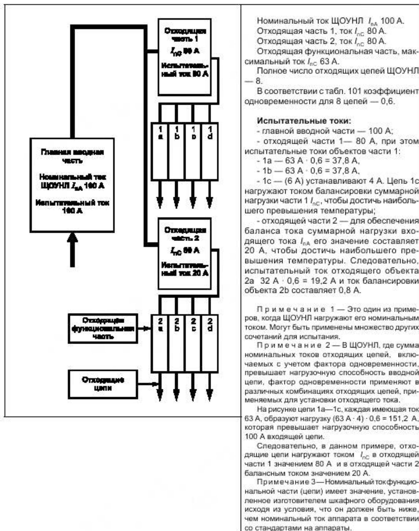
Рисунок 101 — Пример подтверждения превышения температуры испытанием комплектного ЩОУНЛ в соответствии с 10.10.2.3.6
