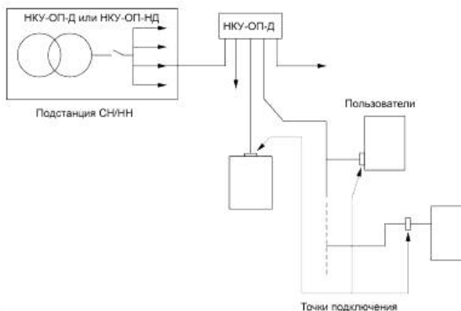
Рисунок 101 — Типичная распределительная система
