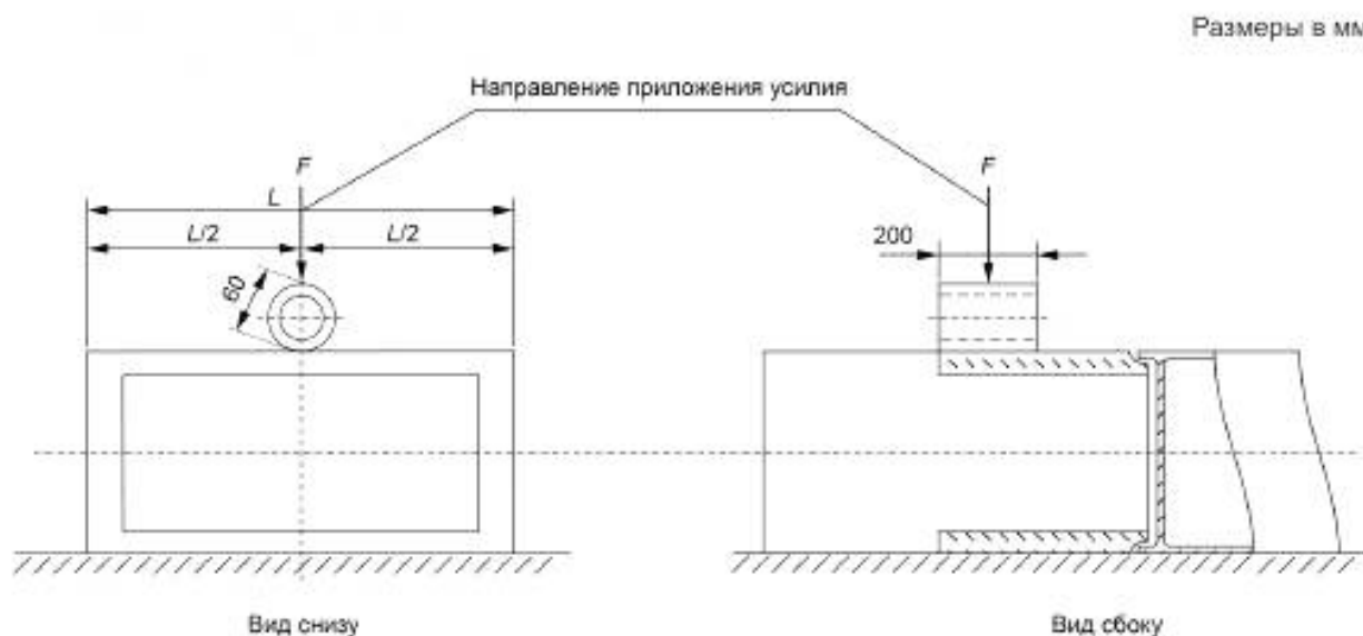
Рисунок 109 — Типовая испытательная установка для механических испытаний основания
