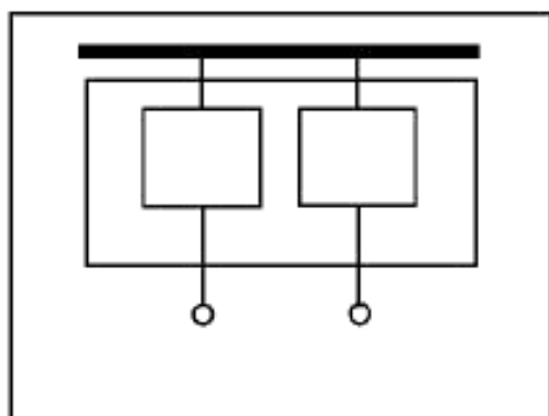
Пример 2a - Зажимы для внешних проводников не отгорожены от сборных шин
