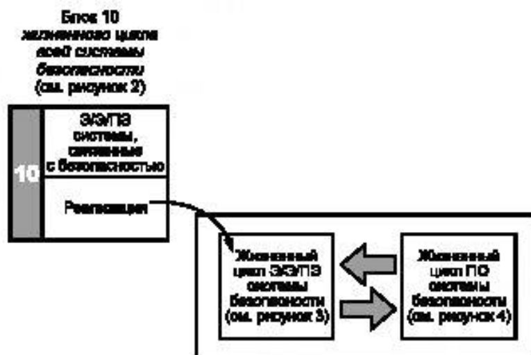
Рисунок 5 — Соотношение между жизненным циклом всей системы безопасности и жизненными циклами ЭЗ/ПЗ системы безопасности и программного обеспечения (ПО) системы безопасности
