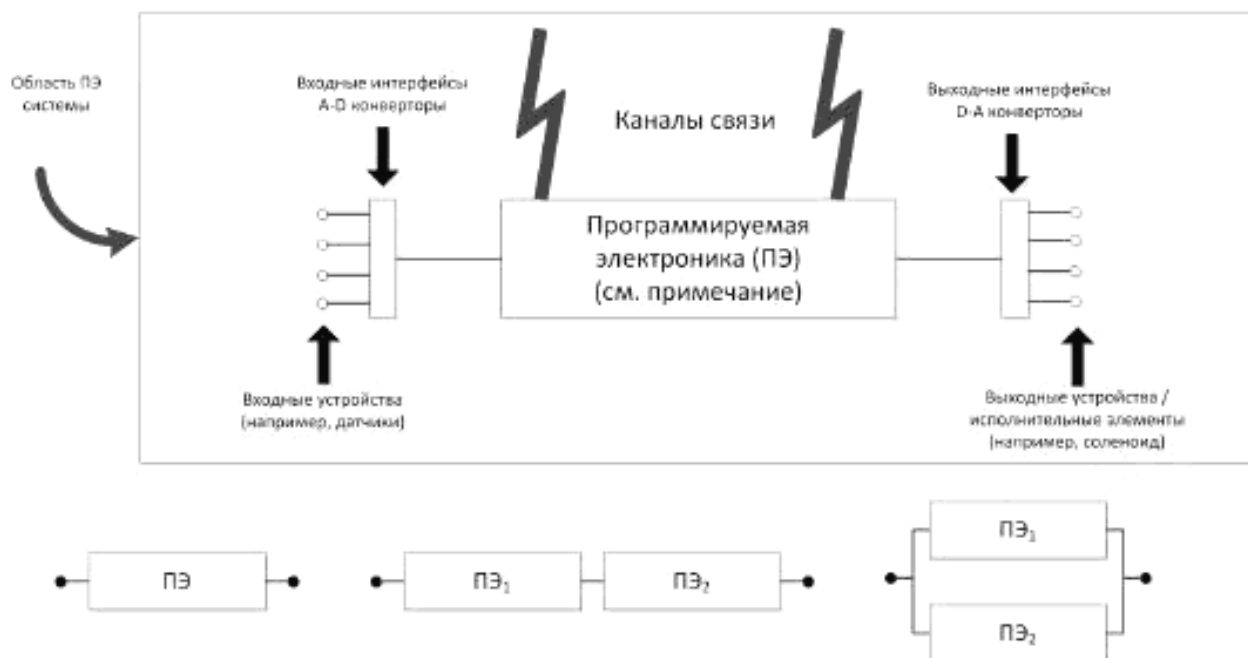
а) Структура базовой ПЭС
