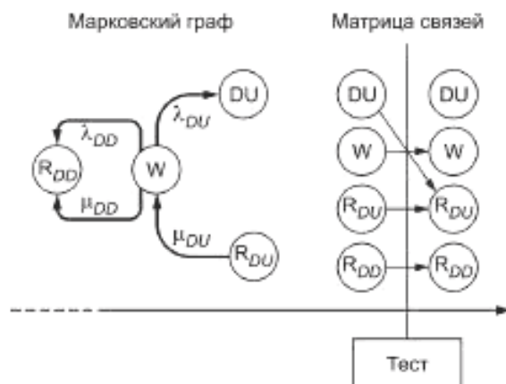
Рисунок В.29 — Многофазная модель Маркова с отказами DD и DU
