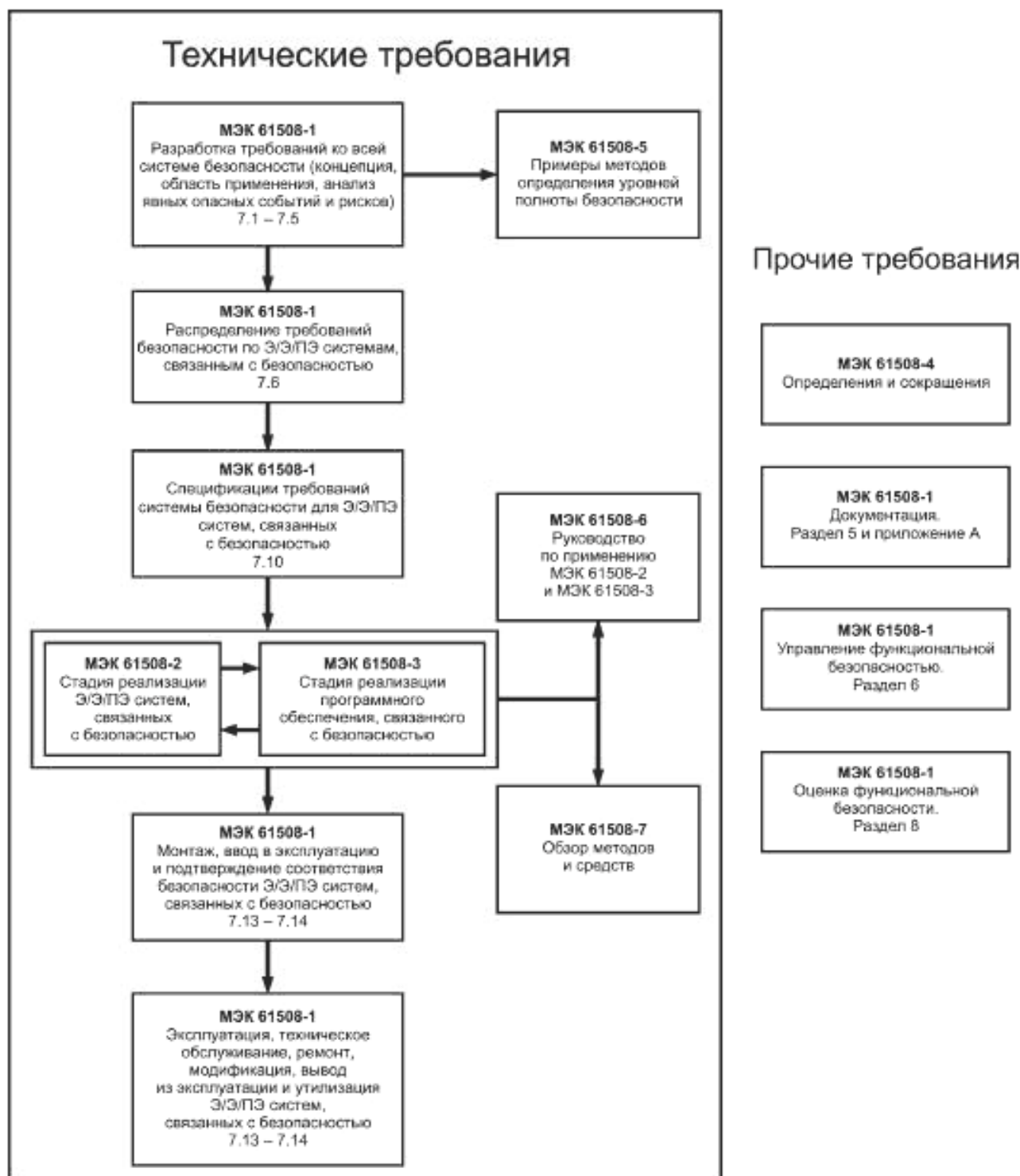
Рисунок 1 — Общая структура серии ГОСТ Р МЭК 61508
