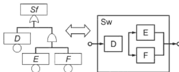
Рисунок В.18 — Эквивалентность дерева отказов и блок-схемы надежности
