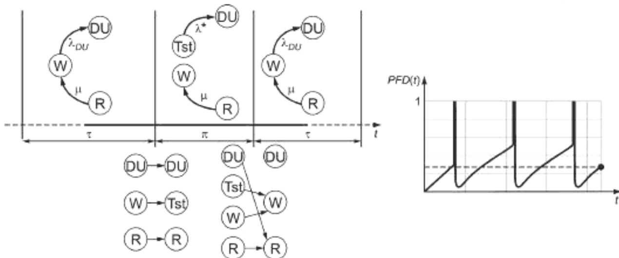
Рисунок В.28 — Моделирование влияния длительности проверки
