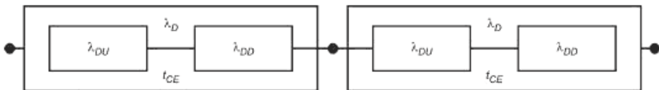
Рисунок В.9 — Структурная схема надежности для архитектуры 2oo2
