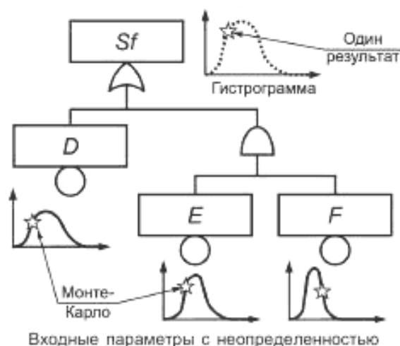
Рисунок В.38 — Принцип распространения неопределенности
