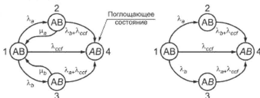
Рисунок В.31 — Марковский граф «надежности» с поглощающим состоянием
