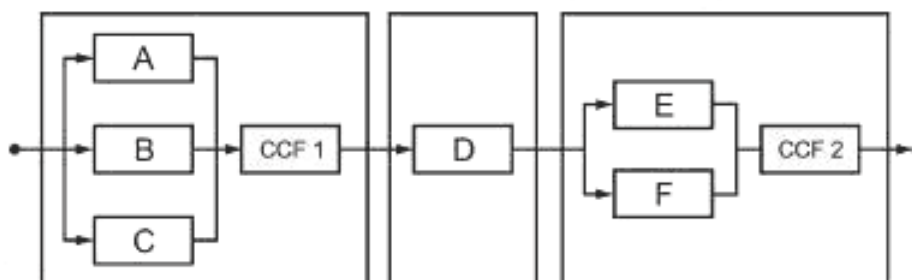
Рисунок В.1 — Блок-схема надежности всей системы безопасности
