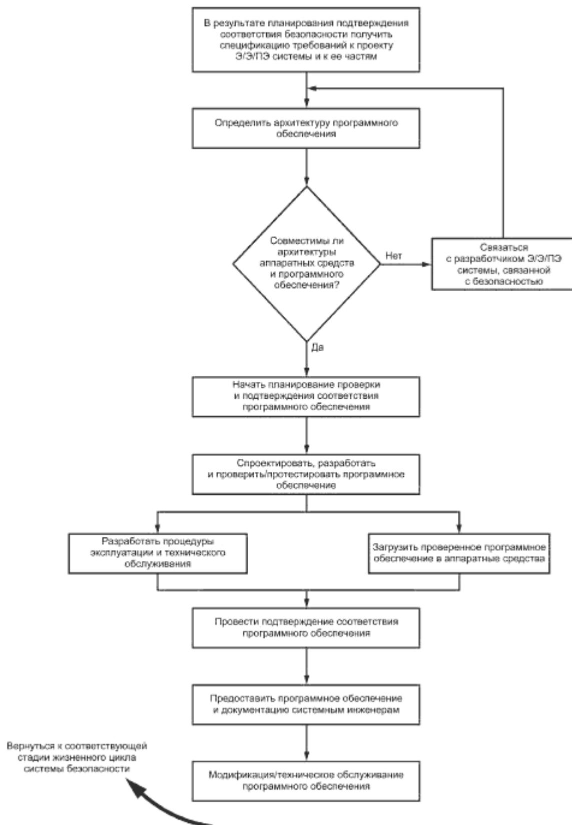
Рисунок А.3 — Функциональные этапы применения МЭК 61508-3
