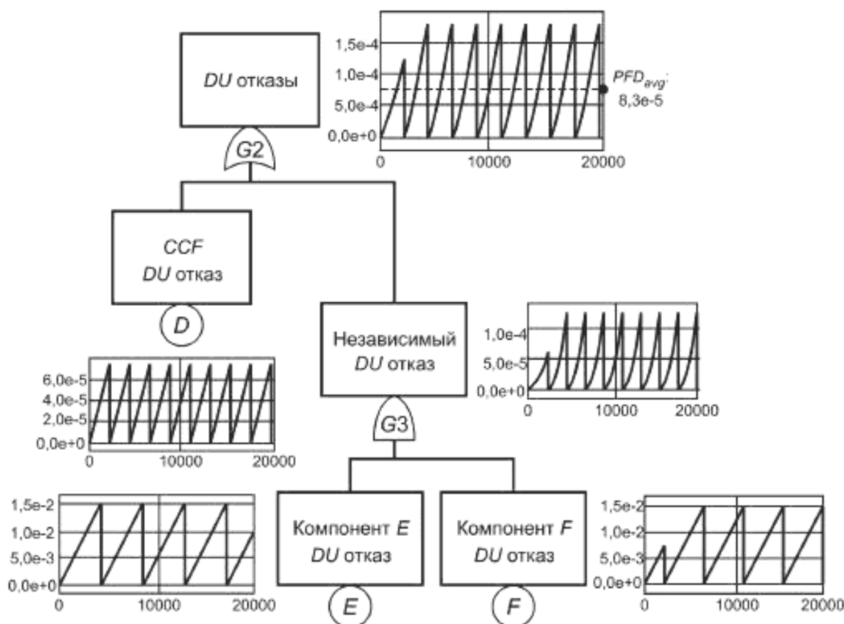
Рисунок В.21 — Влияние смещения проверок
