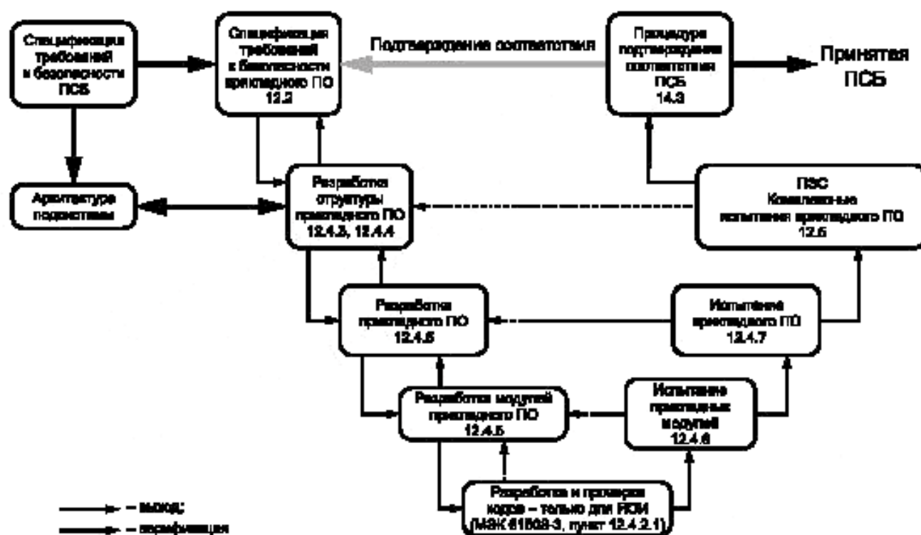
Рисунок 12 — Жизненный цикл разработки ПО (V-образная модель)
