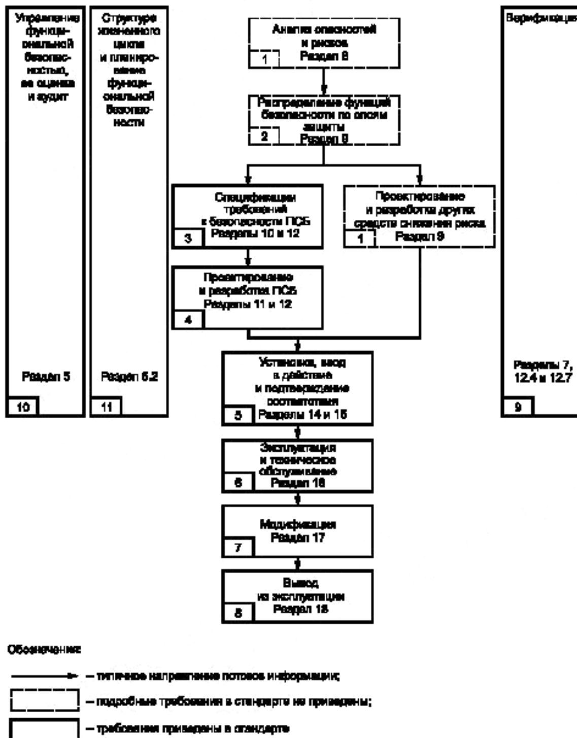
Рисунок 8 — Стадии жизненного цикла безопасности и стадии оценки функциональной безопасности ПСБ
