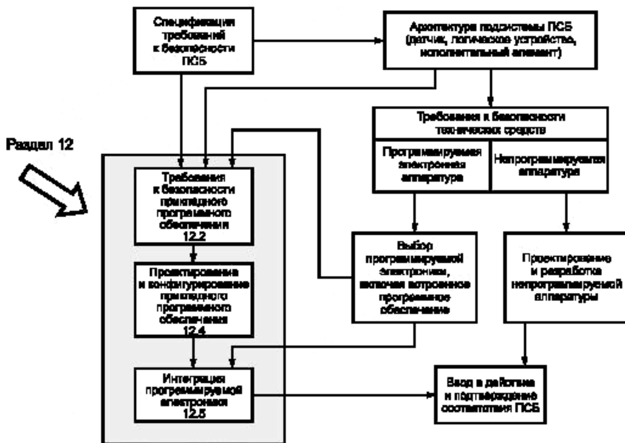
Рисунок 10 — Жизненный цикл безопасности прикладного ПО и его связь с жизненным циклом безопасности ПСБ
