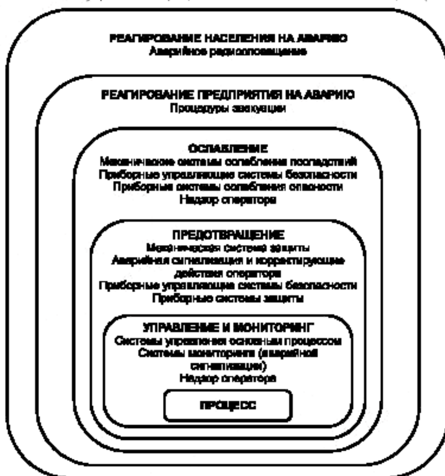
Рисунок 9 — Типовые методы снижения риска, используемые в промышленных процессах на предприятиях
