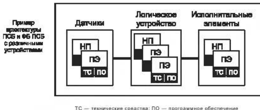
Рисунок 6 — Пример архитектуры ПСБ, включающей три подсистемы ПСБ
