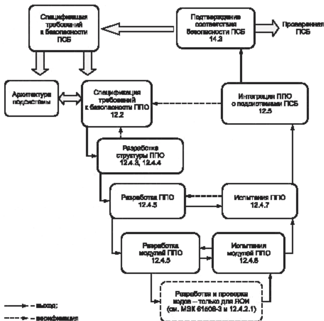
Рисунок 3 — Жизненный цикл разработки ПО (V-модель)
