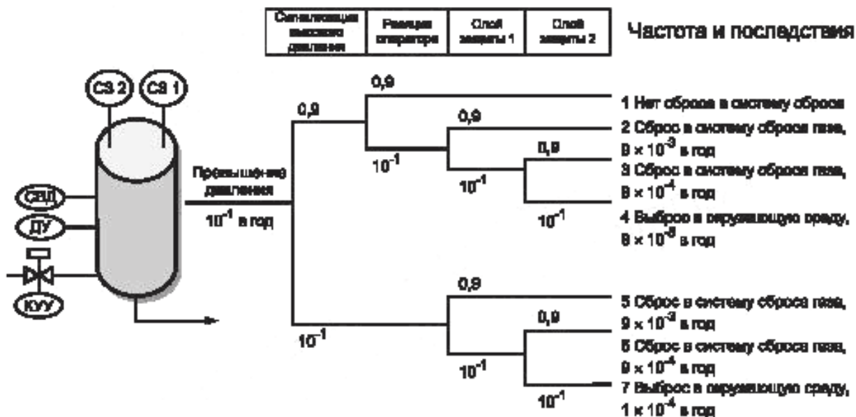
Рисунок В.4 — Опасные события при резервированном слое защиты
