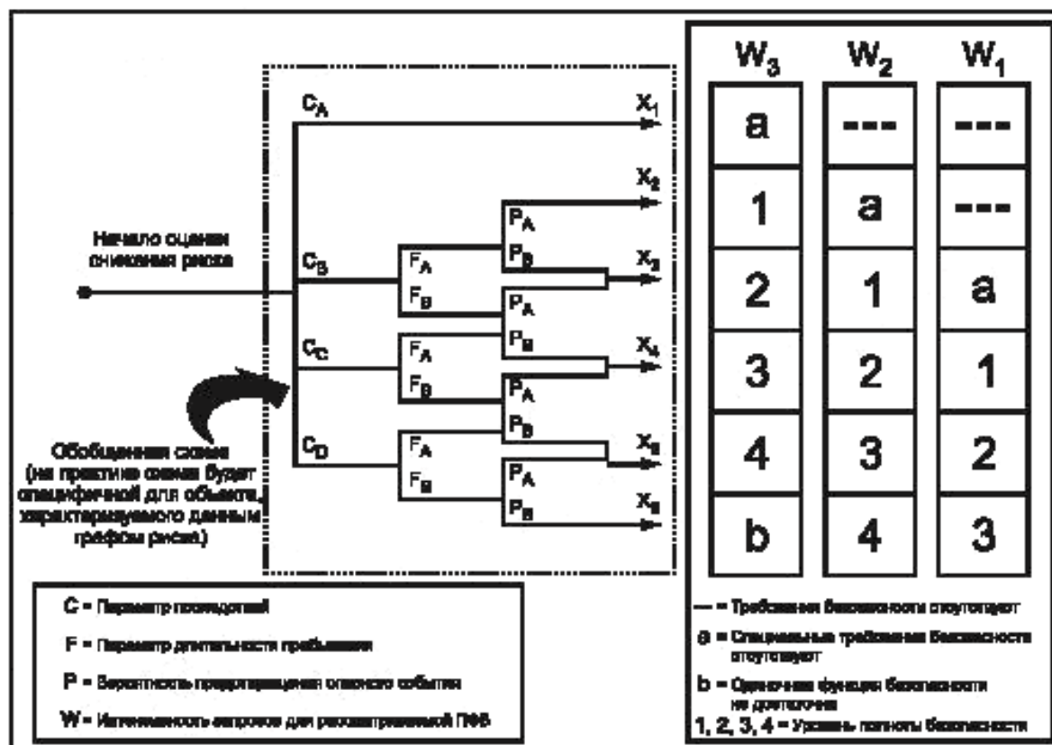
Рисунок D.1 — Граф риска, общая схема
