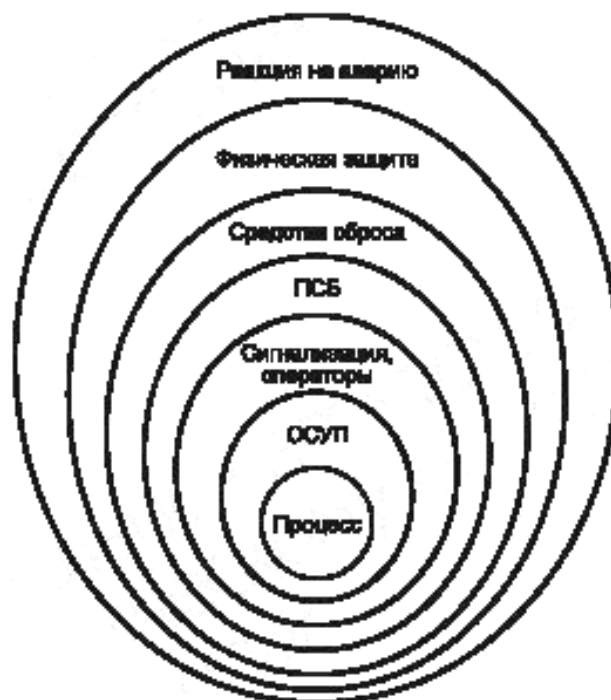
Рисунок С.1 — Слои защиты
