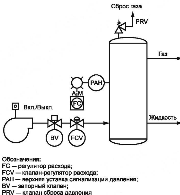
Рисунок В.1 — Емкость под давлением с существующими системами безопасности
