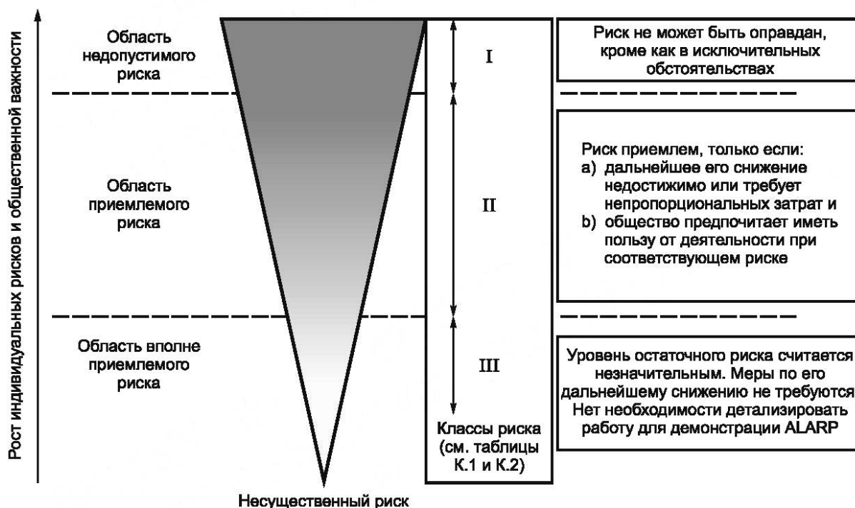
Рисунок К.1 — Приемлемый риск и принцип ALARP
