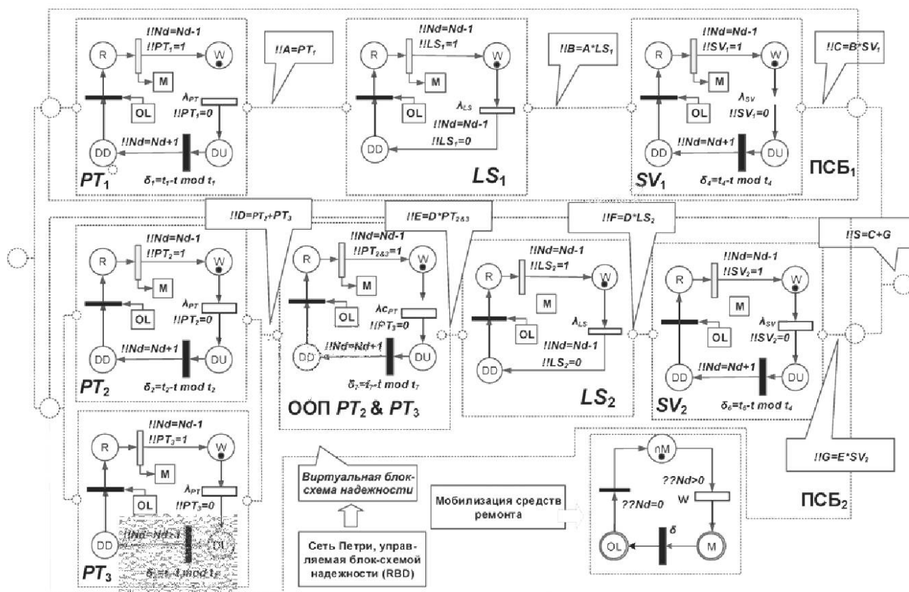
Рисунок J.10 — Моделирование привлечения ресурса ремонта
