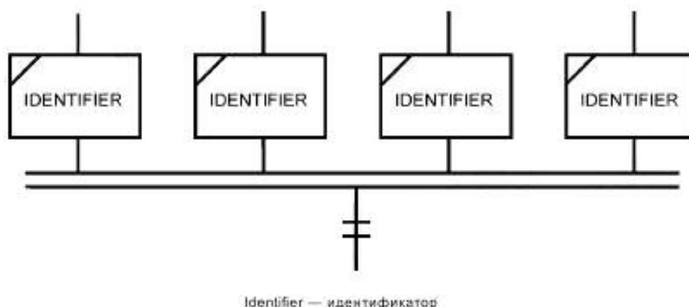
Рисунок 32 — Окончание параллельных последовательностей
