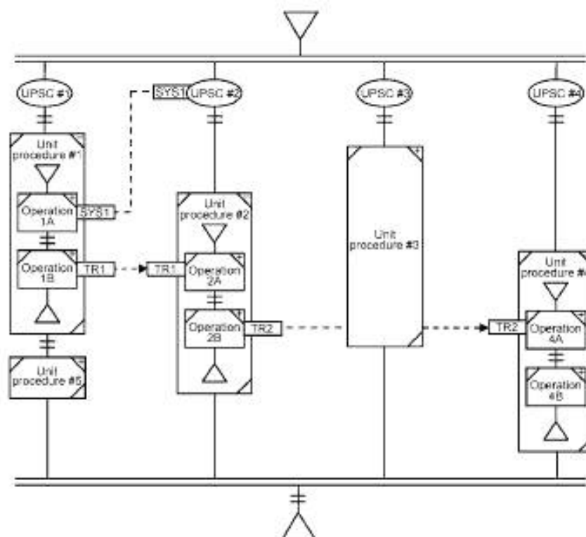
Рисунок 38 — Отношения между процедурными сущностями
