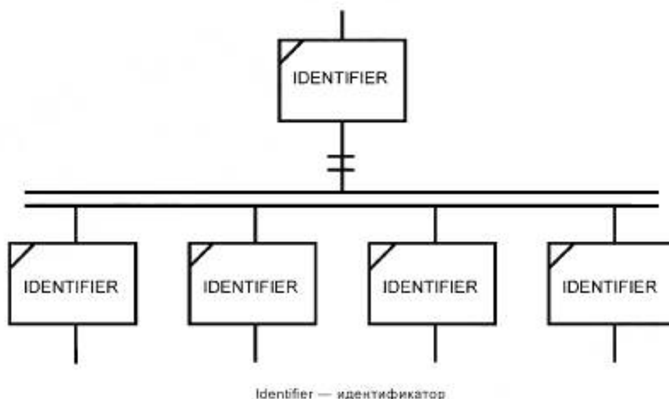
Рисунок 31 — Начало параллельной последовательности
