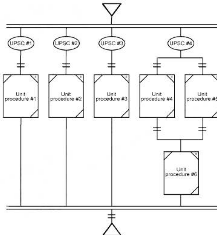
Рисунок 37 — Отображение процедуры технологической установки и ее инициализации
