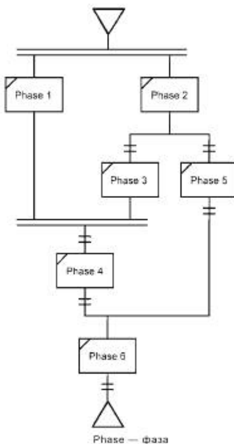
Рисунок 36 — Некорректная процедурная функциональная диаграмма
