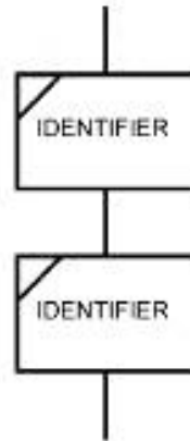
Рисунок 27 — Неявный переход
