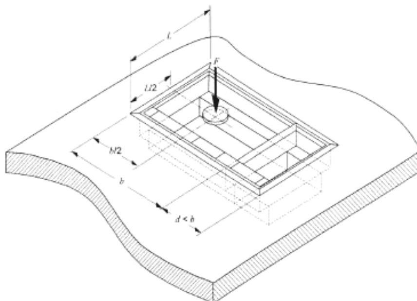
Рисунок 102 – Испытание напольных сервисных блоков, установленных заподлицо с полом, нагрузкой от движущегося транспорта, приложенной к небольшой площади поверхности
