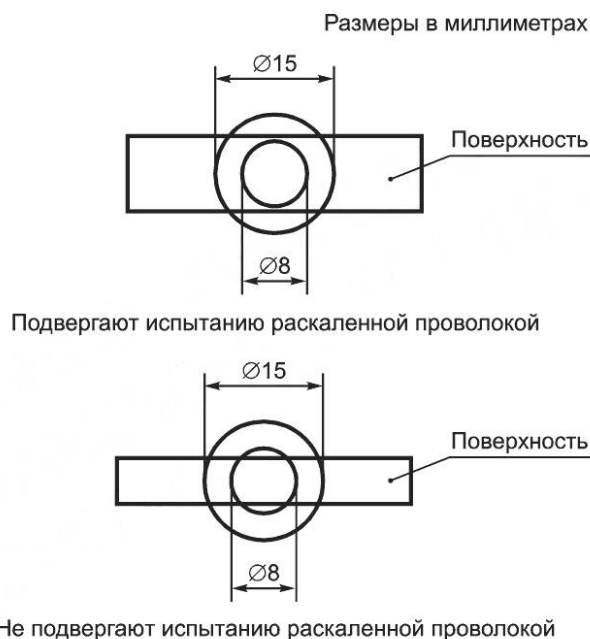
Рисунок 4 — Метод определения поверхности «мелких частей»
