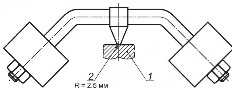
1 — образец; 2 — сферическая поверхность R = 2,5 \text{ мм}
