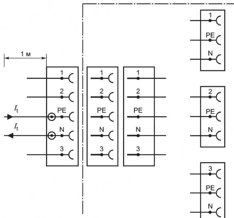
Рисунок В.6 — Испытательная схема соединения 3P+N+PE — 1P+N+PE распределительных щитов, N и PE под нагрузкой
