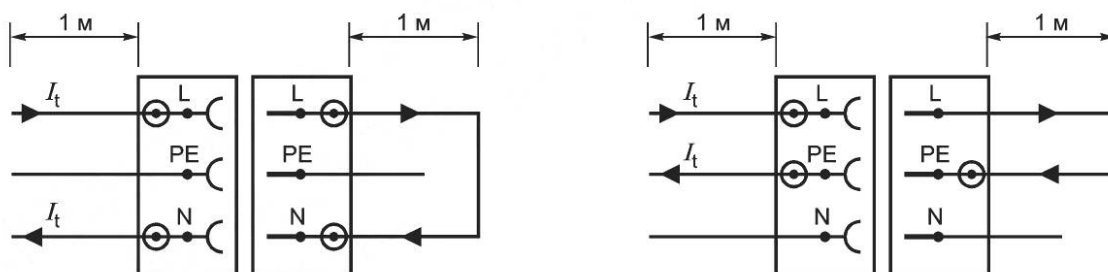
Рисунок В.1 — Испытательная схема соединения 1P+N+PE установочных соединителей, N (рисунок слева), PE (рисунок справа)
