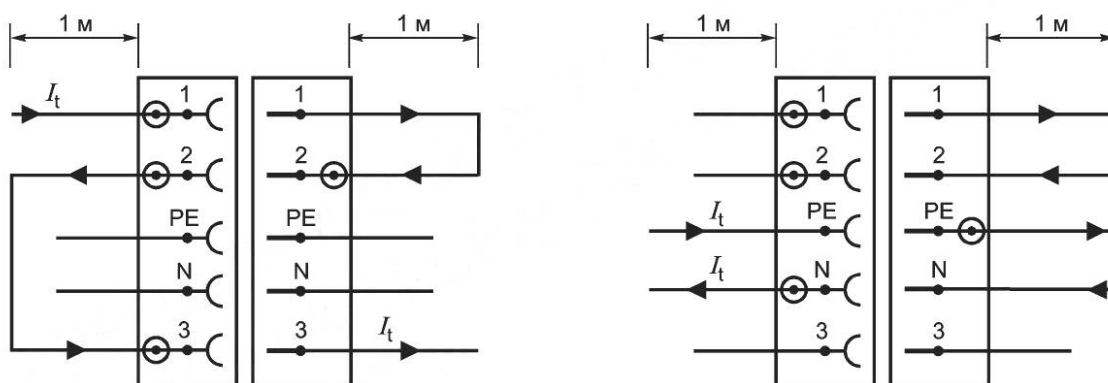
Рисунок В.2 — Испытательная схема соединения 3P+N+PE установочных соединителей, три фазы под нагрузкой (рисунок слева), N и PE под нагрузкой (рисунок справа)
