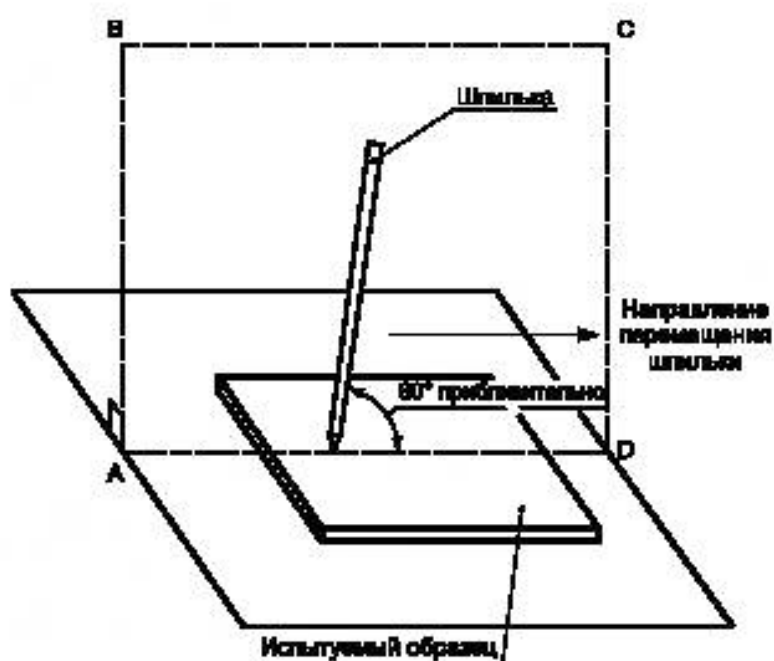
Рисунок 4 — Испытание на соскребание покрытых изоляцией слоев
