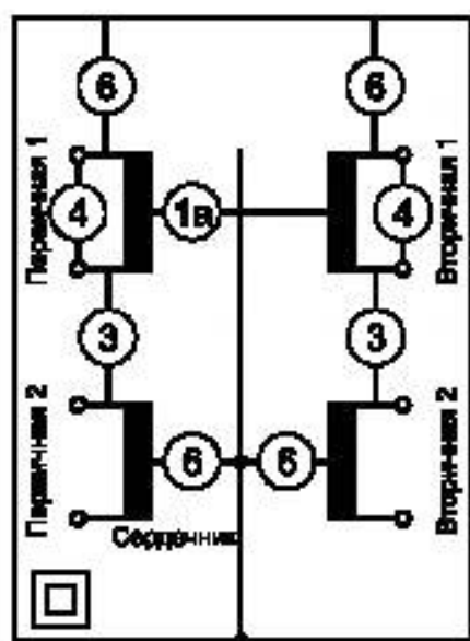
а) Сердечник, соединенный с корпусом
