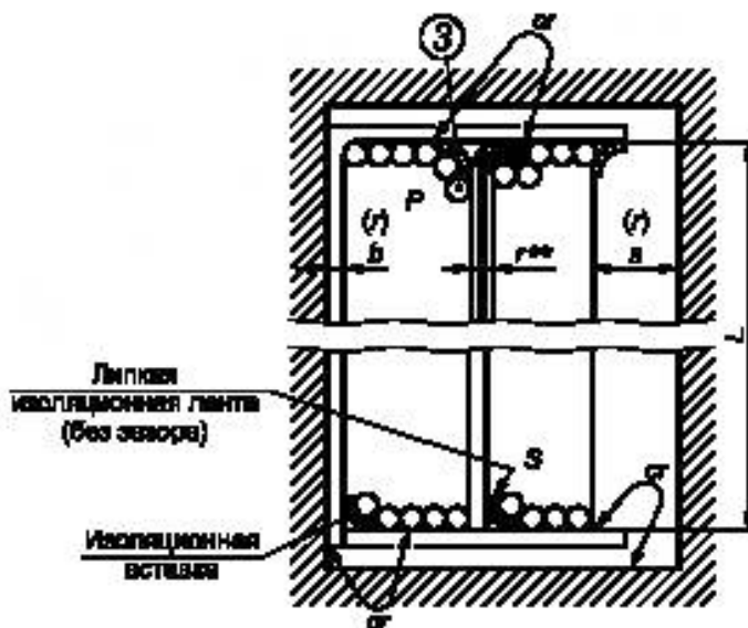
Класс I (II) М.2.1 б)
