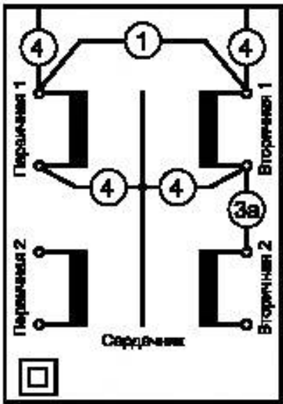
а) Сердечник, соединенный с корпусом
