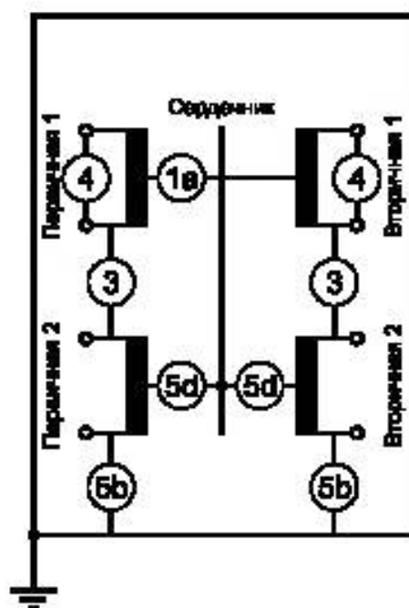
б) Сердечник, не соединенный с корпусом
