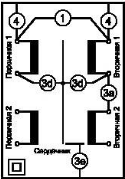
б) Сердечник, не соединенный с корпусом
