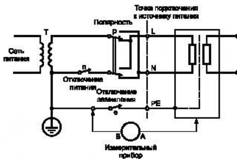
Рисунок В — Испытательная установка: однофазное оборудование систем питающих сетей типа TN или TT
