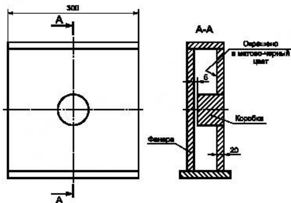
Рисунок 1 — Монтажная коробка для щитовых трансформаторов (см. 5.10)
