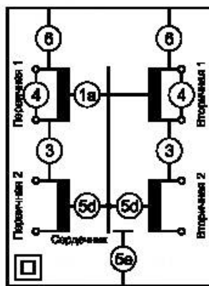
б) Сердечник, не соединенный с корпусом
