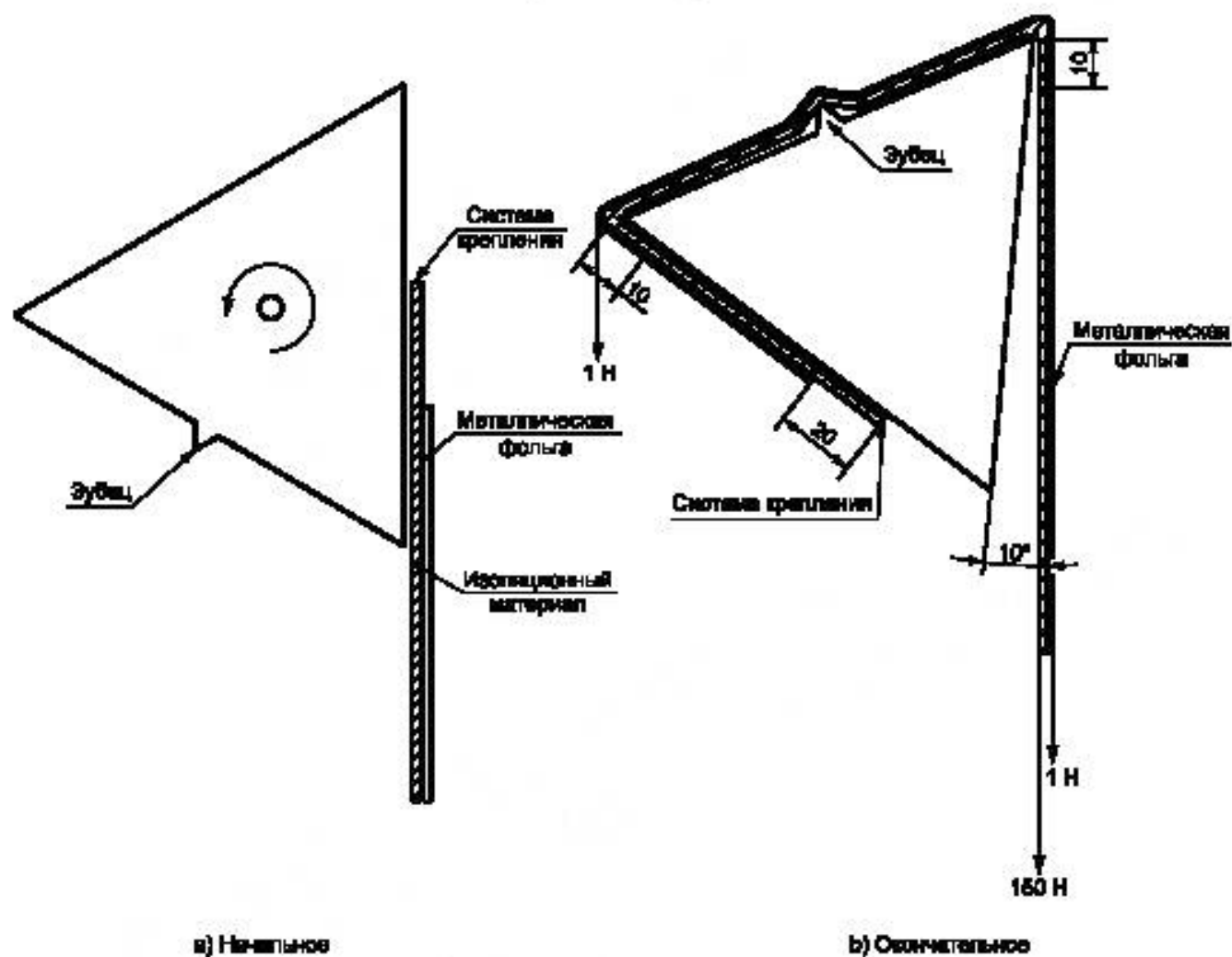
Рисунок 6б — Положение оправки
