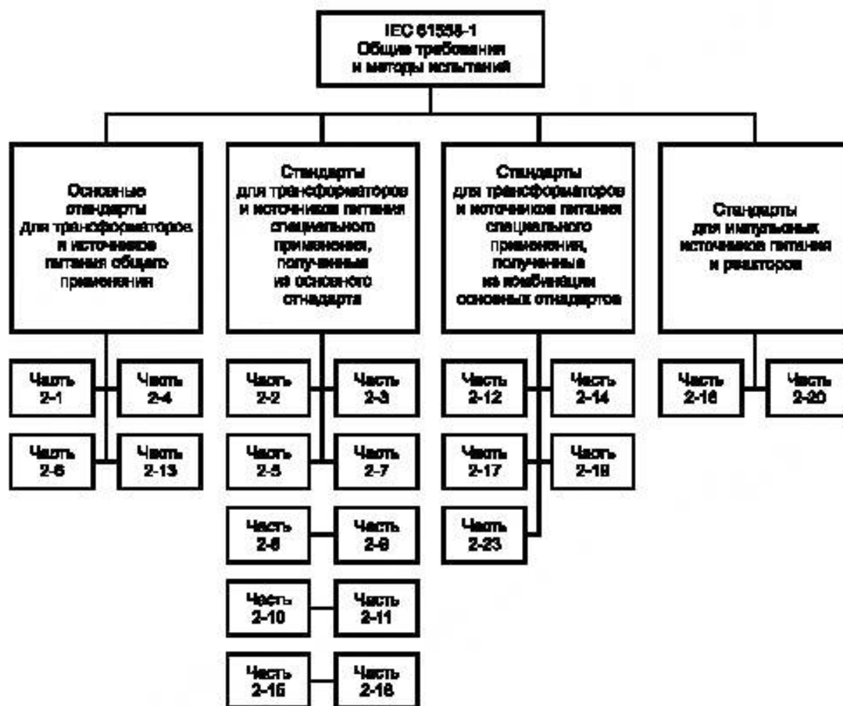
Рисунок 0 — Принцип построения стандартов серии IEC 61558
