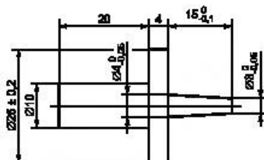
Рисунок 3 — Испытательный стержень [см. 9.2, 15.5.2 и IEC 61032 (испытательный пробник 13)]
