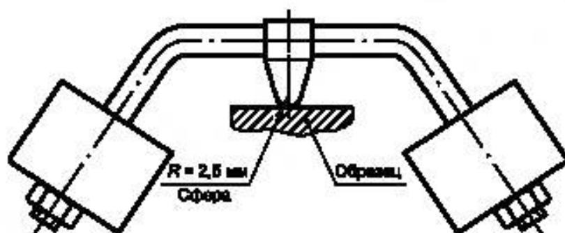
Рисунок 5 — Устройство для вдавливания шарика (см. 27.1)
