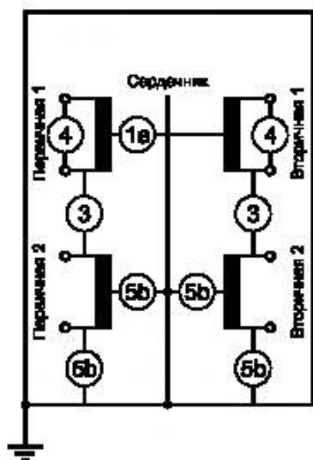
а) Сердечник, соединенный с корпусом
