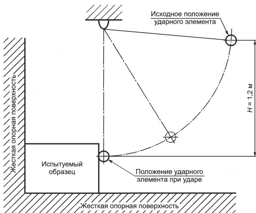
Рисунок 102 — Испытание на удар вертикальной поверхности
