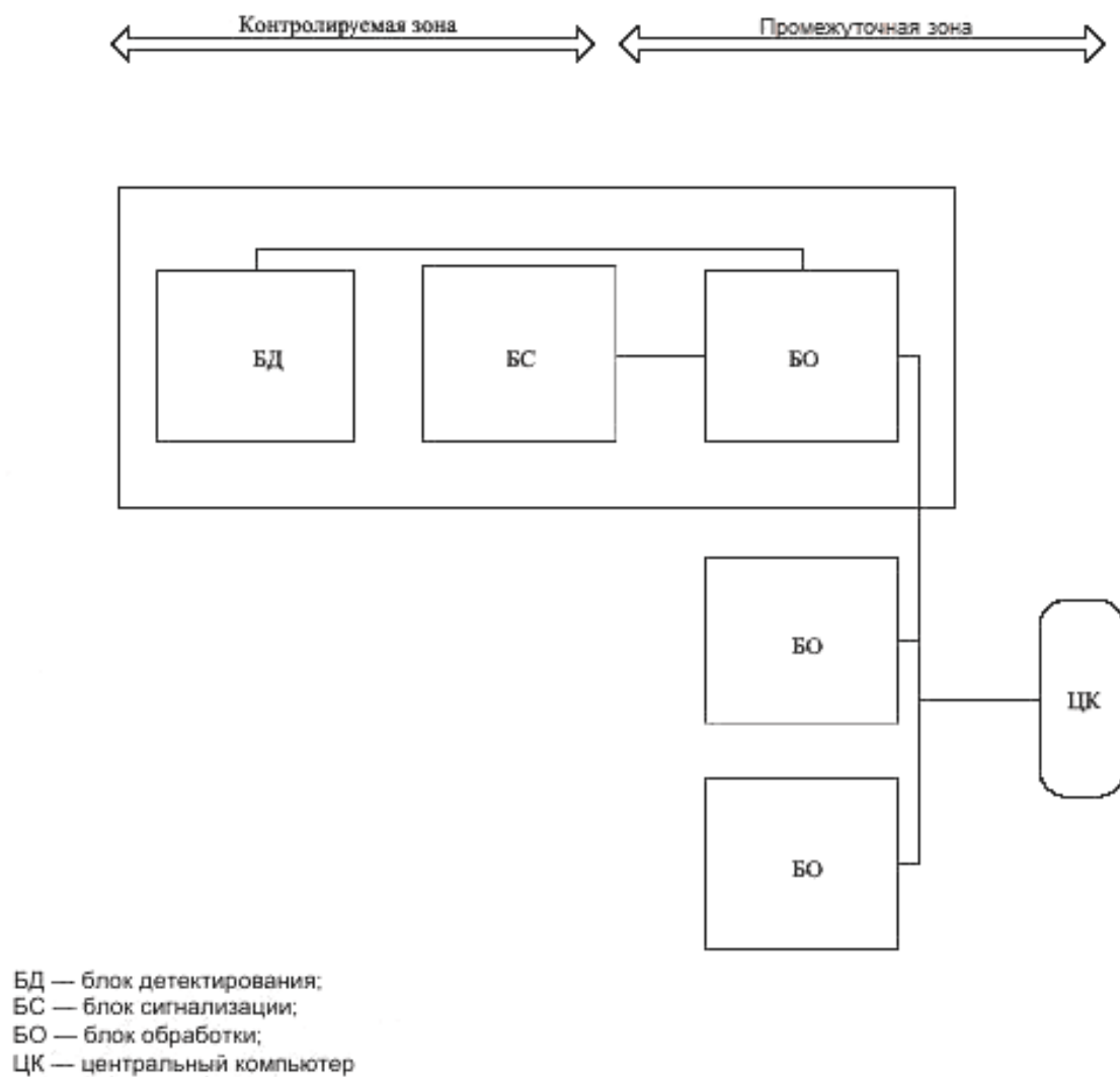
Рисунок 4 — Централизованная конфигурация
