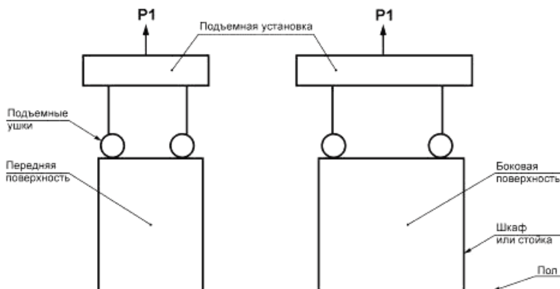
Рисунок 1 — Испытание на подъем для шкафов и стоек
