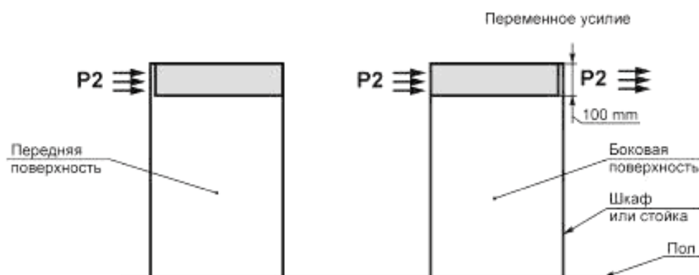
Рисунок 2 — Испытание шкафов и стоек на жесткость
