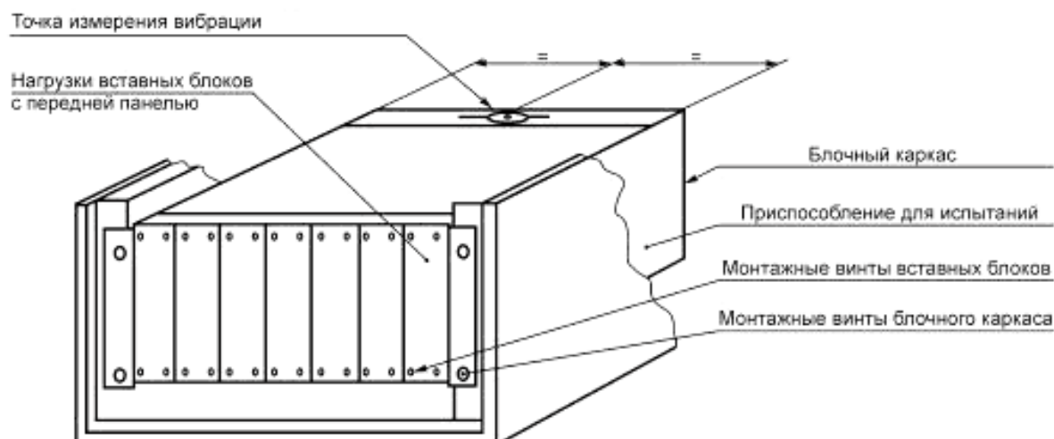
Рисунок 9 — Условия установки блочных каркасов для испытаний на ударное воздействие и вибрацию
