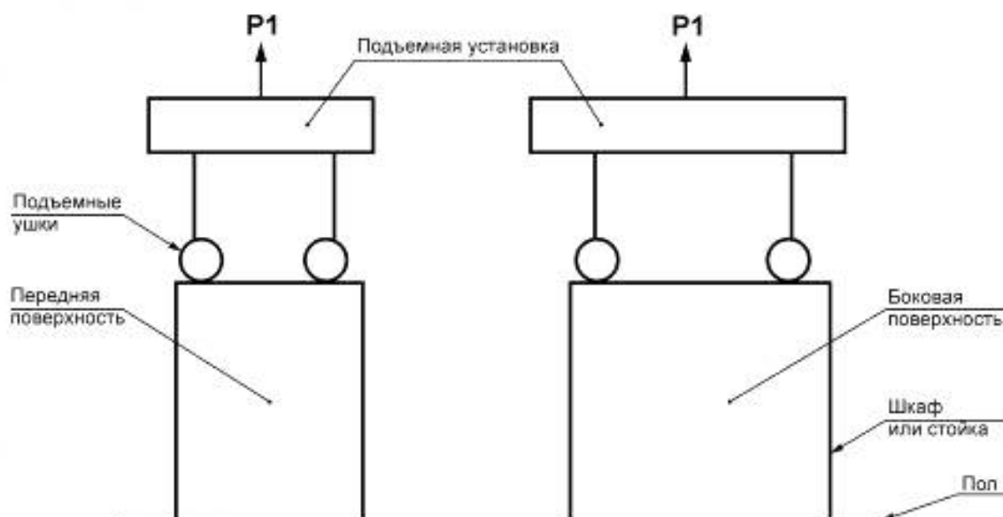
Рисунок 1 — Испытание на подъем для шкафов и стоек
