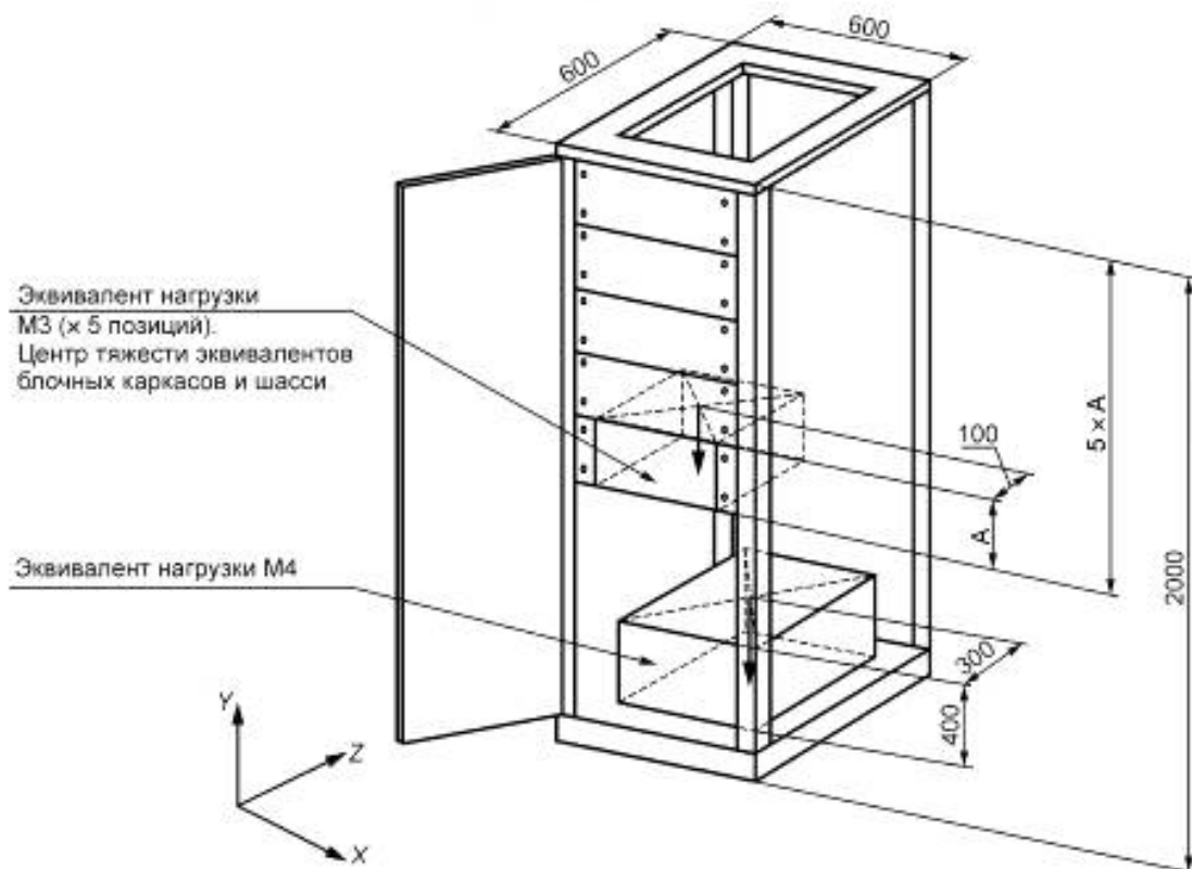
Рисунок 8 — Условия сборки и распределение нагрузки для испытания шкафов на ударное воздействие и вибрацию
