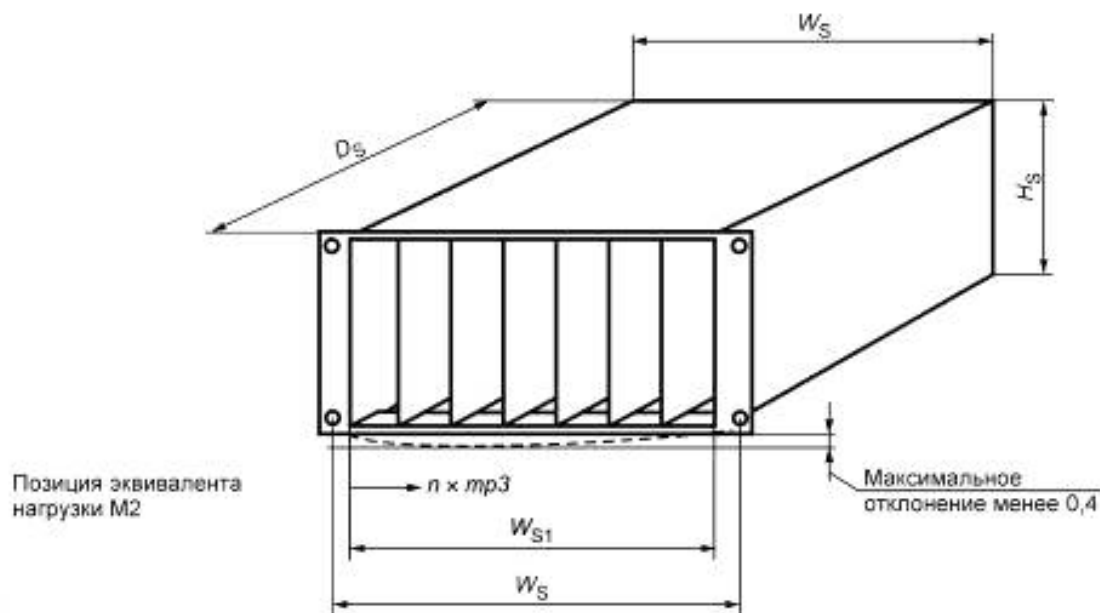
Рисунок 6 — Испытание на статическую нагрузку, распределение мест расположения эквивалентов нагрузки
