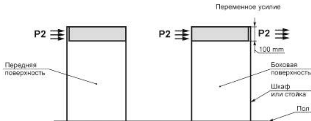
Рисунок 2 — Испытание шкафов и стоек на жесткость
