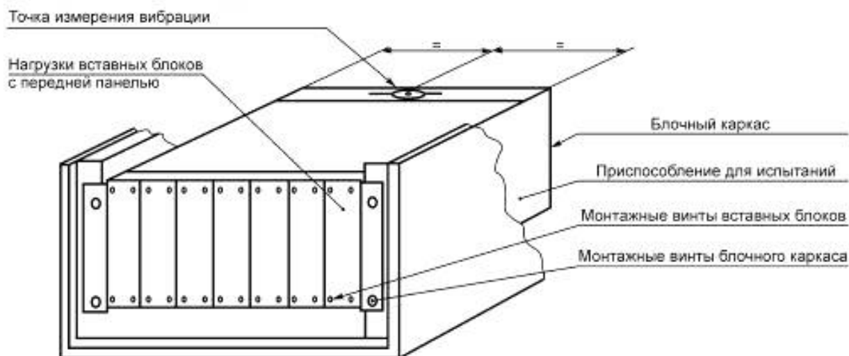
Рисунок 9 — Условия установки блочных каркасов для испытаний на ударное воздействие и вибрацию
