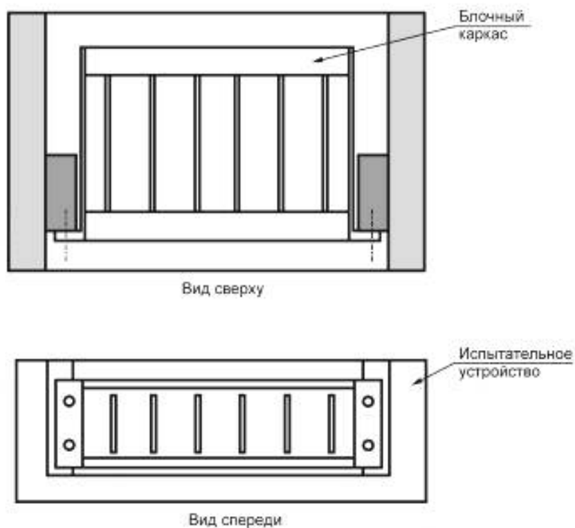
Рисунок 3 — Условия сборки для испытаний на статическую нагрузку для блочных каркасов
