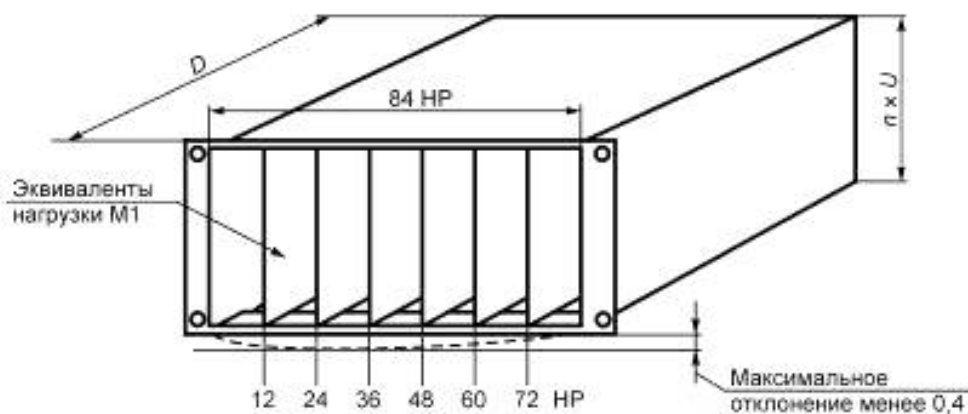
Рисунок 4 — Испытание при статической нагрузке, и места расположения эквивалентов нагрузки
