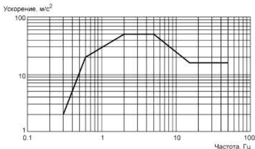
Рисунок 3 — ТСО для тестового сигнала (коэффициент демпфирования 2 %)
