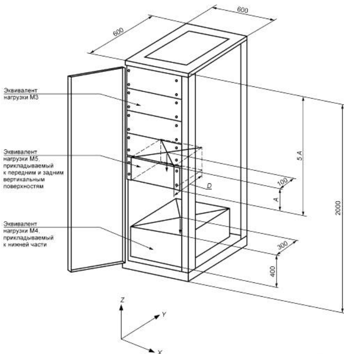
Рисунок 1 — Конфигурация шкафов и стоек для схемы испытания
