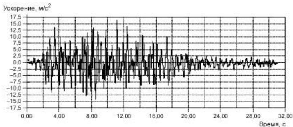
Рисунок 4 — Временная диаграмма тестового сигнала
