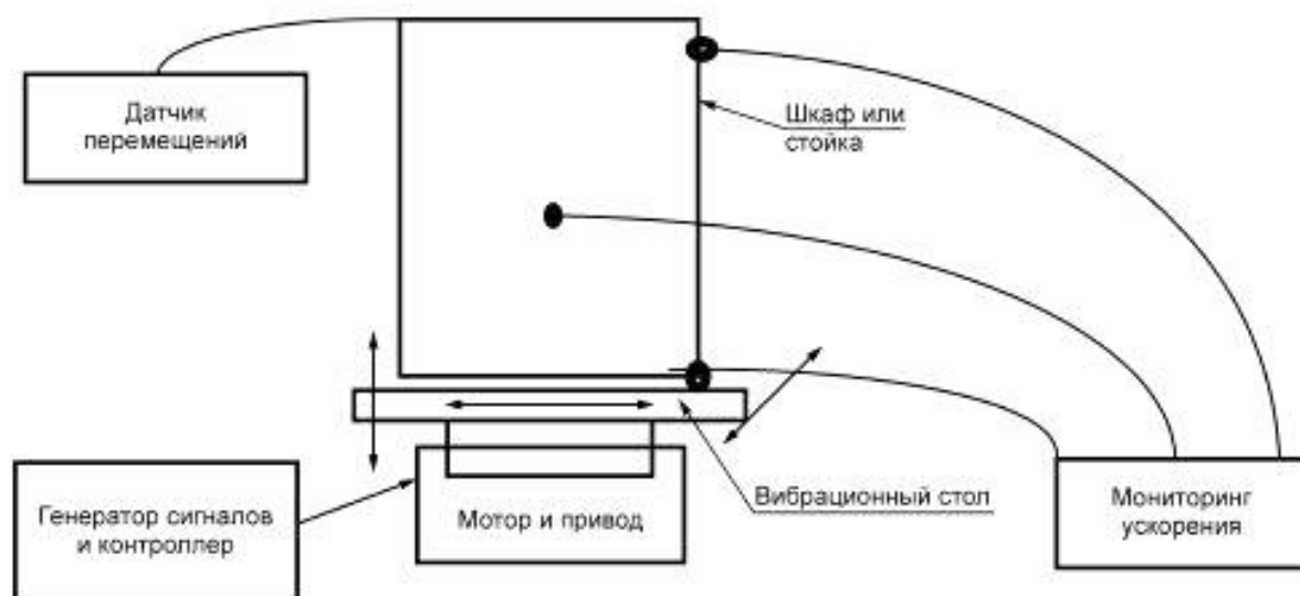
Рисунок 2 — Структурная схема испытания
