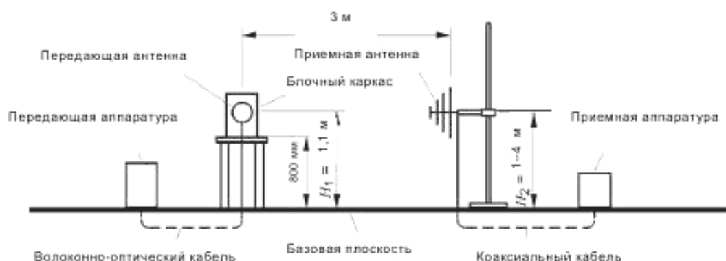
Рисунок 5 – Установка для измерения рассеяния силы сигнала поля E_2 (блочный каркас)
