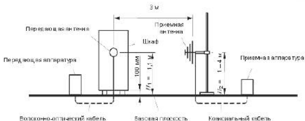
Рисунок 3 – Установка для измерения силы сигнала эталонного поля E_1
