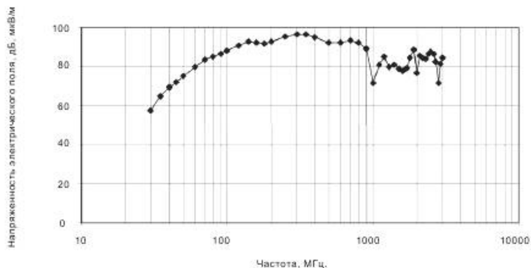
Рисунок А.3 а – Результаты измерений
