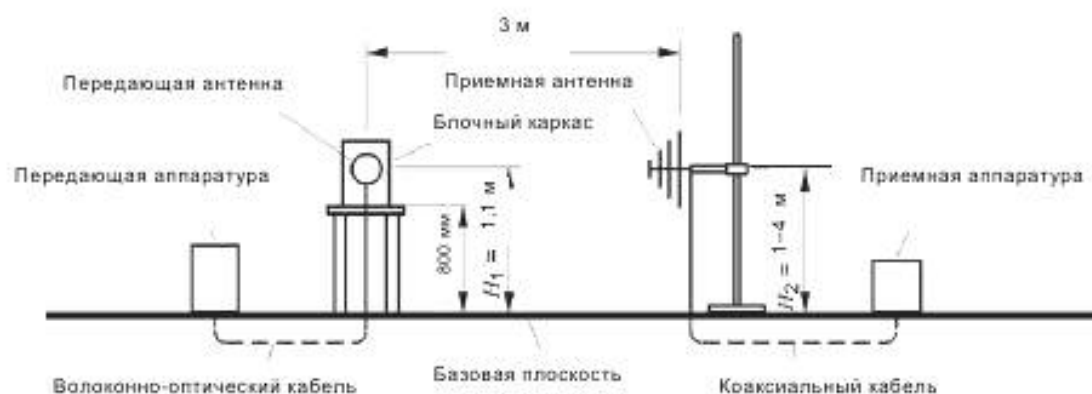
Рисунок 5 – Установка для измерения рассеяния силы сигнала поля E_2 (блочный каркас) 3.5.3 Полубеззховые или полностью беззховые камеры
