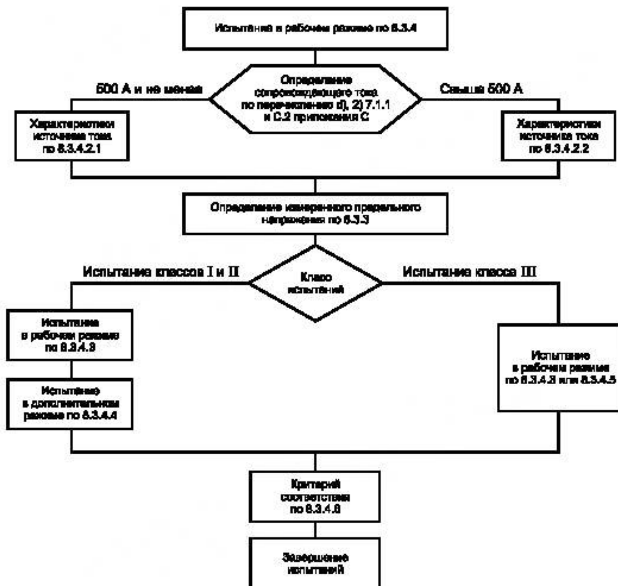
Рисунок 6 — Схема испытания в рабочем режиме
