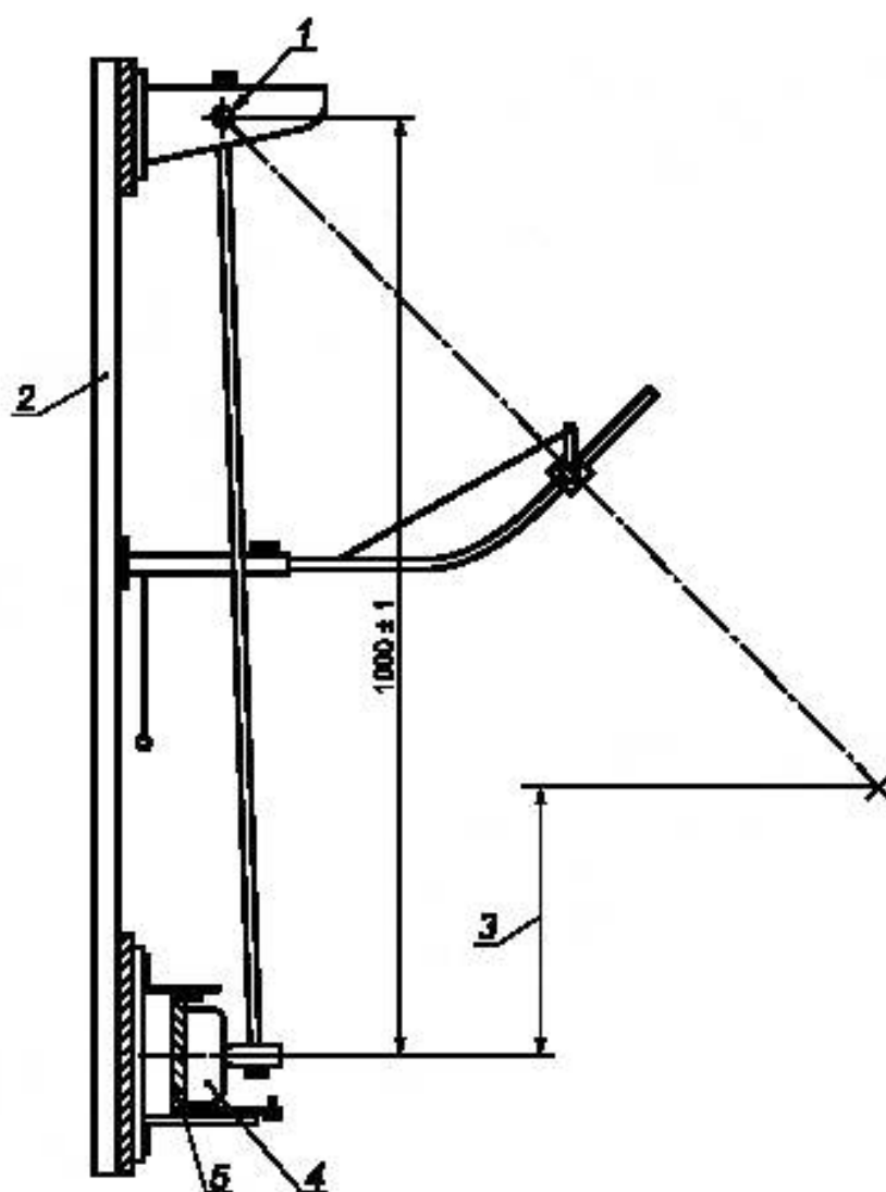
1 — маятник; 2 — рама; 3 — высота падения; 4 — образец; 5 — монтажный хрепез
