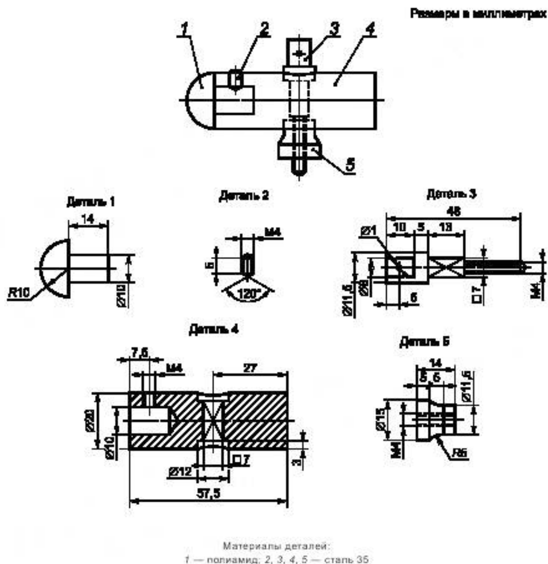
Рисунок 19 — Ударный элемент маятникового молотка для нанесения удара
