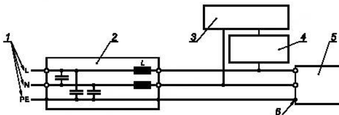
Рисунок 2 — Пример развязывающего фильтра для однофазной сети
