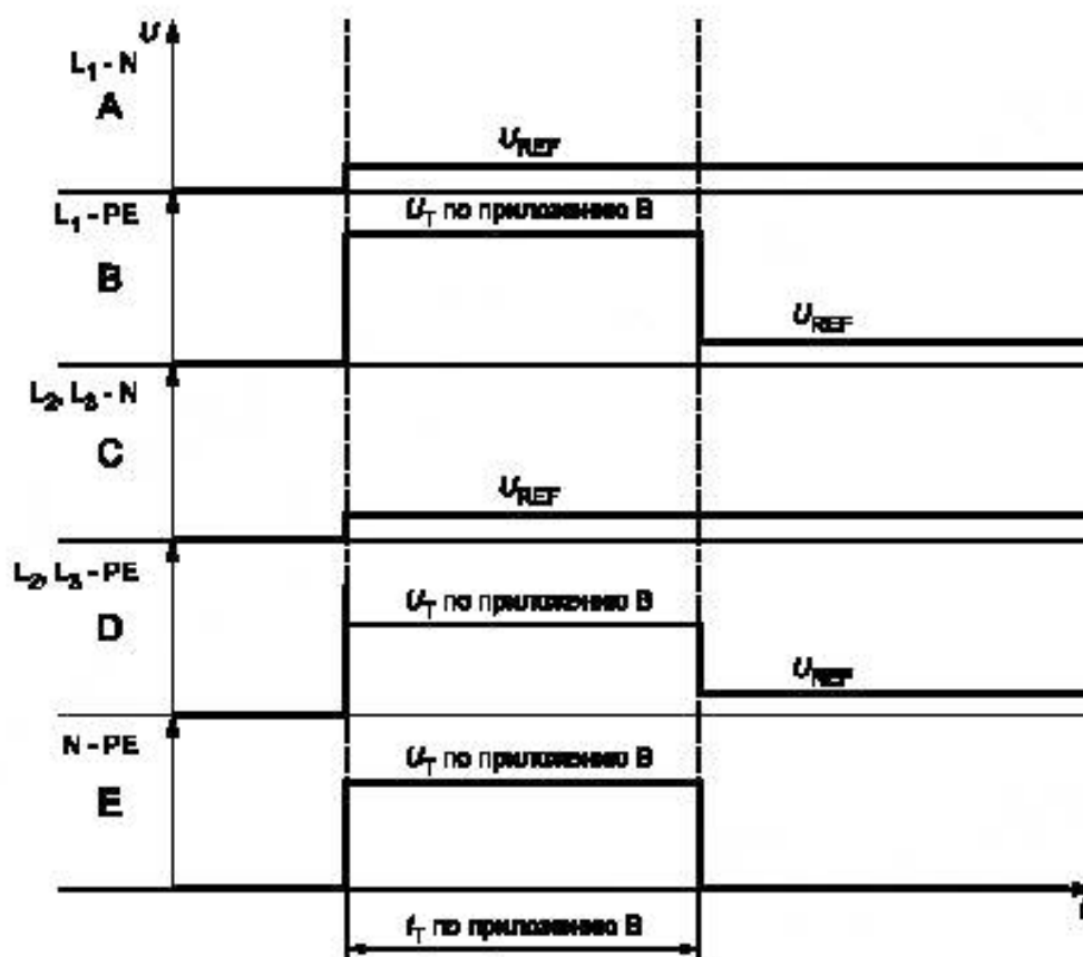
Рисунок 17 — Схема по времени для испытания УЗИП в условиях ВПН, вызванного повреждением в системе высокого (среднего) напряжения, с использованием схемы цепи по рисунку 16
