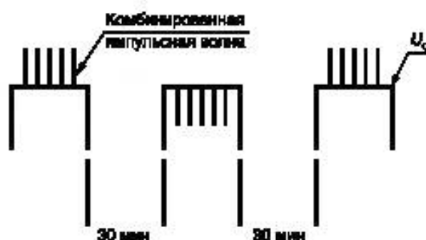
Рисунок 10 — Схема по времени испытаний класса III в рабочем режиме
