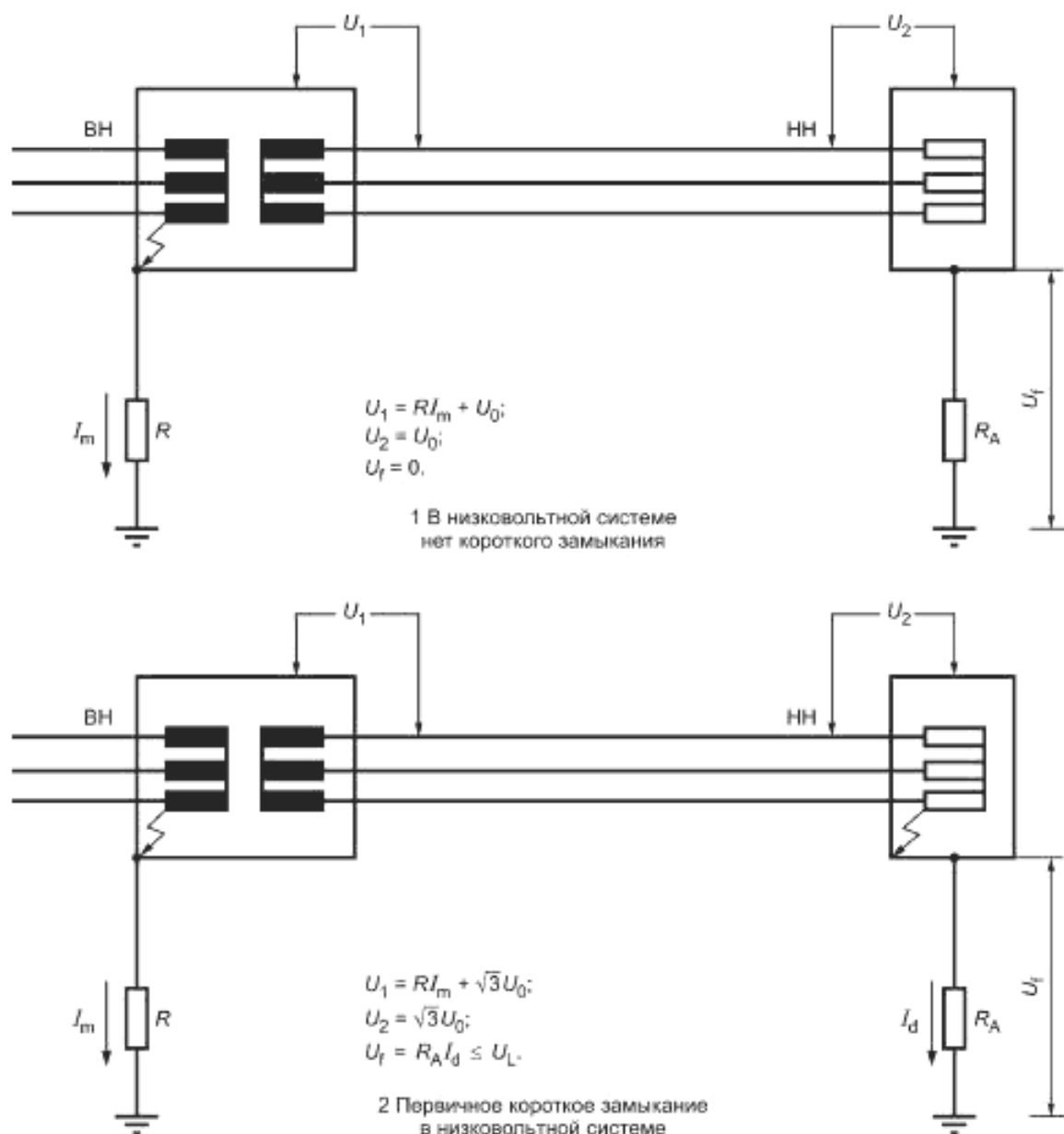
Рисунок Е.7 — Система IT, пример с2
