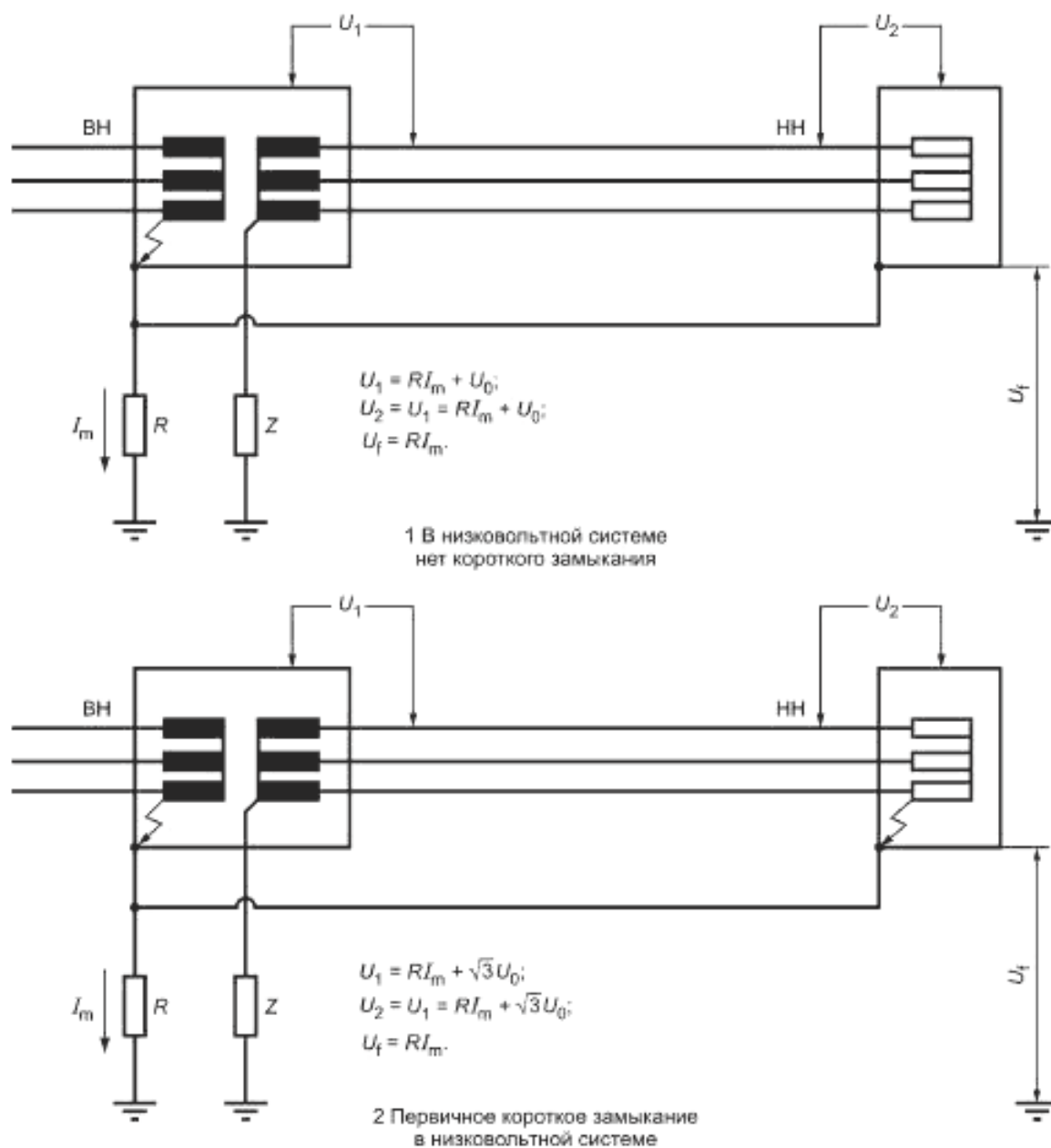
Рисунок Е.9 — Система IT, пример в1
