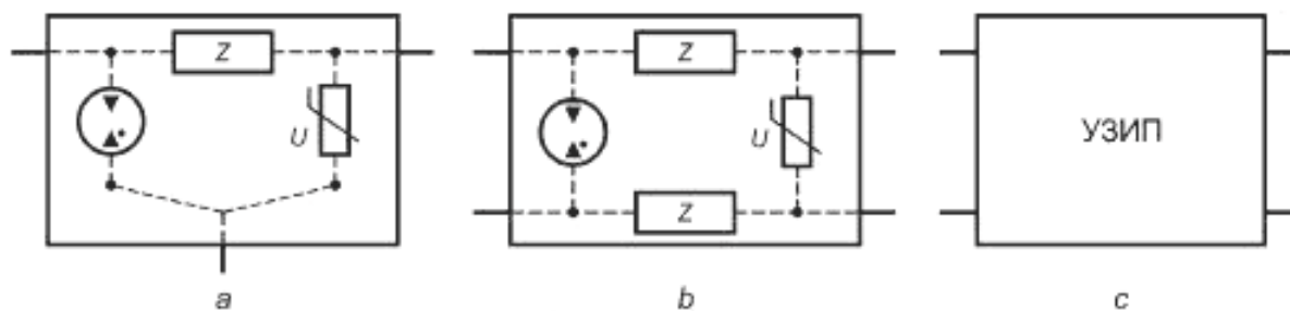
a — двухпроводное УЗИП с тремя выводами; b — двухпроводное УЗИП с четырьмя выводами; c — общий символ обозначения двухпроводного УЗИП; Z — полное сопротивление, включенное последовательно между вводными и выводными зажимами
