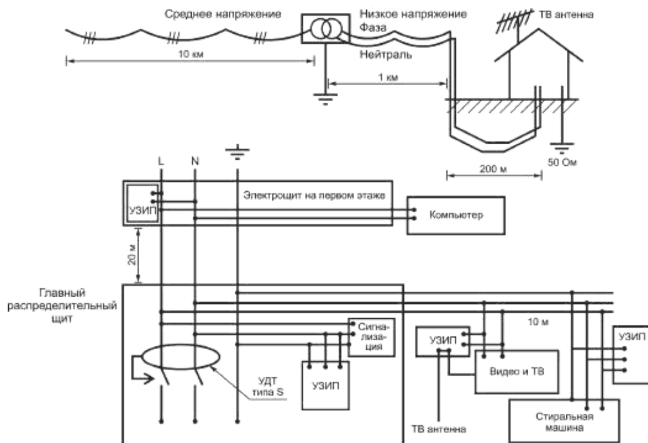
Рисунок G.1 — Бытовая электроустановка
