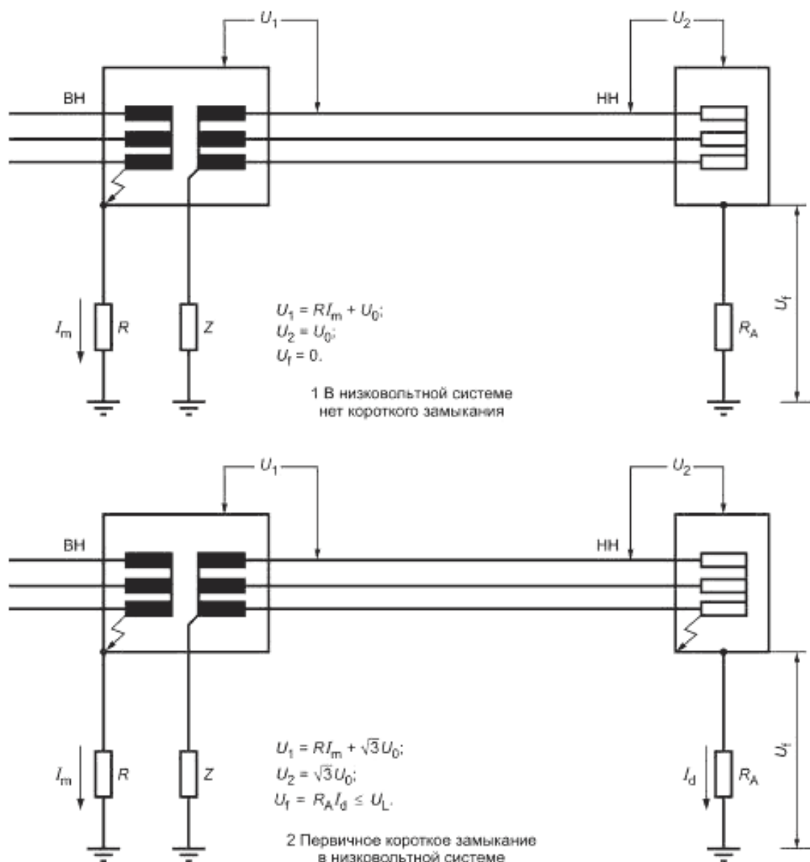
Рисунок Е.6 — Система IT, пример с1
