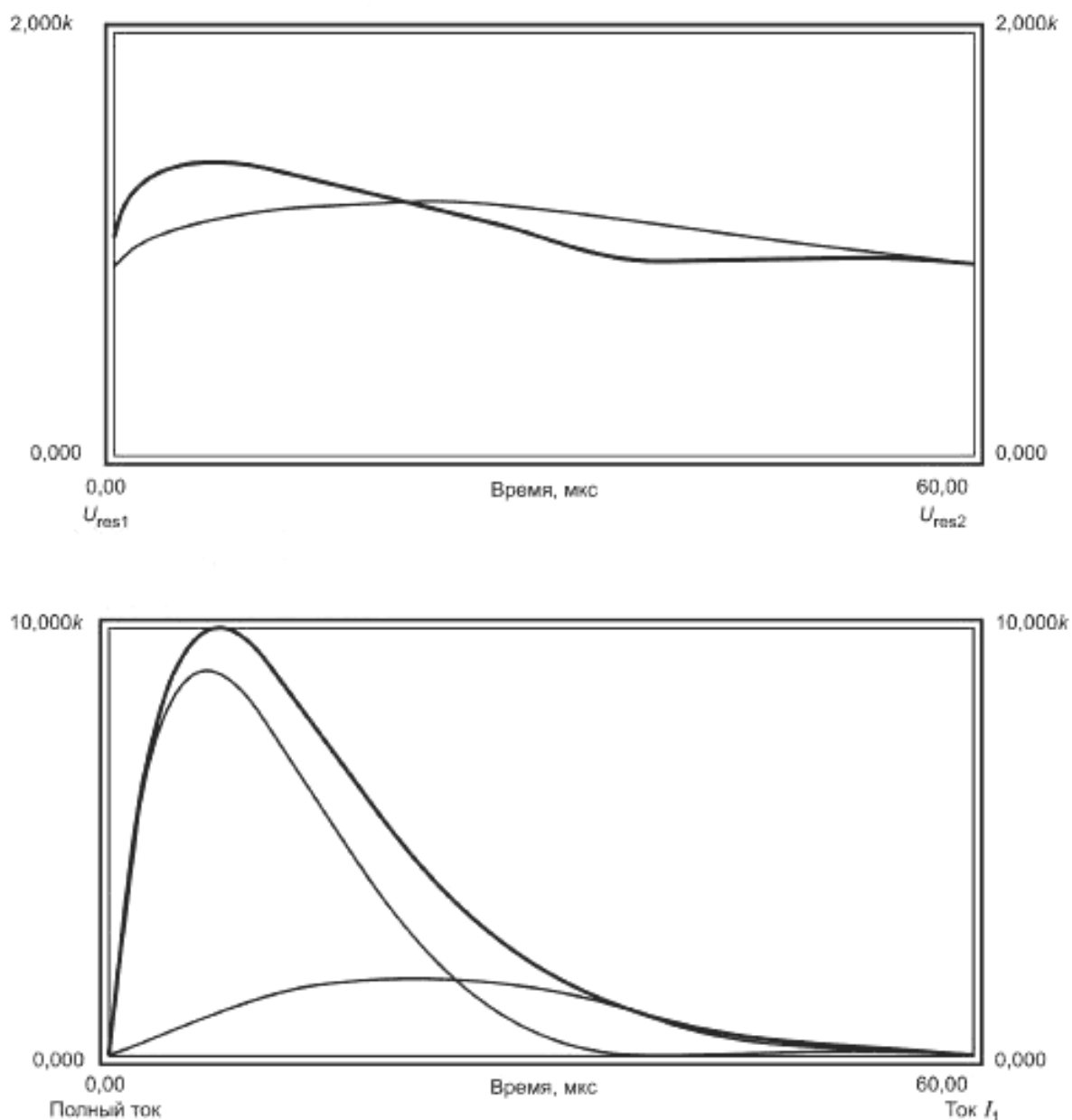
Рисунок К.12 — Координация двух цинкооксидных варисторов
