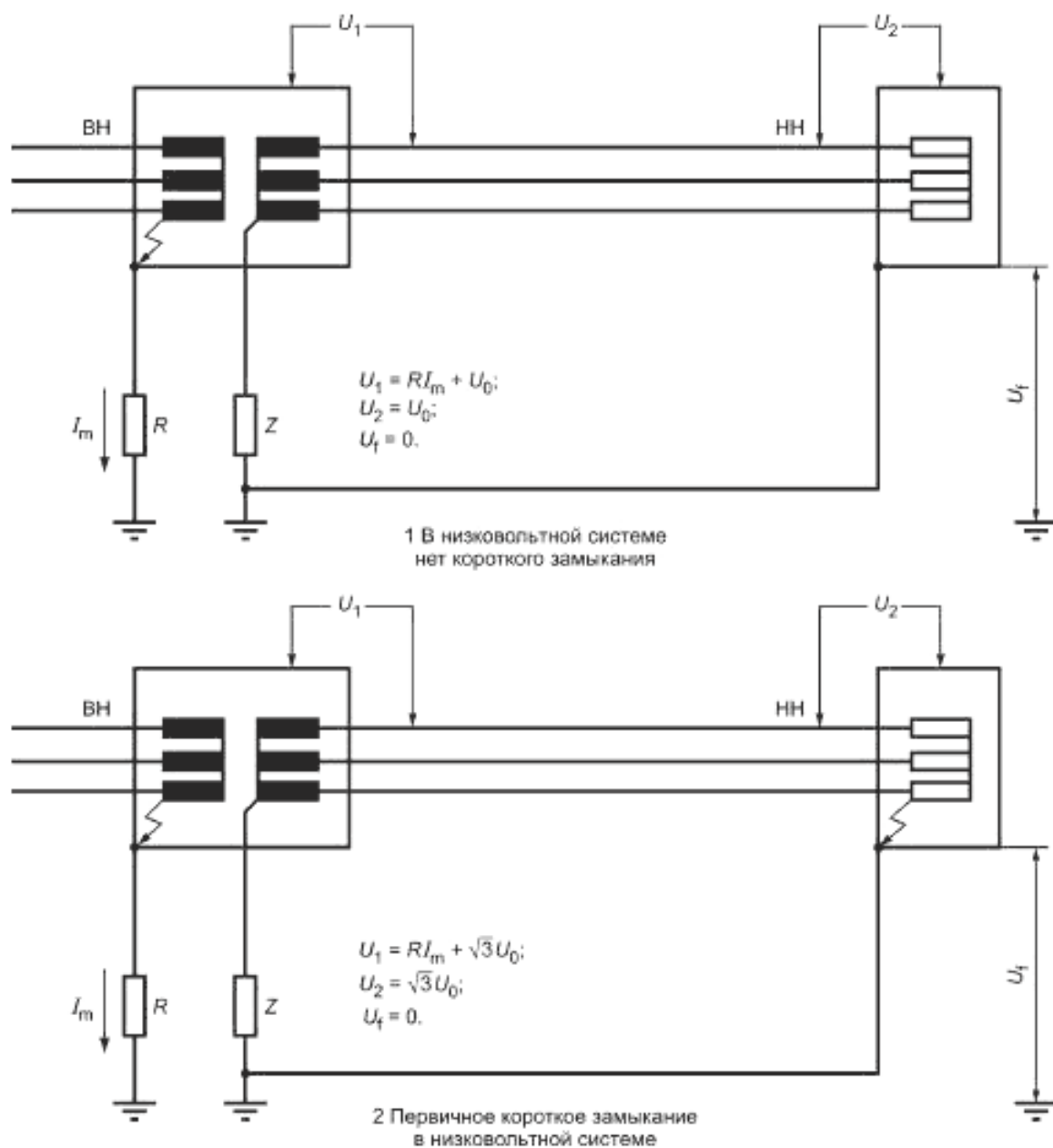
Рисунок Е.8 — Система IT, пример d
