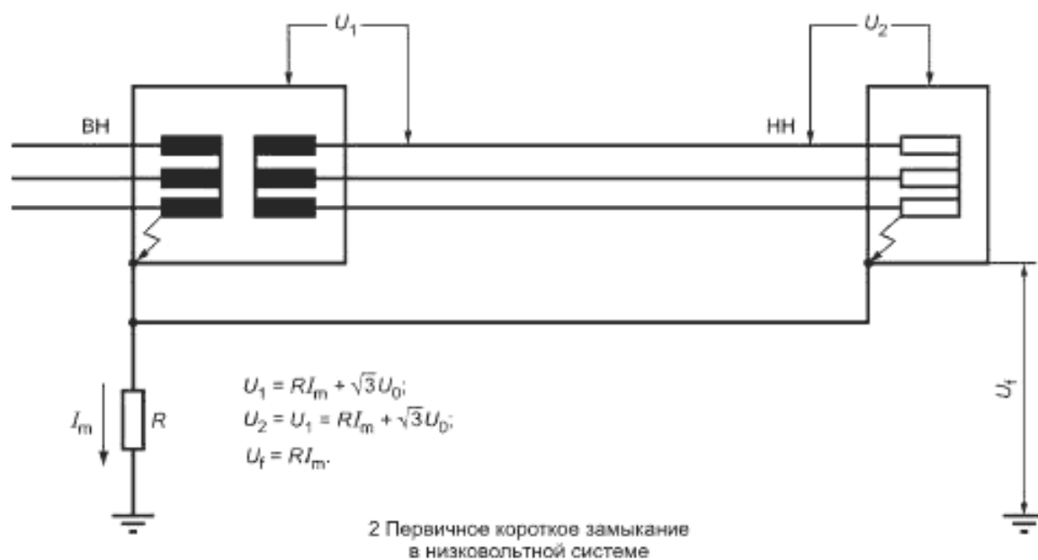
Рисунок Е.10 — Система IT, пример e2
