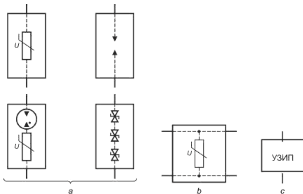
a — однопроводные УЗИП; b — однопроводное УЗИП с раздельными вводными и выводными зажимами; c — общий символ обозначения однопроводного УЗИП
