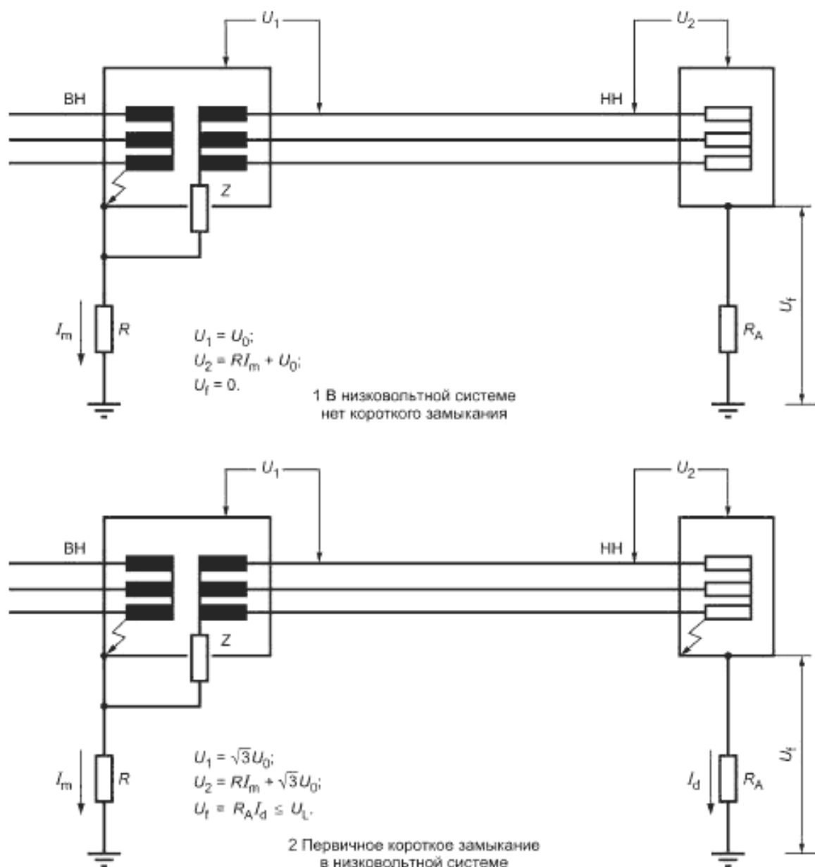
Рисунок Е.5 — Система IT, пример b
