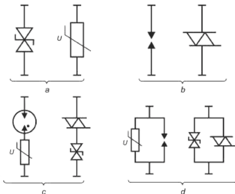
а — элементы, ограничивающие напряжение; б — элементы, коммутирующие напряжение; в — элементы, ограничивающие напряжение, в последовательном соединении с элементами, коммутирующими напряжение; г — элементы, ограничивающие напряжение, в параллельном соединении с элементами, коммутирующими напряжение
