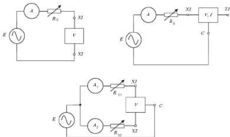
Рисунок 2 – Испытательные цепи для проверки времени восстановления импульсов
