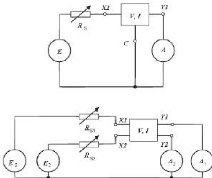
Рисунок 4 – Испытательные цепи для проверки устойчивости к воздействию импульсов и режима повреждения при перенапряжении
