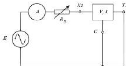
Рисунок 5 – Испытательные цепи для проверки номинального тока, последовательного сопротивления, времени срабатывания, времени возврата тока, максимального напряжения отключения и рабочего режима
