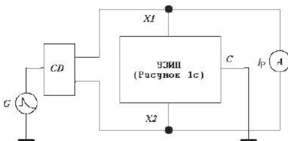
Рисунок E.3 – Определение сквозного тока дифференциального вида
