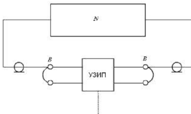
Рисунок 8 – Испытательные цепи для проверки потерь при вводе
