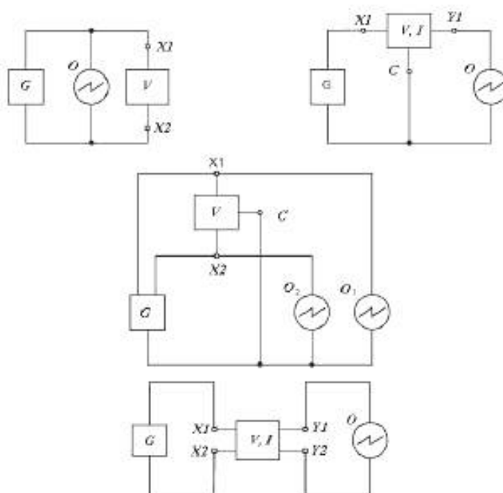
Рисунок 3 – Испытательные цепи для проверки устойчивости к воздействию переменного тока и режима повреждения при перенапряжении
