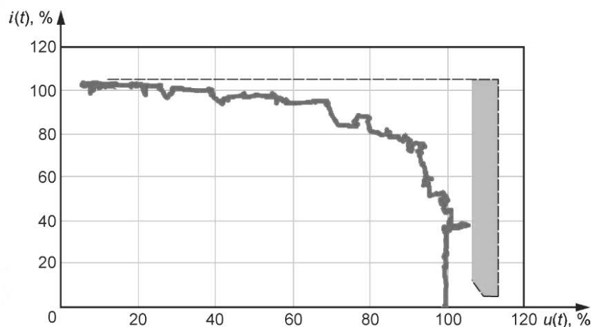
Рисунок В.7 — Характеристика I/U имитатора фотозлектрической батареи, рассчитанная на основании нормализованных значений тока и напряжения, указанных на рисунке В.6
