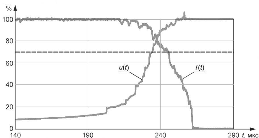
Рисунок В.6 — Нормализованное поведение при отключении во время функционирования плавкого предохранителя, рассчитанного на 0,1I_{кзРВ} , при использовании имитатора фотозлектрической батареи с точкой пересечения i(t) и u(t)
