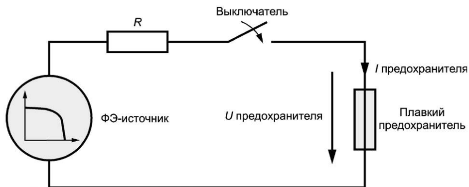
Рисунок В.5 — Испытательная установка с использованием плавкого предохранителя для определения поведения имитатора фотозлектрической батареи в переходном режиме
