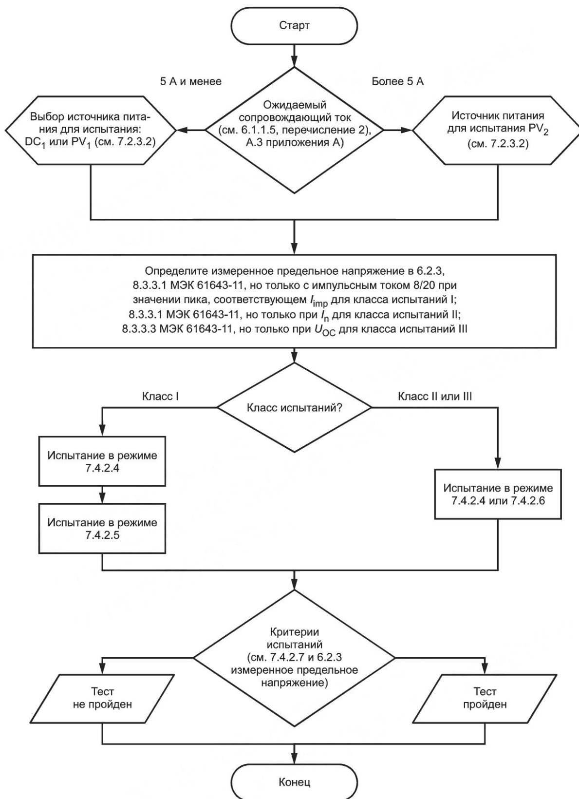
Рисунок 2 — Схема проведения испытания в рабочем режиме
