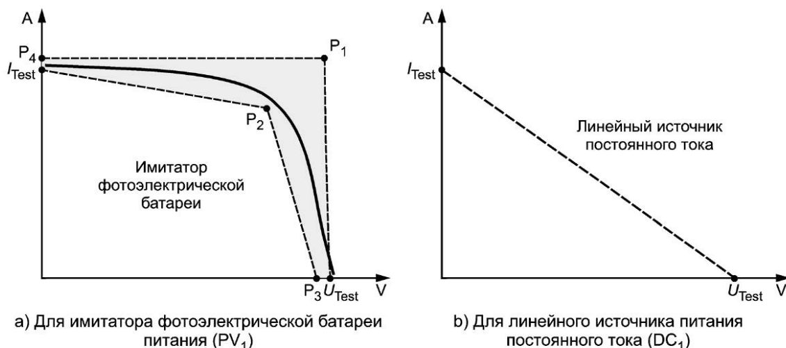
Рисунок 1 — Вольт-амперные характеристики
