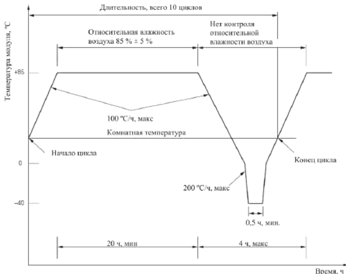
Рисунок 5 — Термоциклирование при высокой влажности
