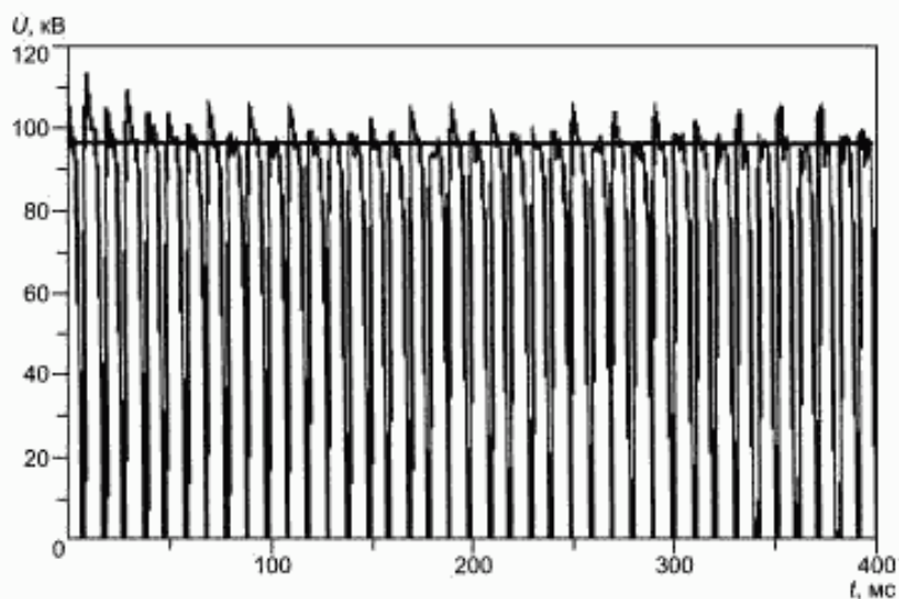
Рисунок В.1 — Пример выходного напряжения для двухпульсного генератора
