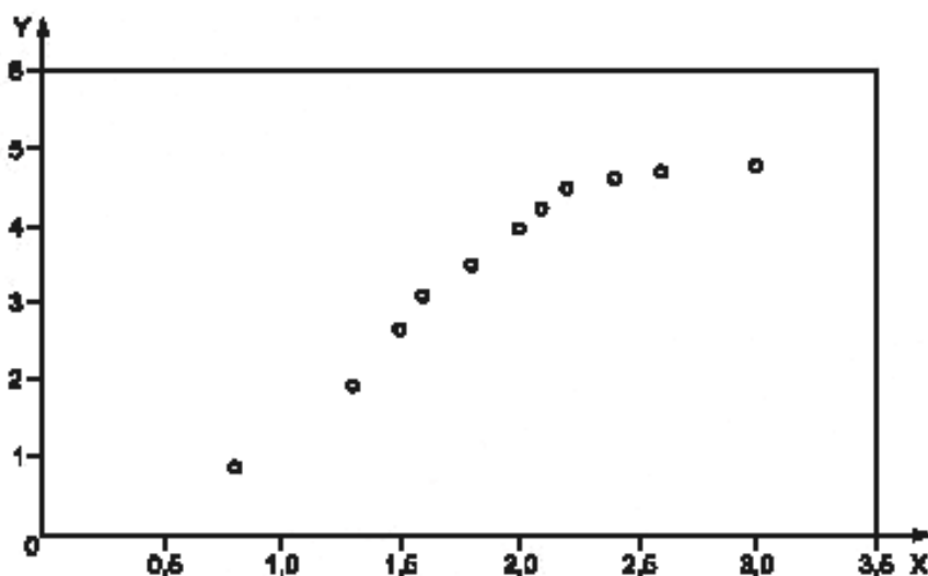
Рисунок 1.2 — Измеренная мощность, прошедшая через апертуры различного диаметра, для лечебной головки с частотой 1 МГц
