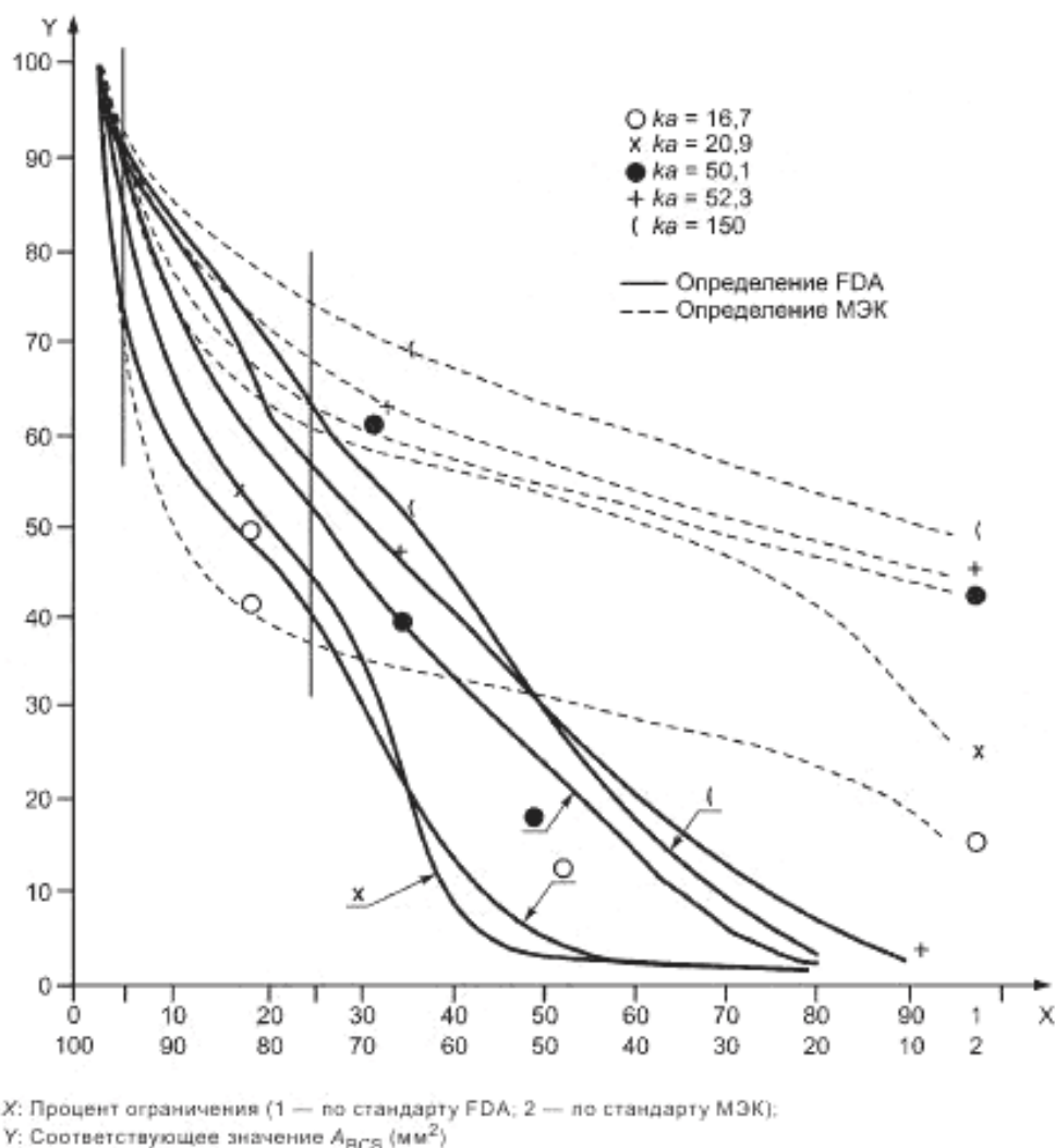
Рисунок D.3 — Нормированные значения площади поперечного сечения пучка при ограничениях FDA и МЭК для 5 преобразователей с различными ka при z = 0,5 см
