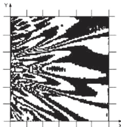
Рисунок D.1 — Линии равных давлений типовой физиотерапевтической лечебной головки малой геометрической площади ( k = 17 )
