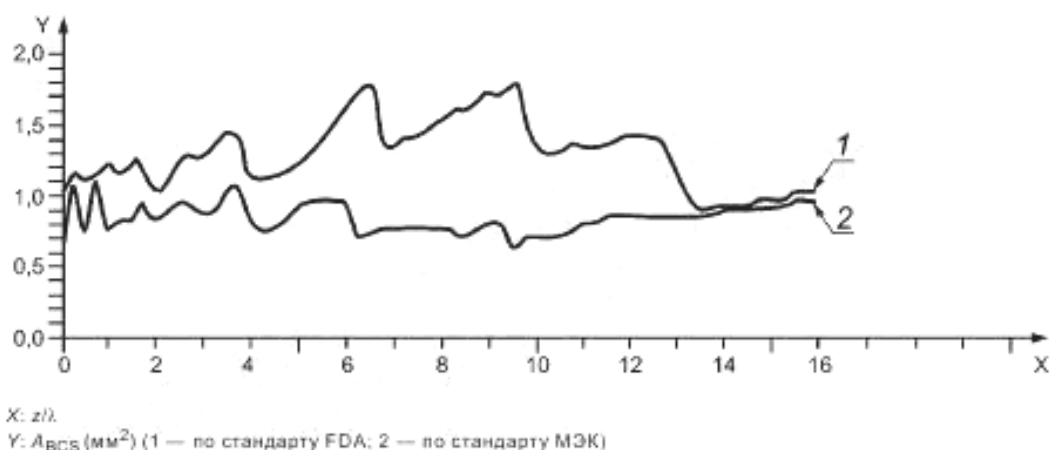
Рисунок D.3 — Нормированные значения площади поперечного сечения пучка при ограничениях FDA и МЭК для 5 преобразователей с различными ka при z = 0,5 см
