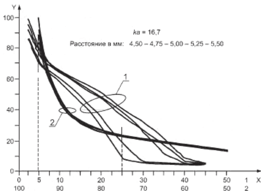
Рисунок D.1 — Линии равных давлений типовой физиотерапевтической лечебной головки малой геометрической площади ( k = 17 )
