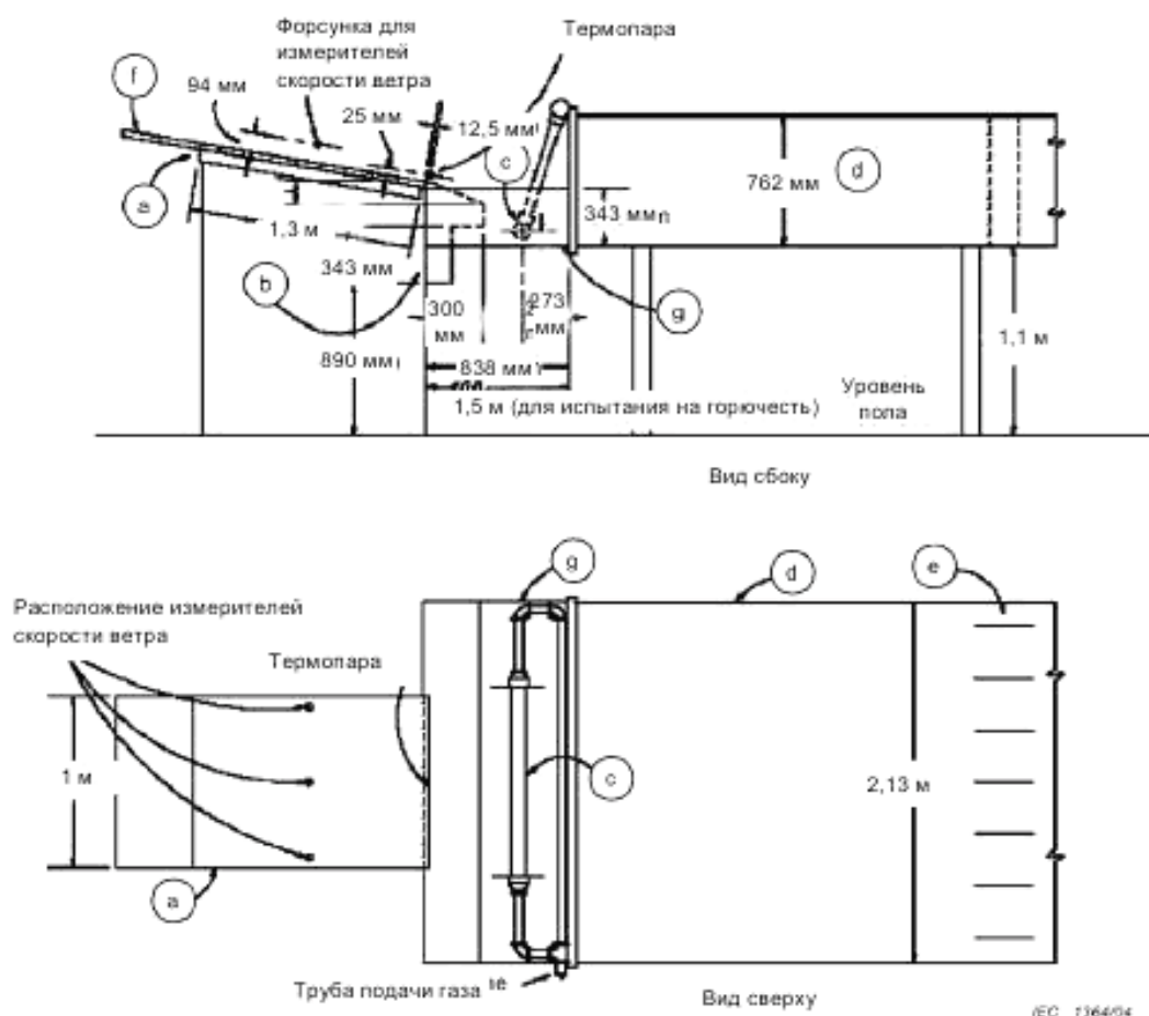
Рисунок А.1 — Конструкция для испытания на огнестойкость
