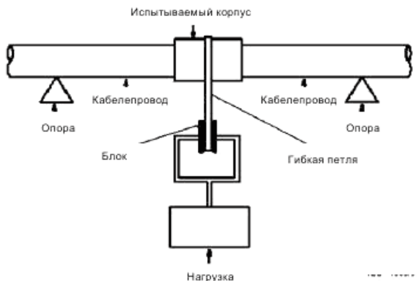
Рисунок 7 — Испытательное приспособление в сборе
