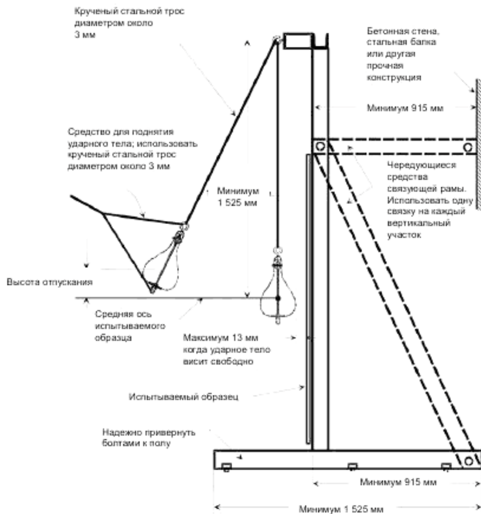
Рисунок 5 — Конструкция № 1 для испытания на удар
