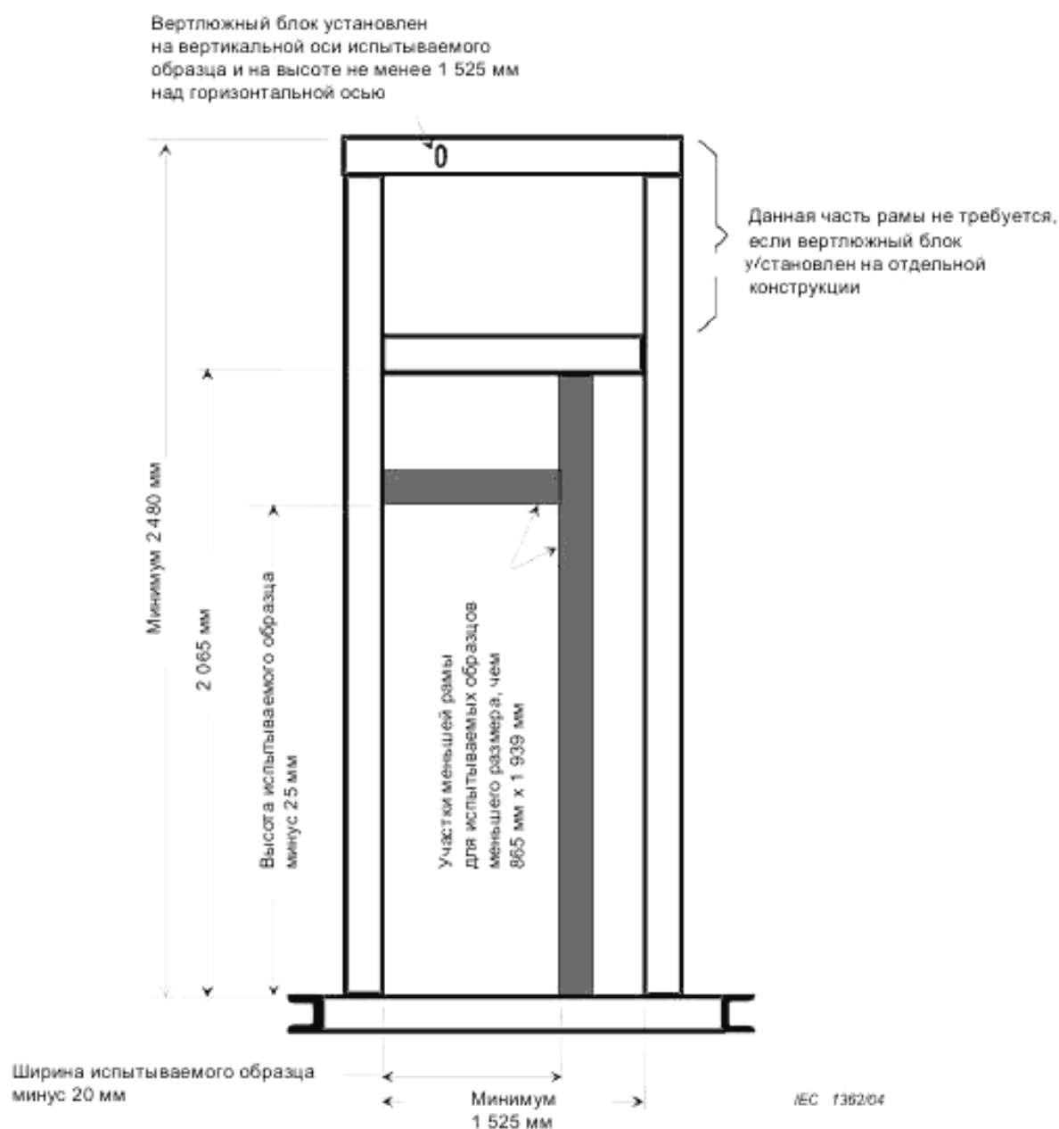
Рисунок 6 — Конструкция № 2 для испытания на удар
