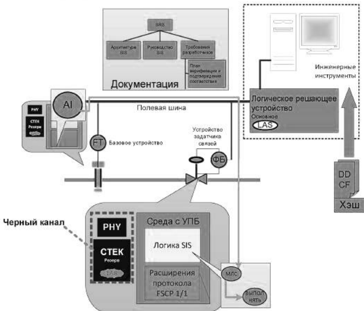
Рисунок 6 — Архитектура (H1) FSCP 1/1
