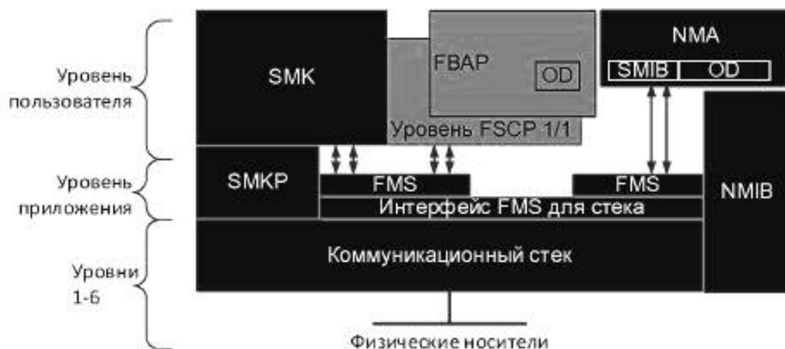
Рисунок 10 — Уровни протокола FSCP 1/1
