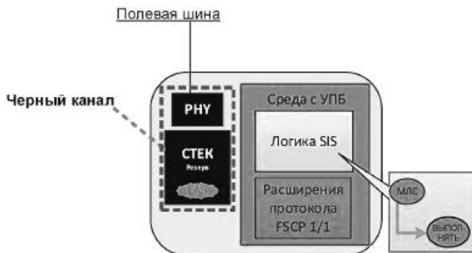
Рисунок 9 — Устройство Н1 с FSCP 1/1
