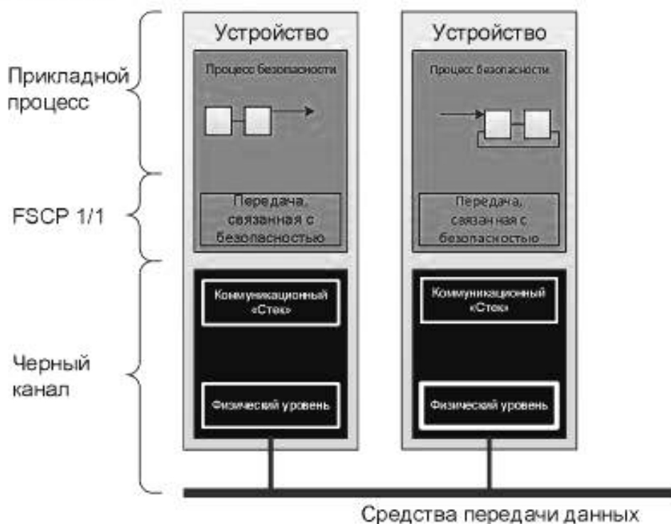
Рисунок 14 — Пример коммуникаций FSCP 1/1
