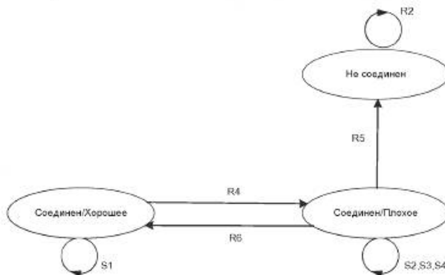
Рисунок 21 — Диаграмма перехода состояний для подписчика FSCP 1/1
