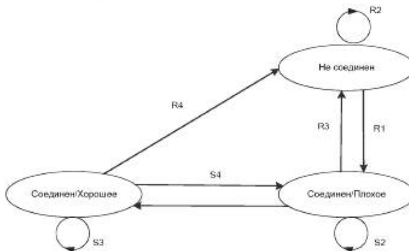
Рисунок 18 — Диаграмма перехода состояний для издателя FSCP 1/1
