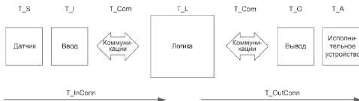
Рисунок 14 —Вычисление наихудшего времени реакции функции безопасности
