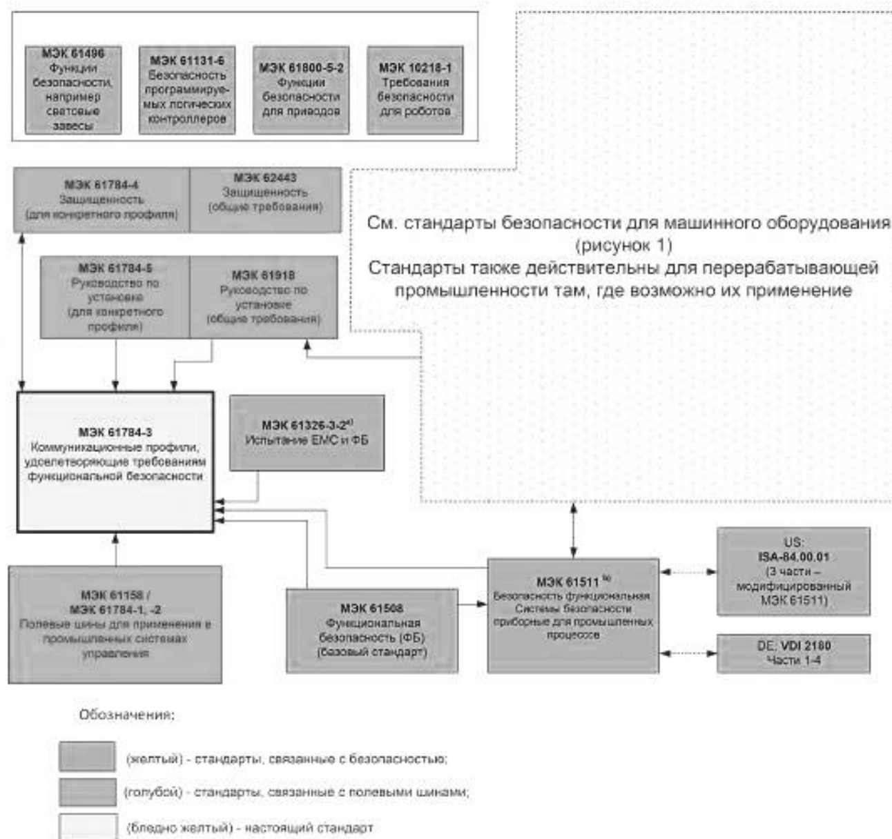
Рисунок 2 — Связь МЭК 61158-3 с другими стандартами (промышленные процессы)
