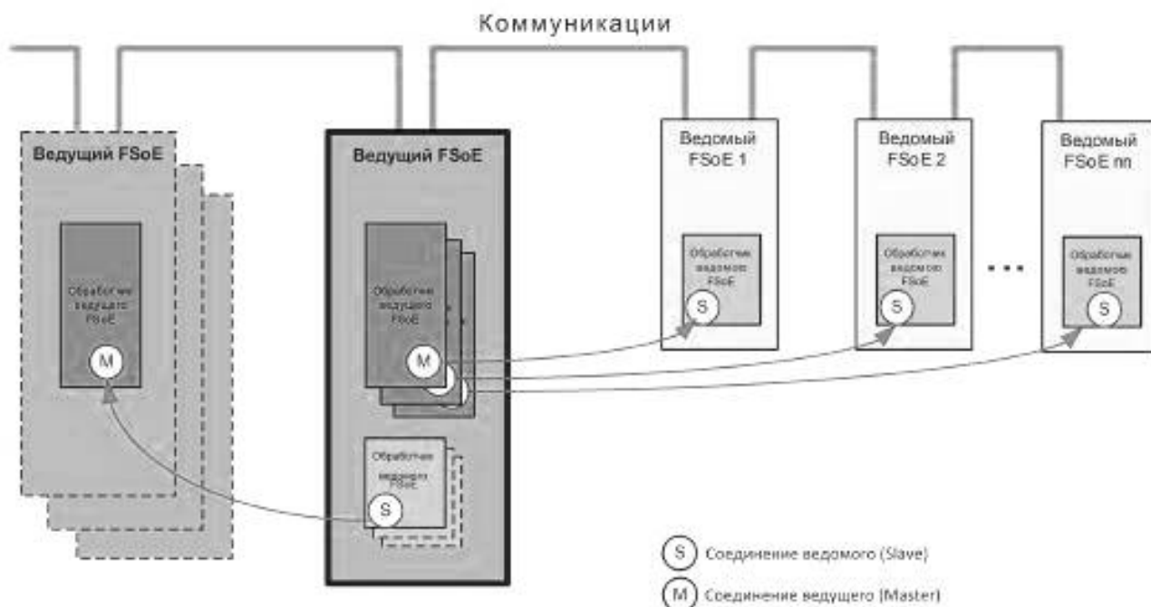
Рисунок 6 — Структура коммуникаций FSCP 12/1
