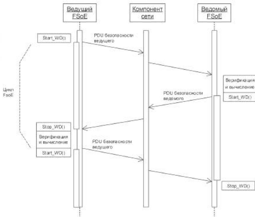
Рисунок 5 — Цикл FSoE
