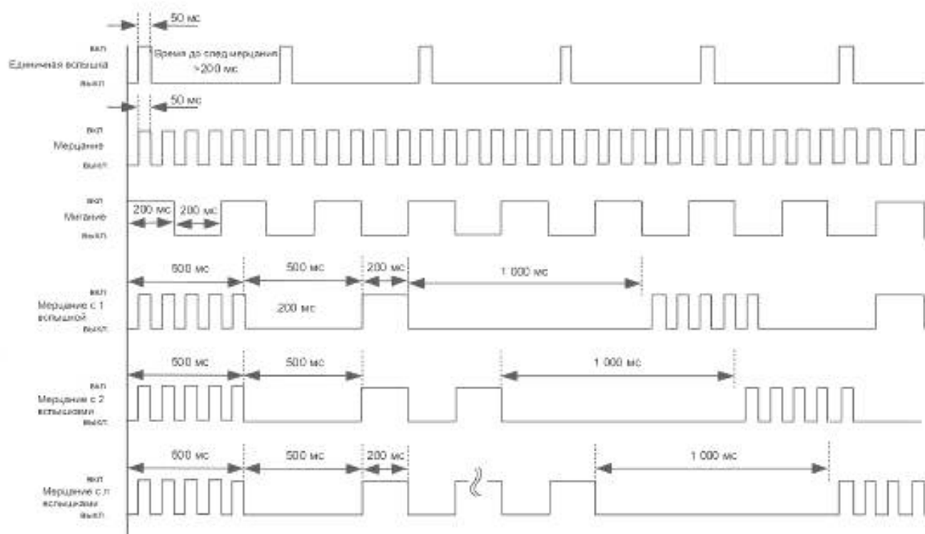
Рисунок 11 — Частота вспышек индикаторов
