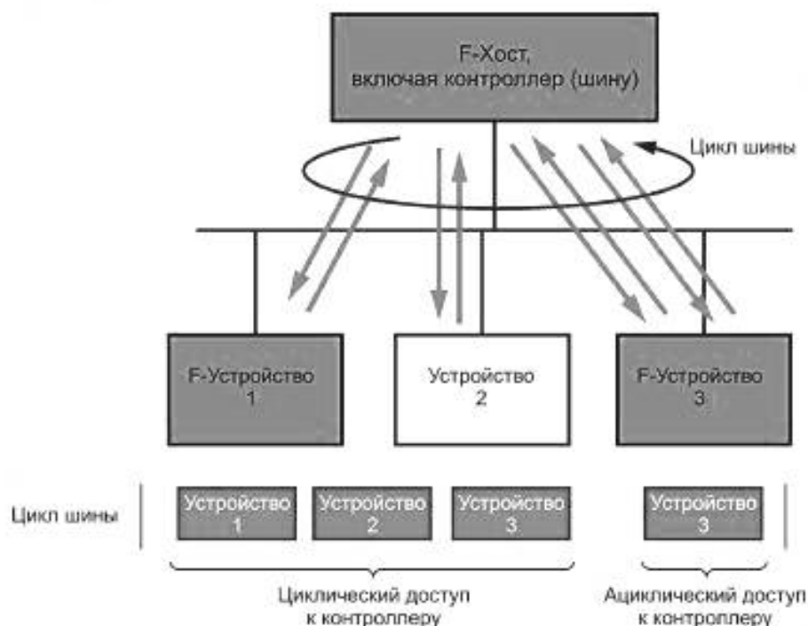
Рисунок 9 — Базовые предварительные условия коммуникации для FSCP 3/1
