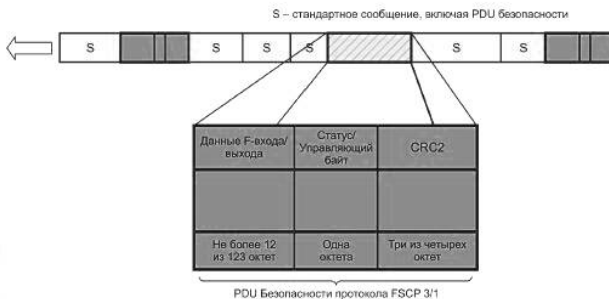
Рисунок 10 — Структура PDU безопасности профиля FSCP 3/1
