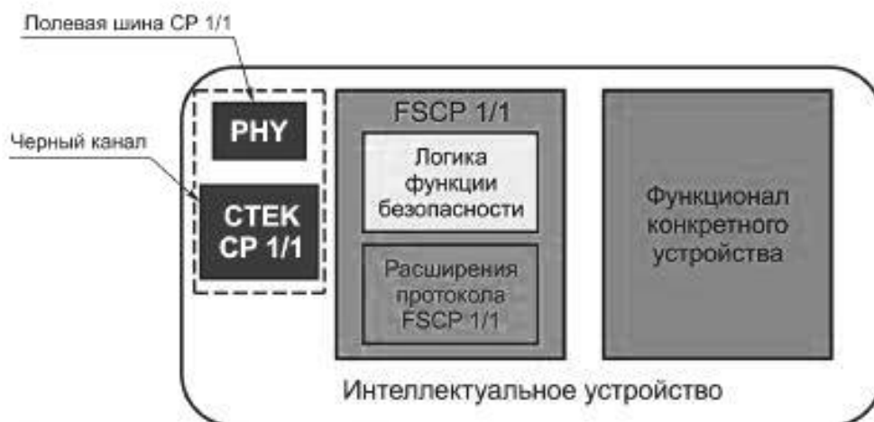
Рисунок 7 — Область применения FSCP 1/1
