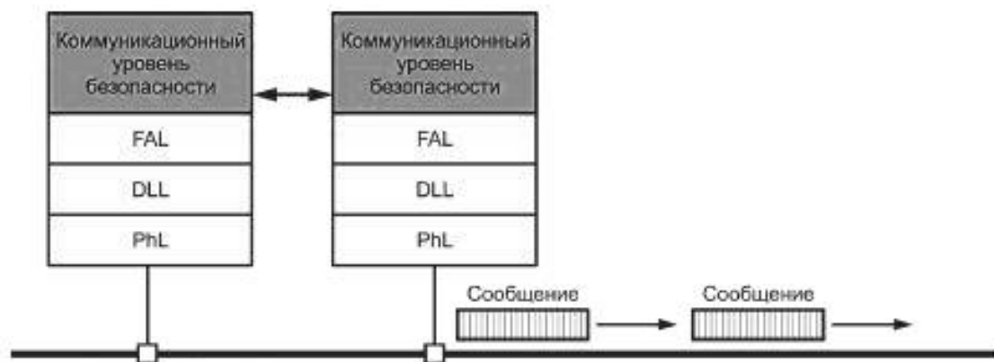
Рисунок A.3 — Модель C
