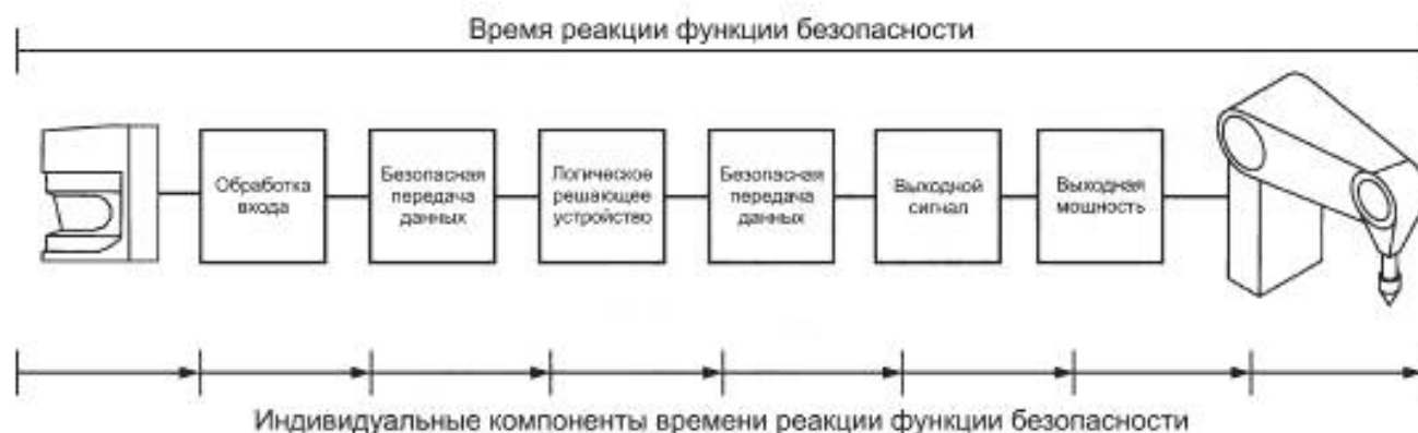
Рисунок 5 — Пример компонентов, составляющих время реакции функции безопасности
