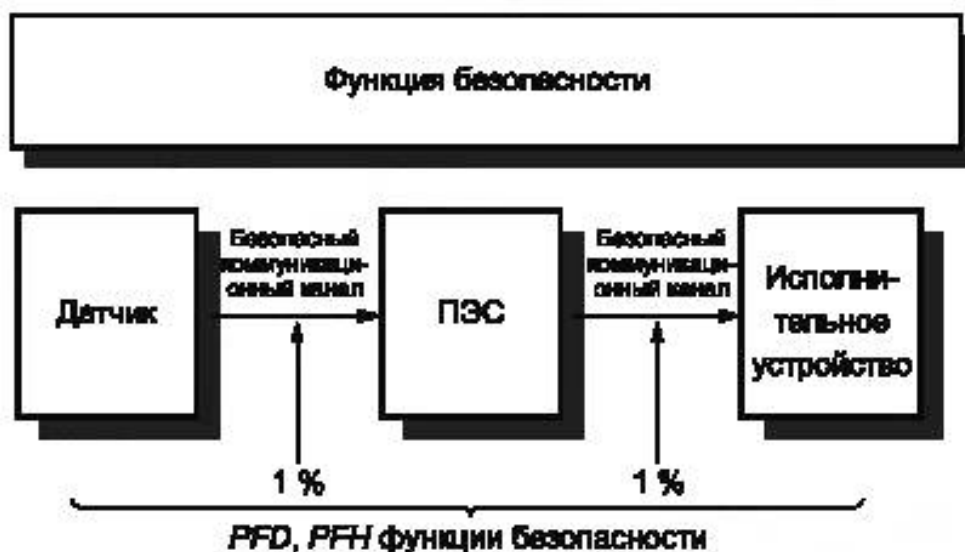
Рисунок 3 — Безопасная коммуникация является частью функции безопасности
