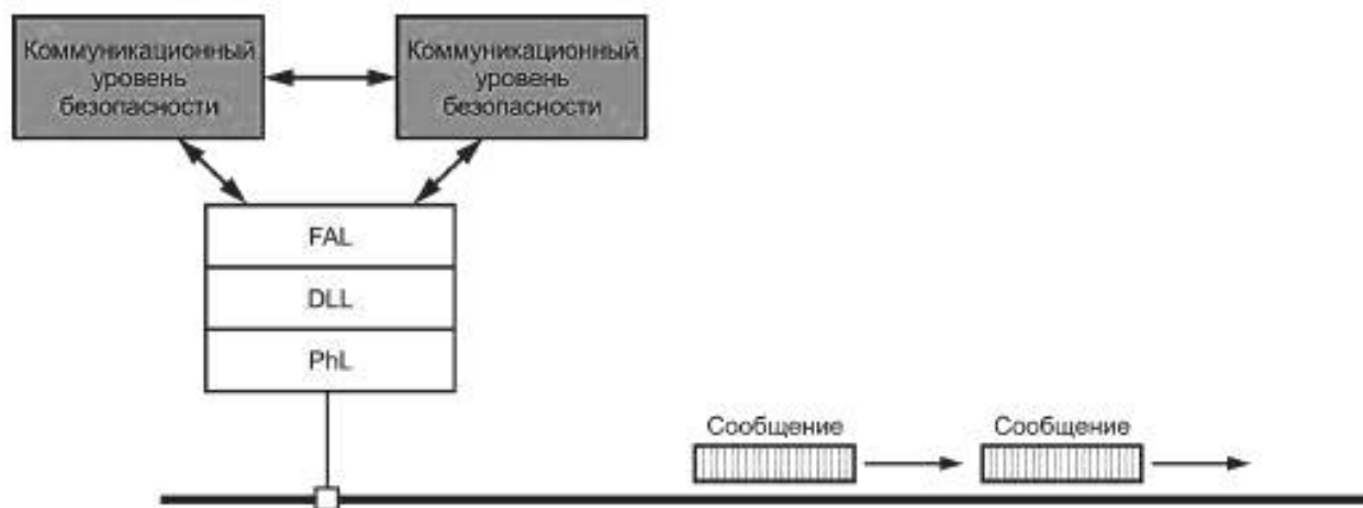
Рисунок А.4 — Модель D
