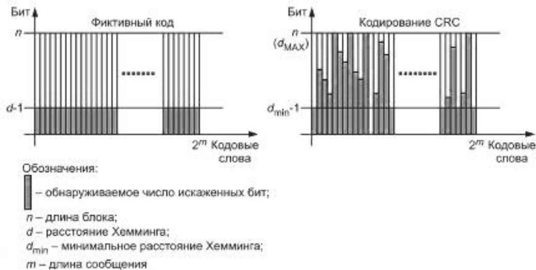
Рисунок В.4 — Коды блоков для обнаружения ошибок
