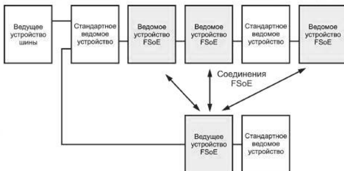
Рисунок 13 — Базовая система FSCP 12/1
