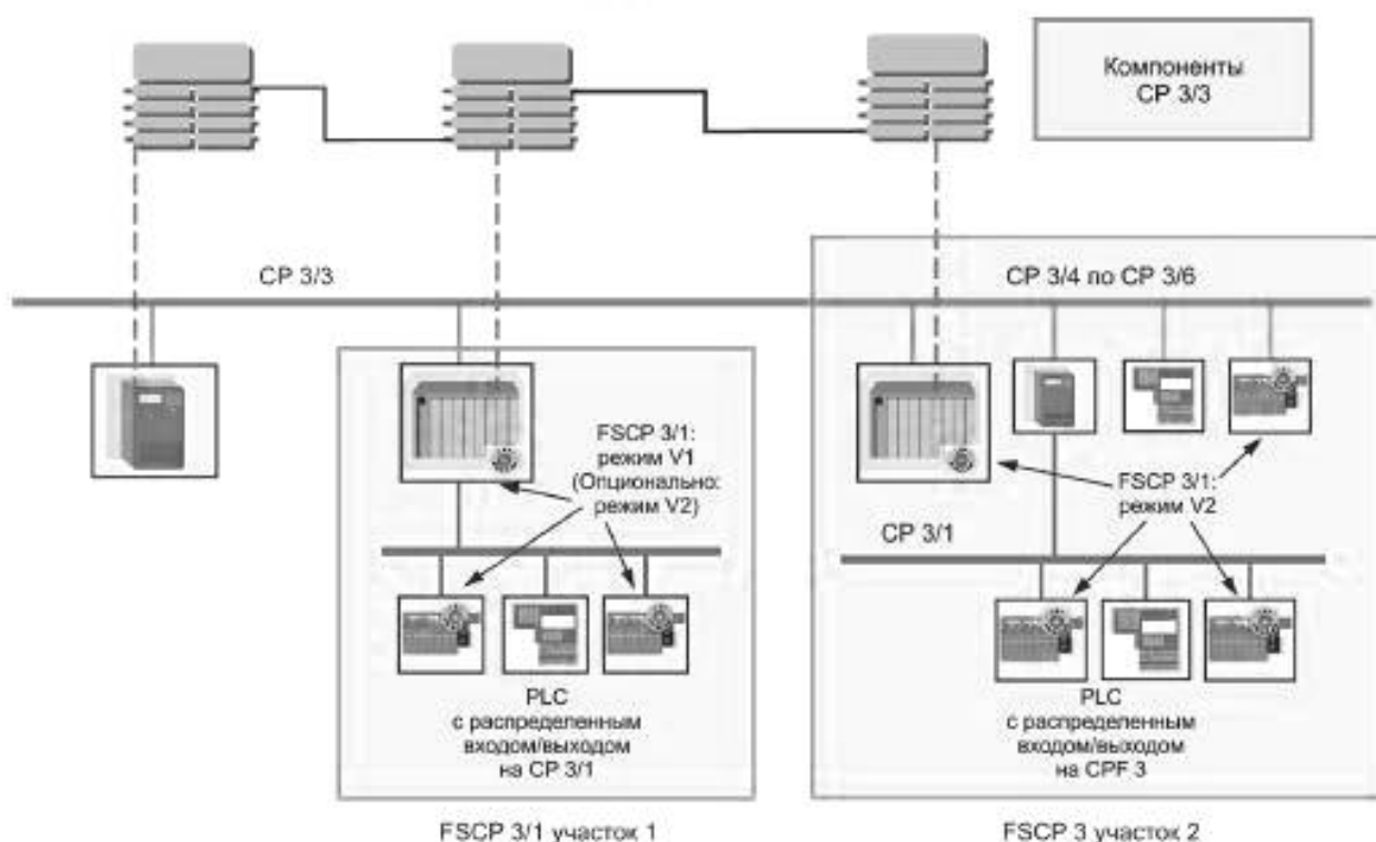
Рисунок 11 — Режимы безопасных коммуникаций
