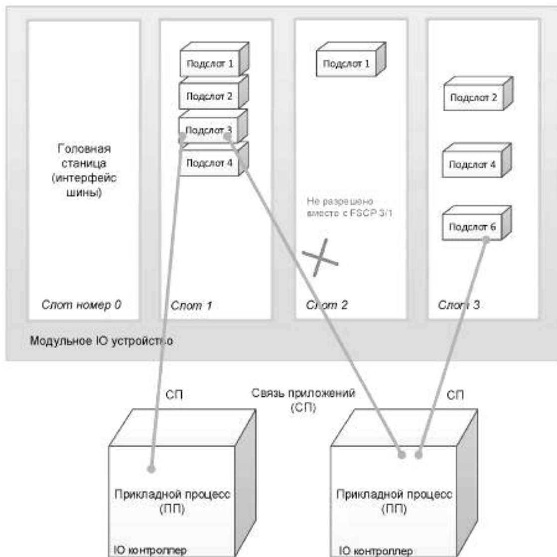
Рисунок 14 — Связи приложений модульного устройства
