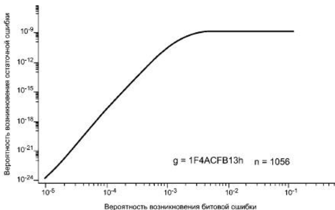
Рисунок 82 — Годность 32-битового полинома для 132 октетов
