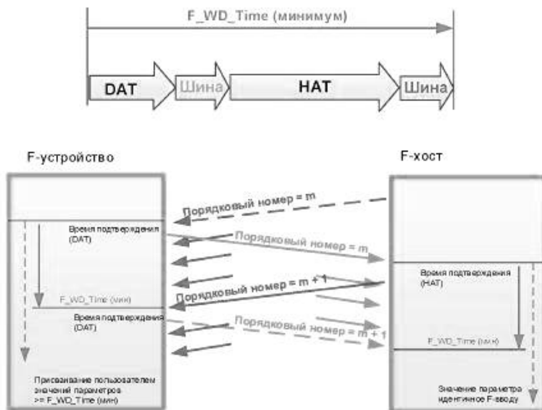
Рисунок 76 — Временные секции, формирующие F WD Time профиля FSCP 3/1
