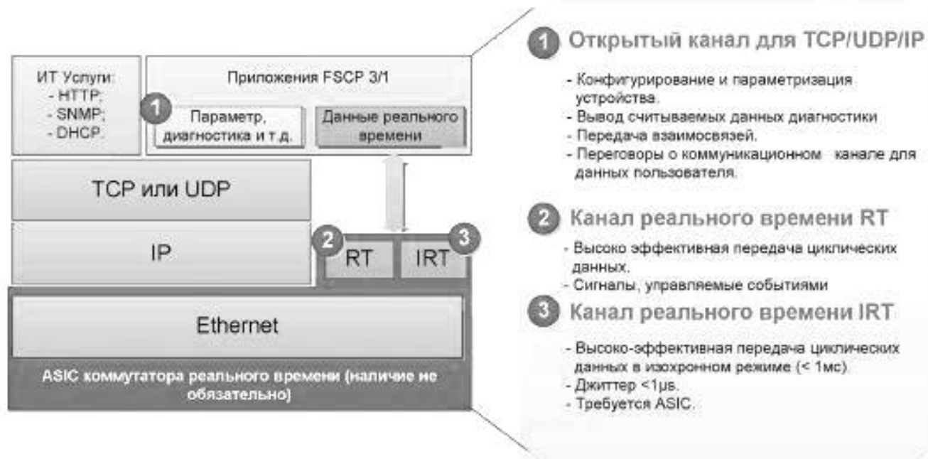
Рисунок 8 — Базовые уровни коммуникаций
