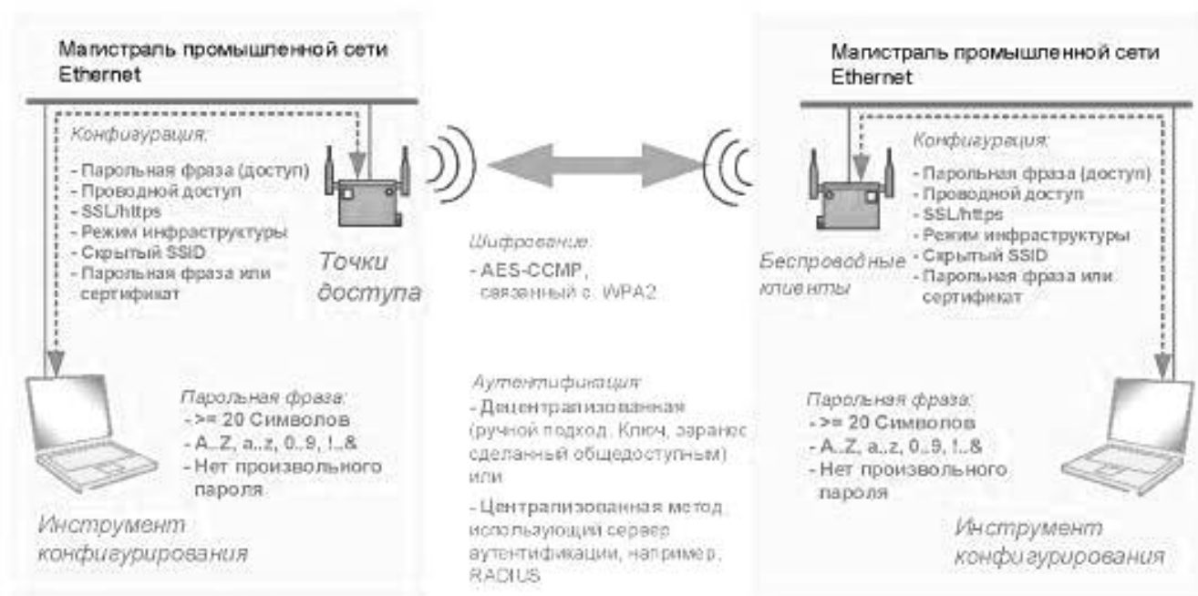
Рисунок 84 — Защита для WLAN сетей
