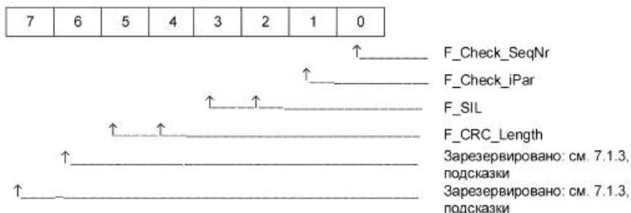
Рисунок 43 — F_Prm_Flag1
