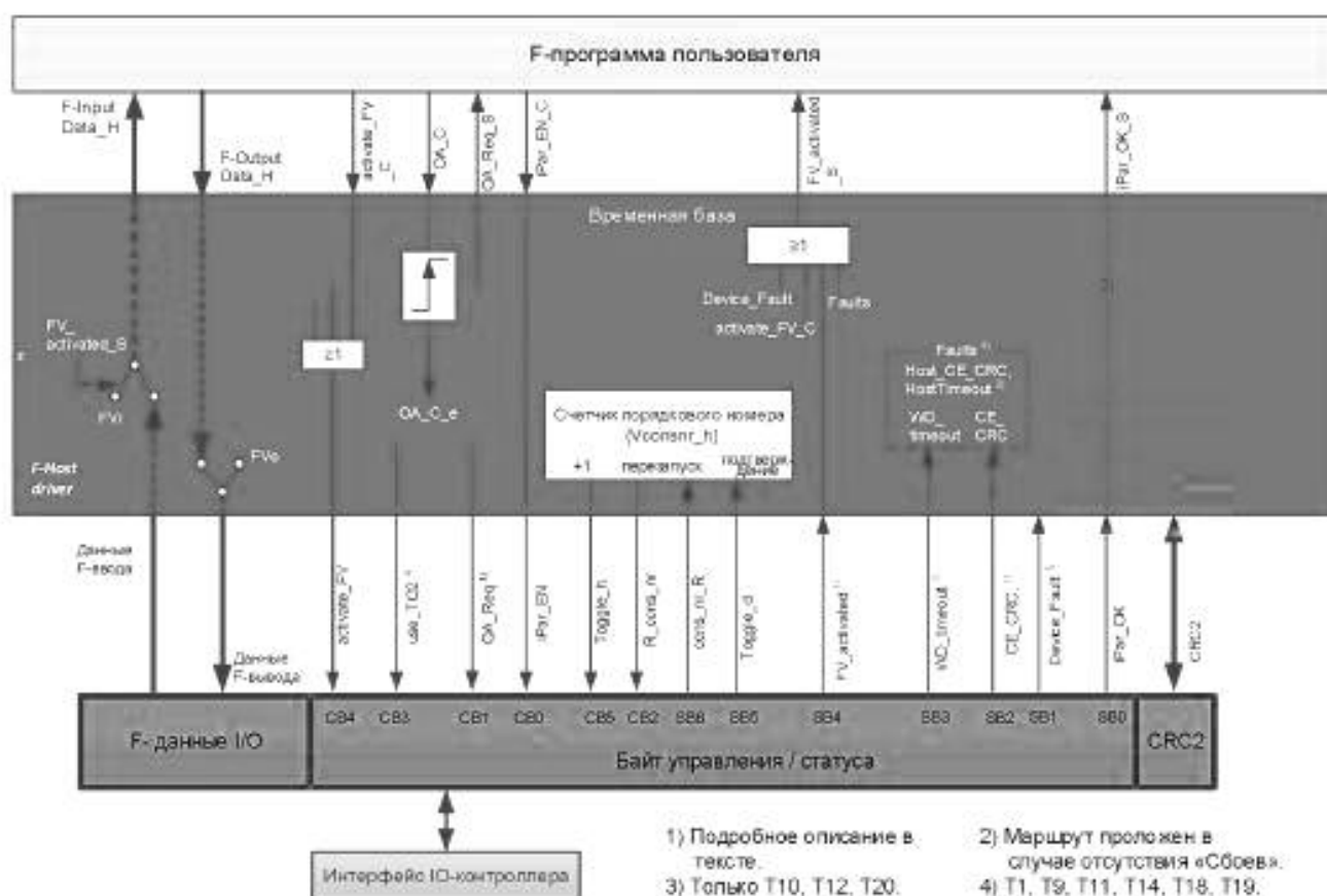
Рисунок 18 — F-интерфейс пользователя для экземпляров драйвера F-хоста
