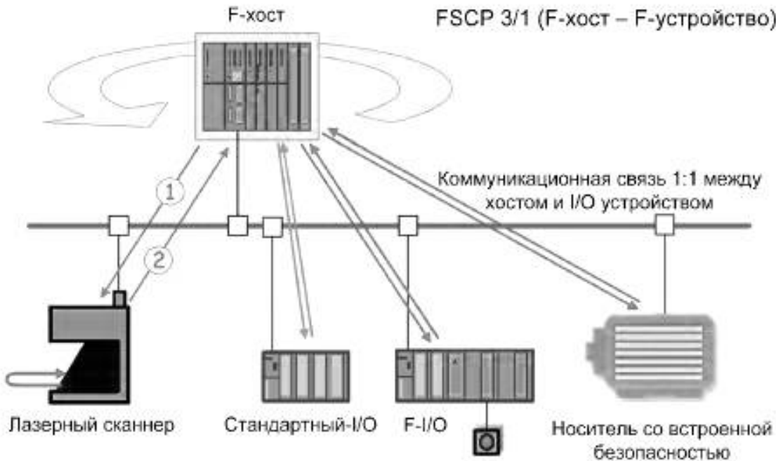
Рисунок 6 — Стандартная система передачи CPF 3
