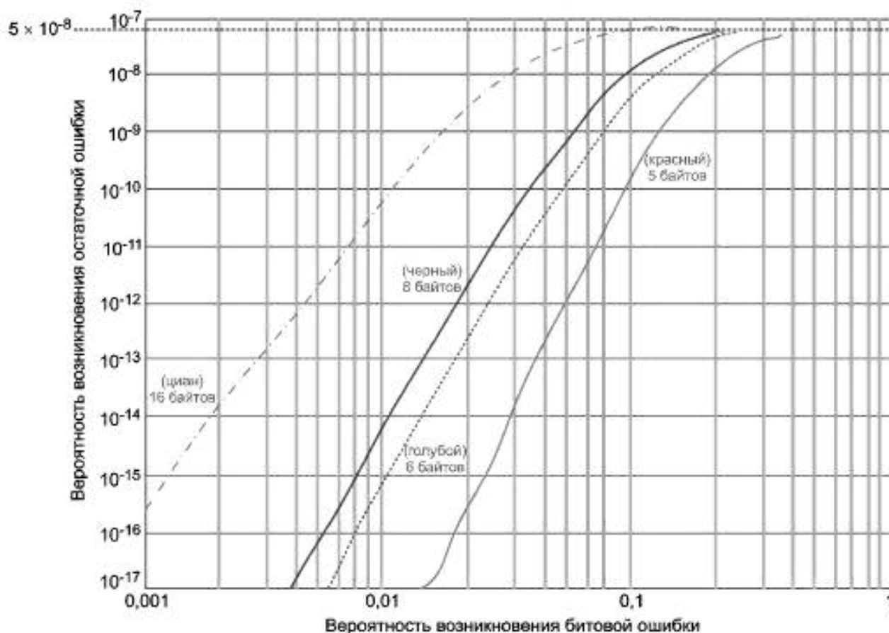
Рисунок 80 — Вероятности возникновения остаточной ошибки для 24-битового полинома
