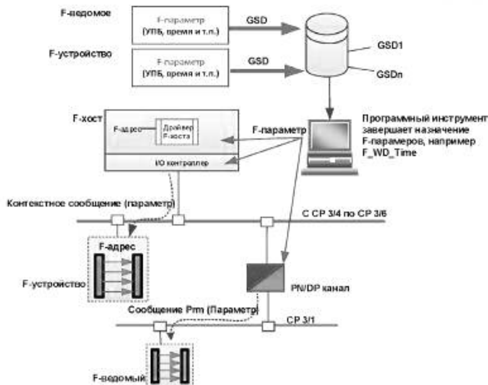
Рисунок 63 — Назначение F-параметров простым F-устройствам и F-ведомым устройствам
