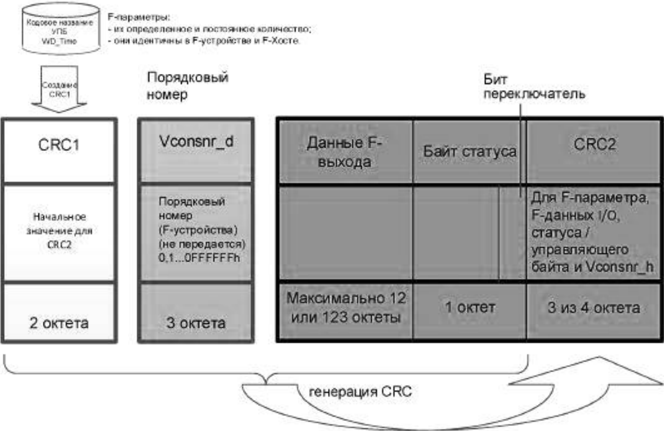
Рисунок 25 — Генерация CRC2 (вывод F-хоста)
