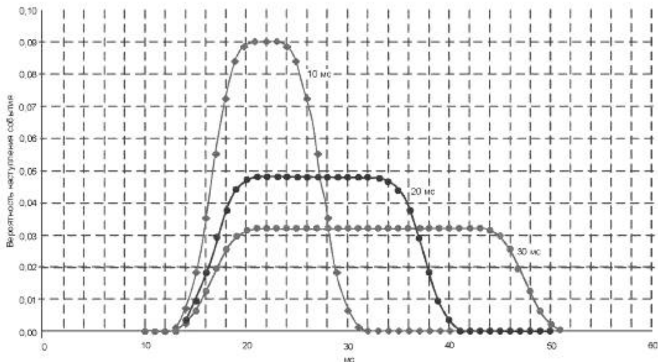
Рисунок 74 — Распределения частот типового времени реакции модели
