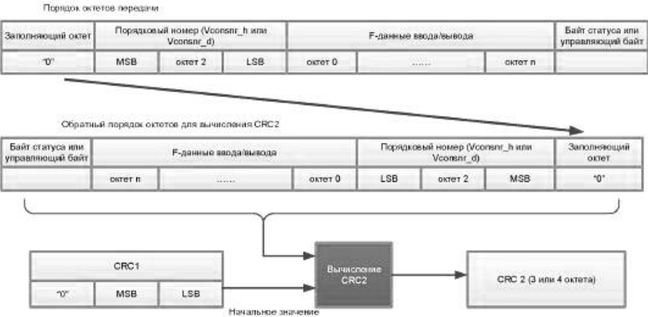
Рисунок 26 — Подробности вычисления CRC2 (обратный порядок)
