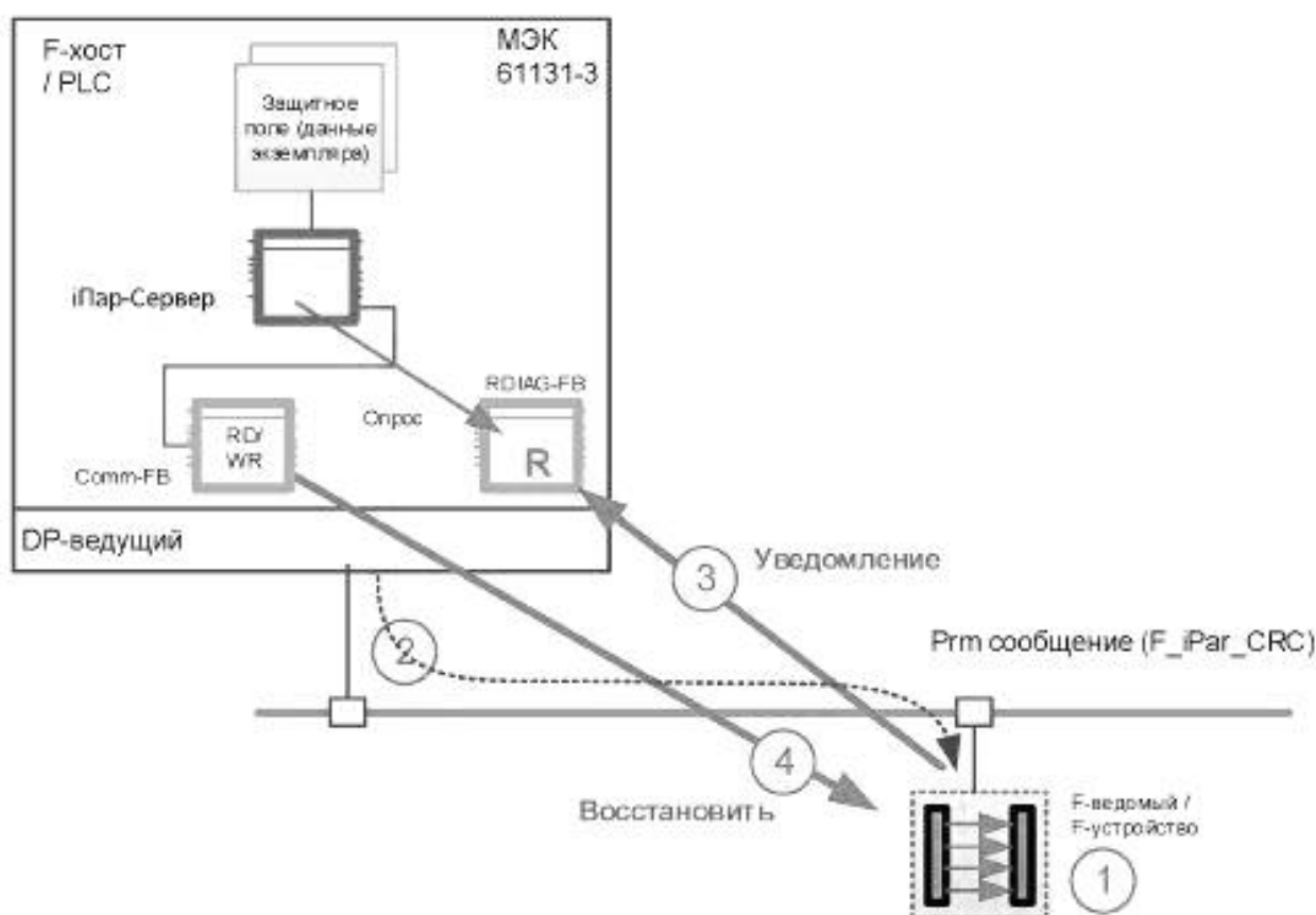
Рисунок 67 — Механизм iPar-сервера (например, замена F-устройства)
