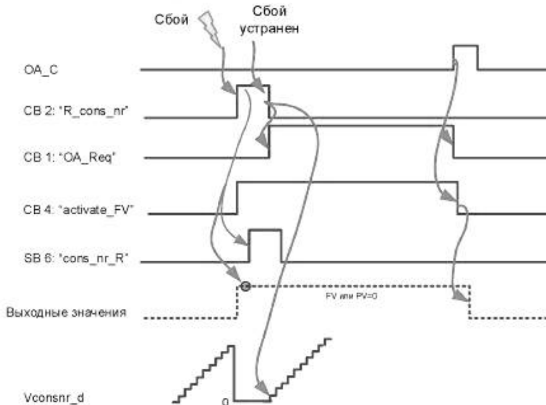
Рисунок 36 — Влияние сигнала сброса счетчика
