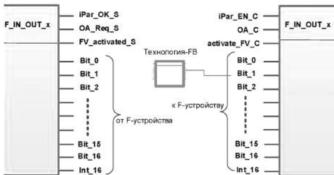
Рисунок 62 — Пример макета драйвера F-канала
