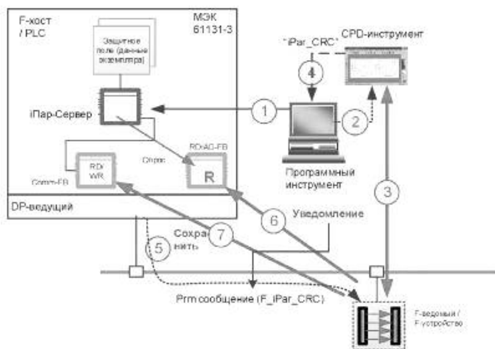
Рисунок 66 — Механизм iPar-сервера (ввод в эксплуатацию)
