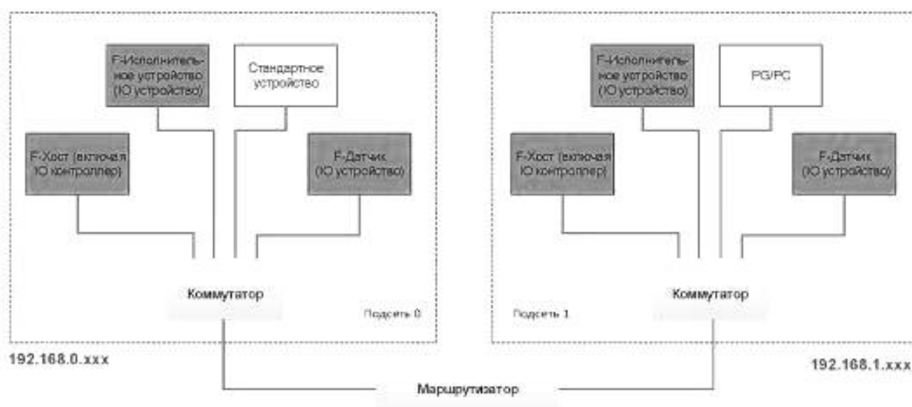
Рисунок 11 — Пересечение границ сети с маршрутизаторами
