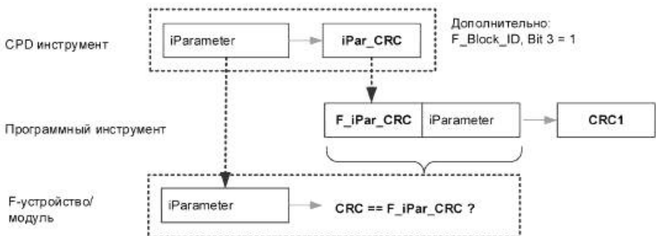
Рисунок 54 — CRC1, включая iPar_CRC
