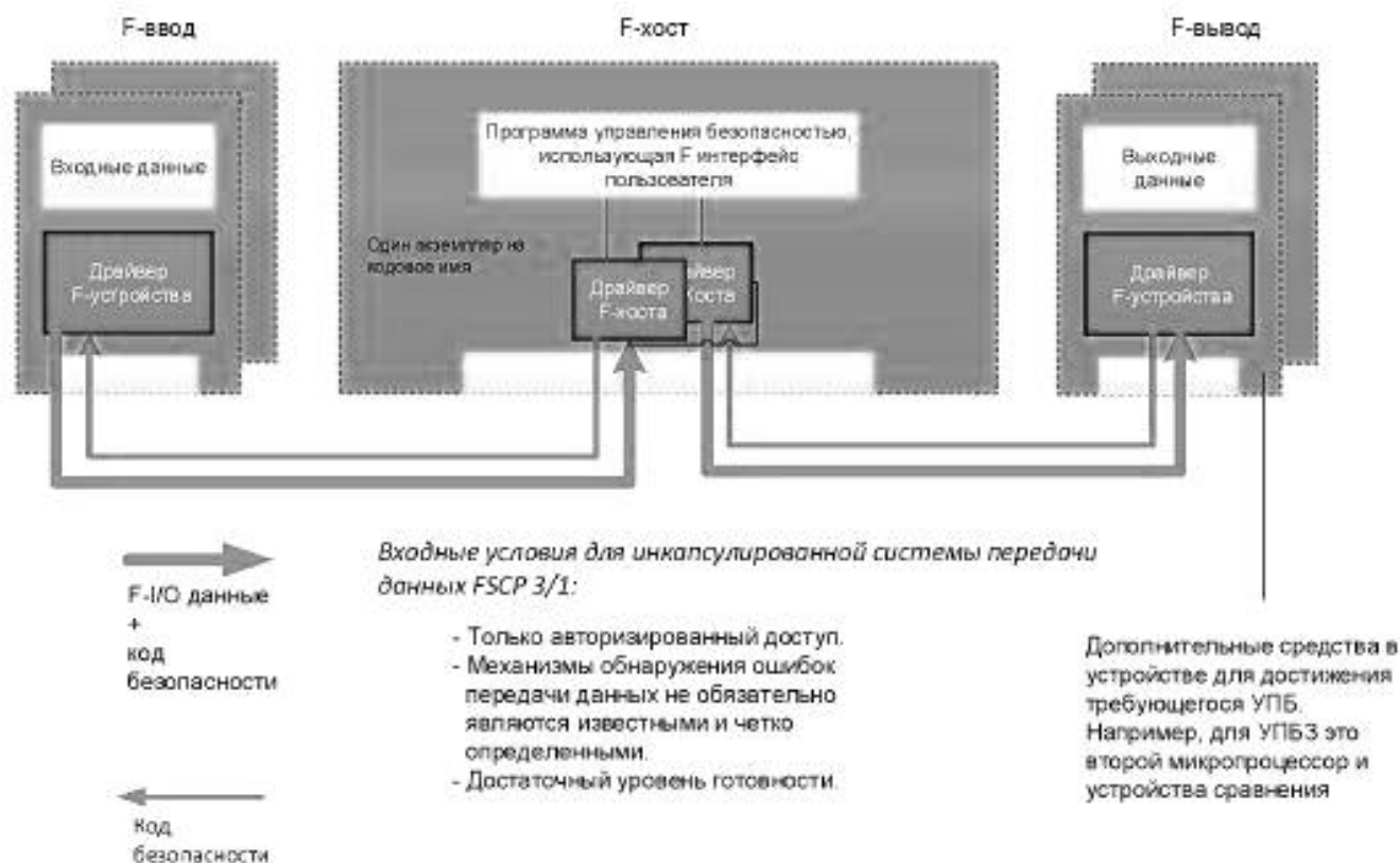
Рисунок 17 — Структура коммуникаций FSCP 3/1
