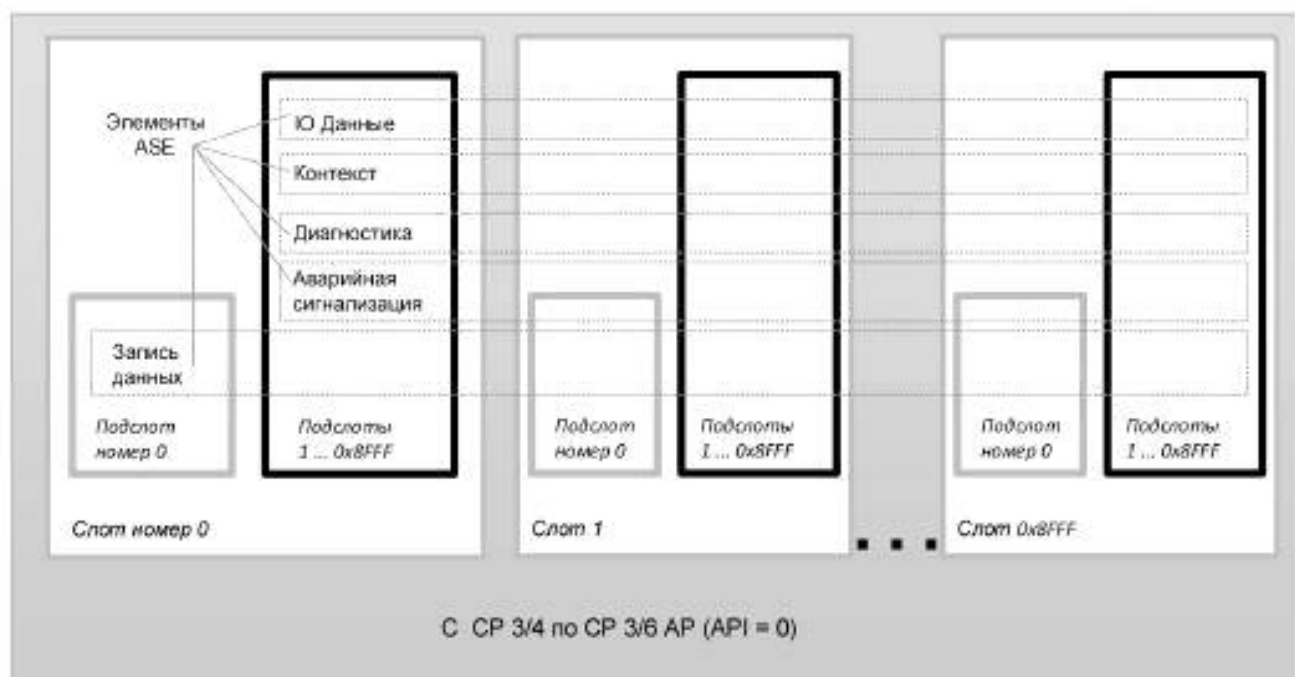
Рисунок 13 — Модель устройства
