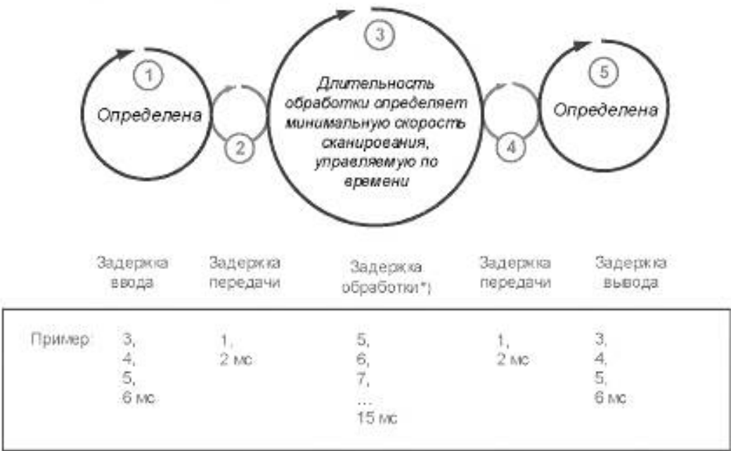
Рисунок 73 — Упрощенная модель типового времени реакции
