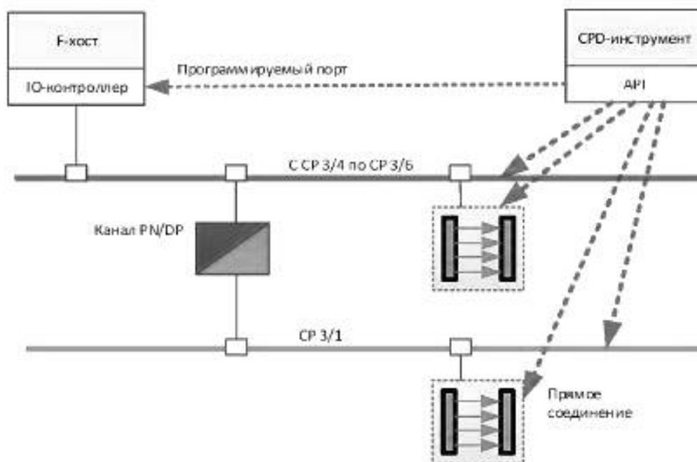
Рисунок 65 — Интеграция системы CPD-инструментов
