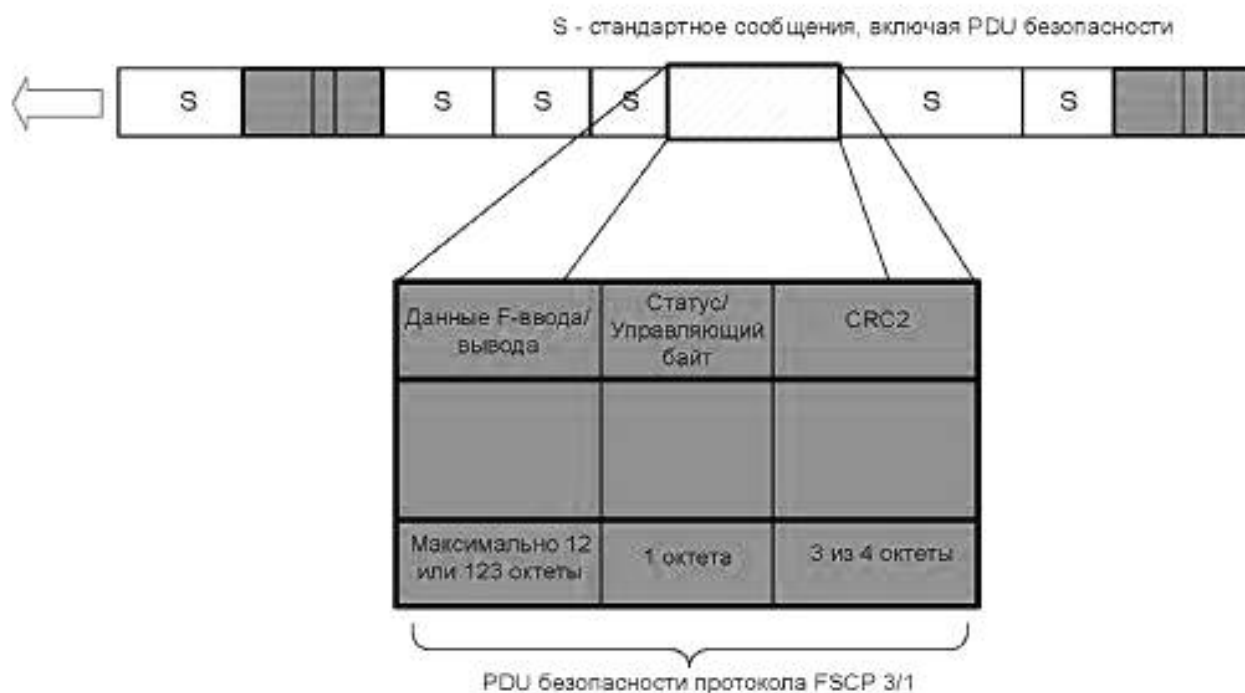
Рисунок 4 — Структура PDU безопасности FSCP 3/1
