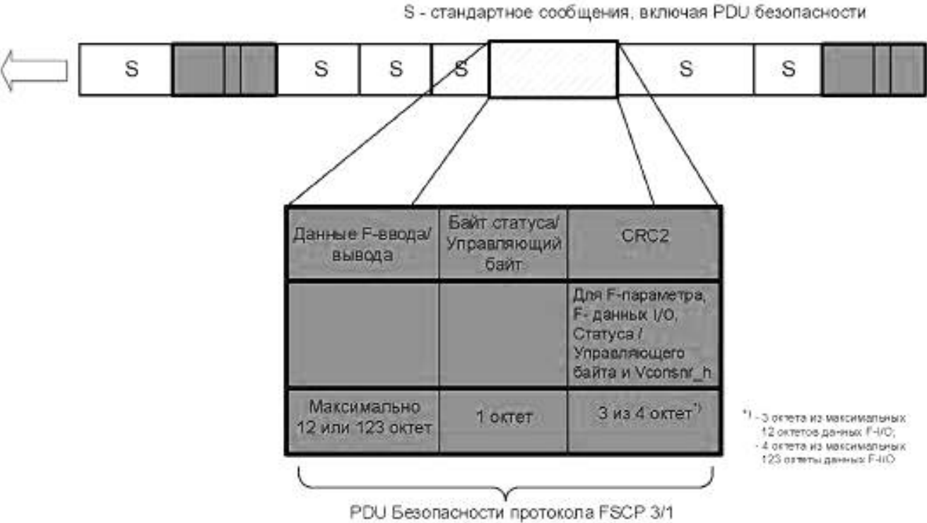
Рисунок 20 — PDU безопасности для CPF 3
