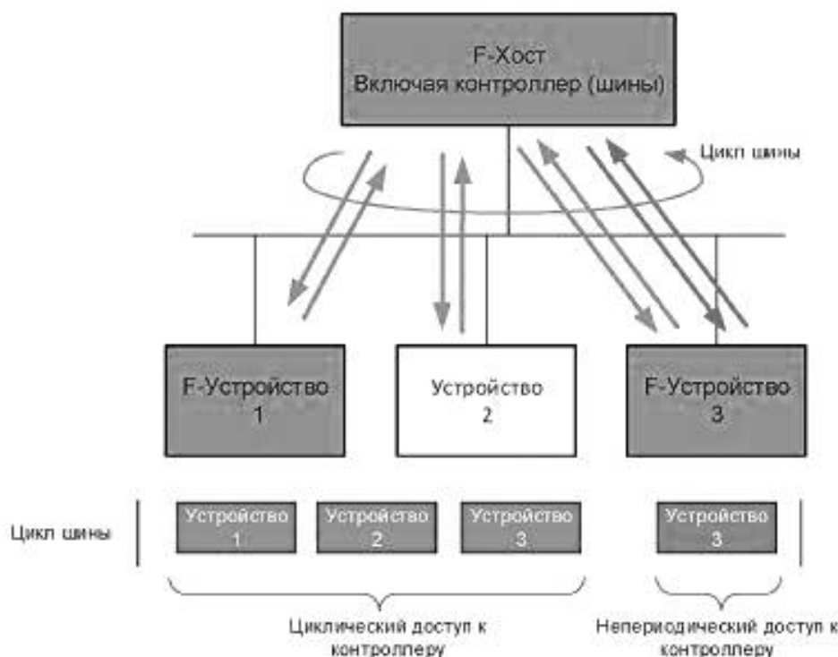
Рисунок 3 — Базовые предварительные условия для коммуникаций в FSCP 3/1
