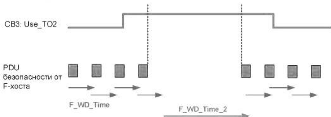
Рисунок 42 — Эффект F_WD_Time_2
