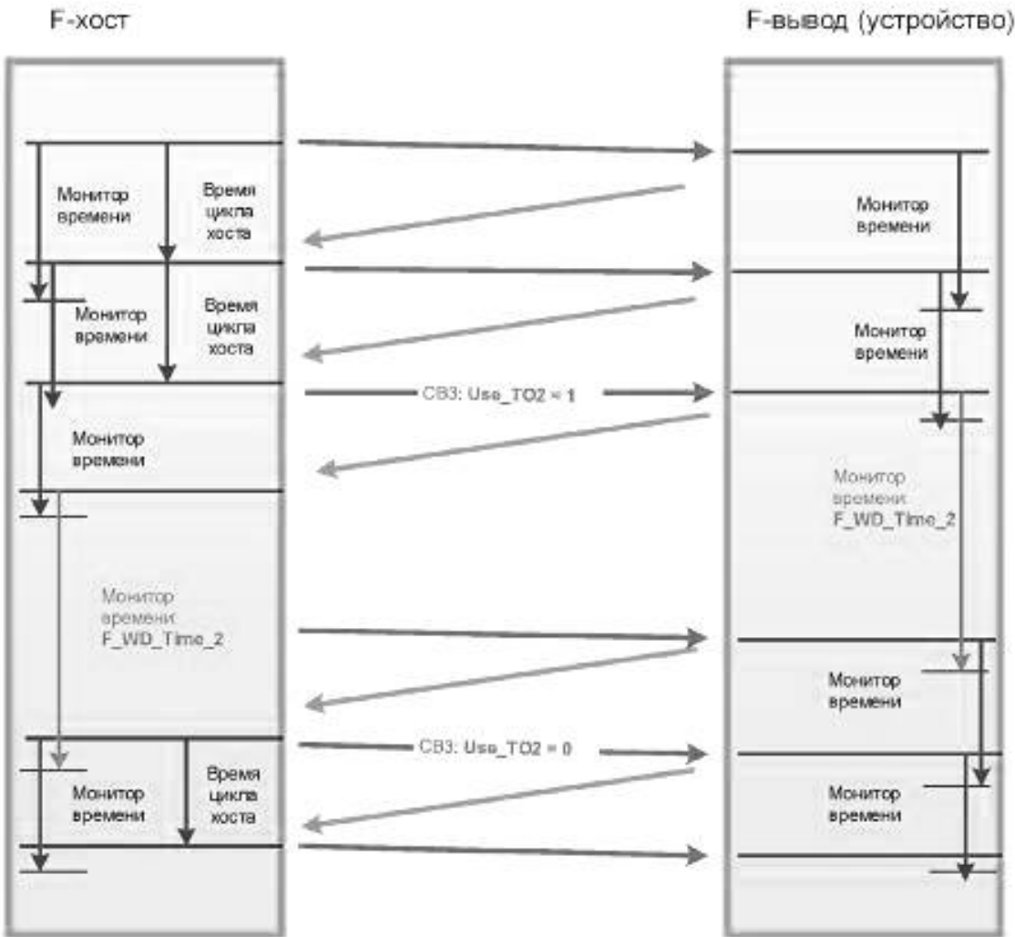
Рисунок 39 — Расширенное время сторожевого таймера по запросу
