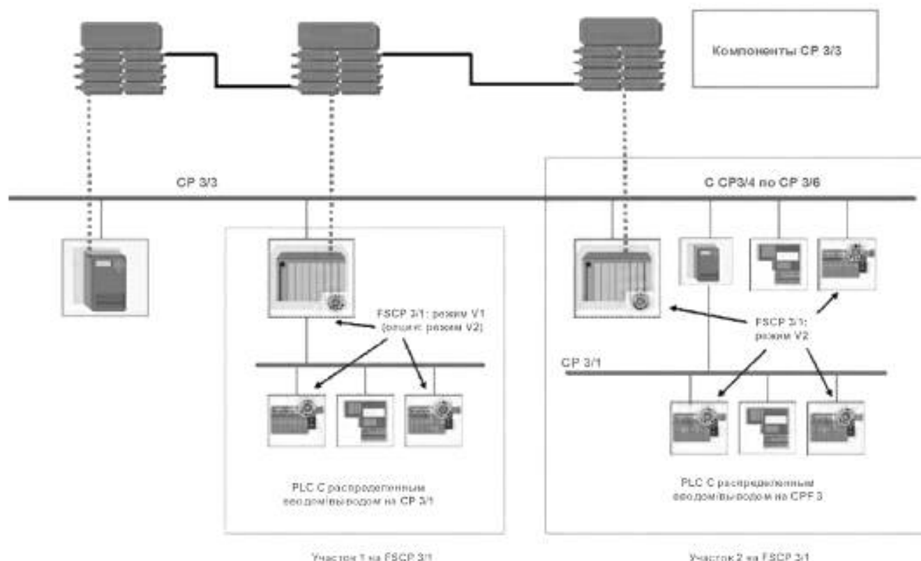
Рисунок 5 — Режимы коммуникаций безопасности
