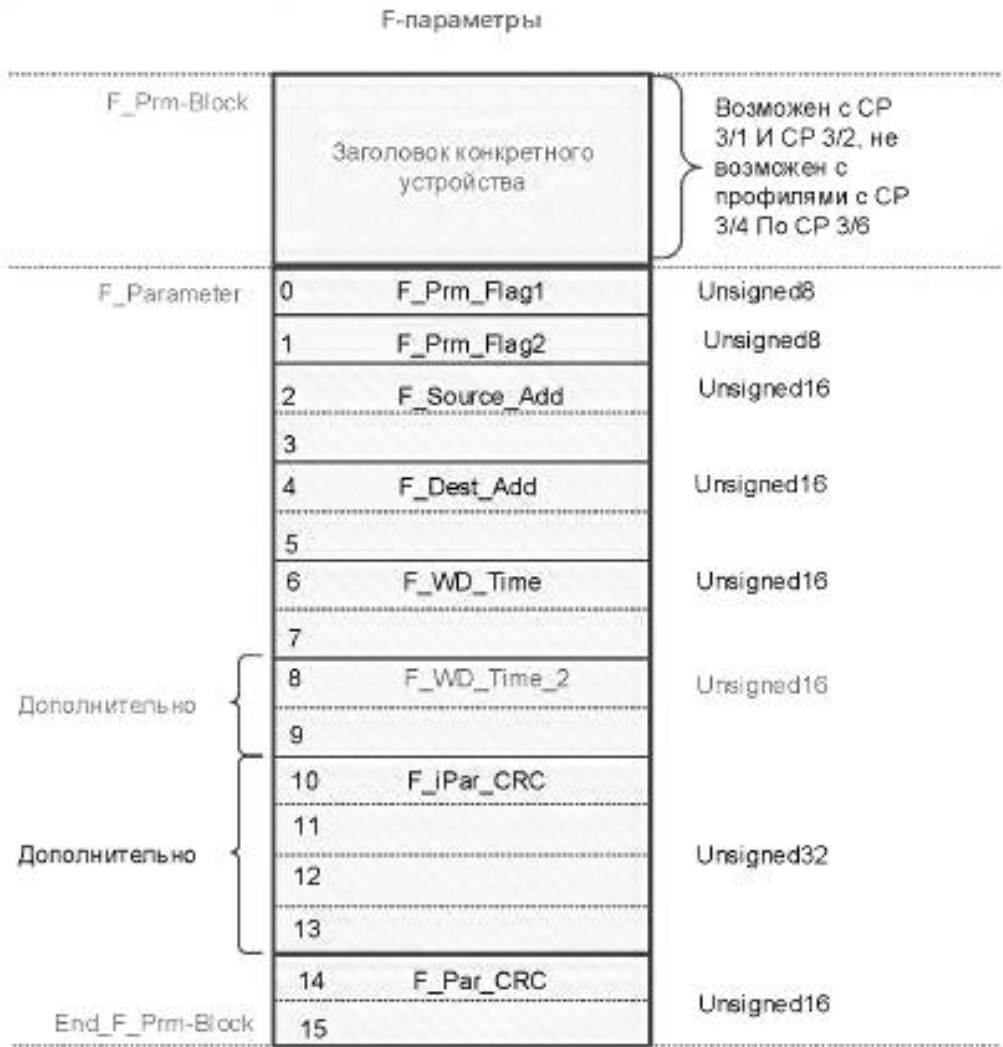
Рисунок 51 — F-параметр
