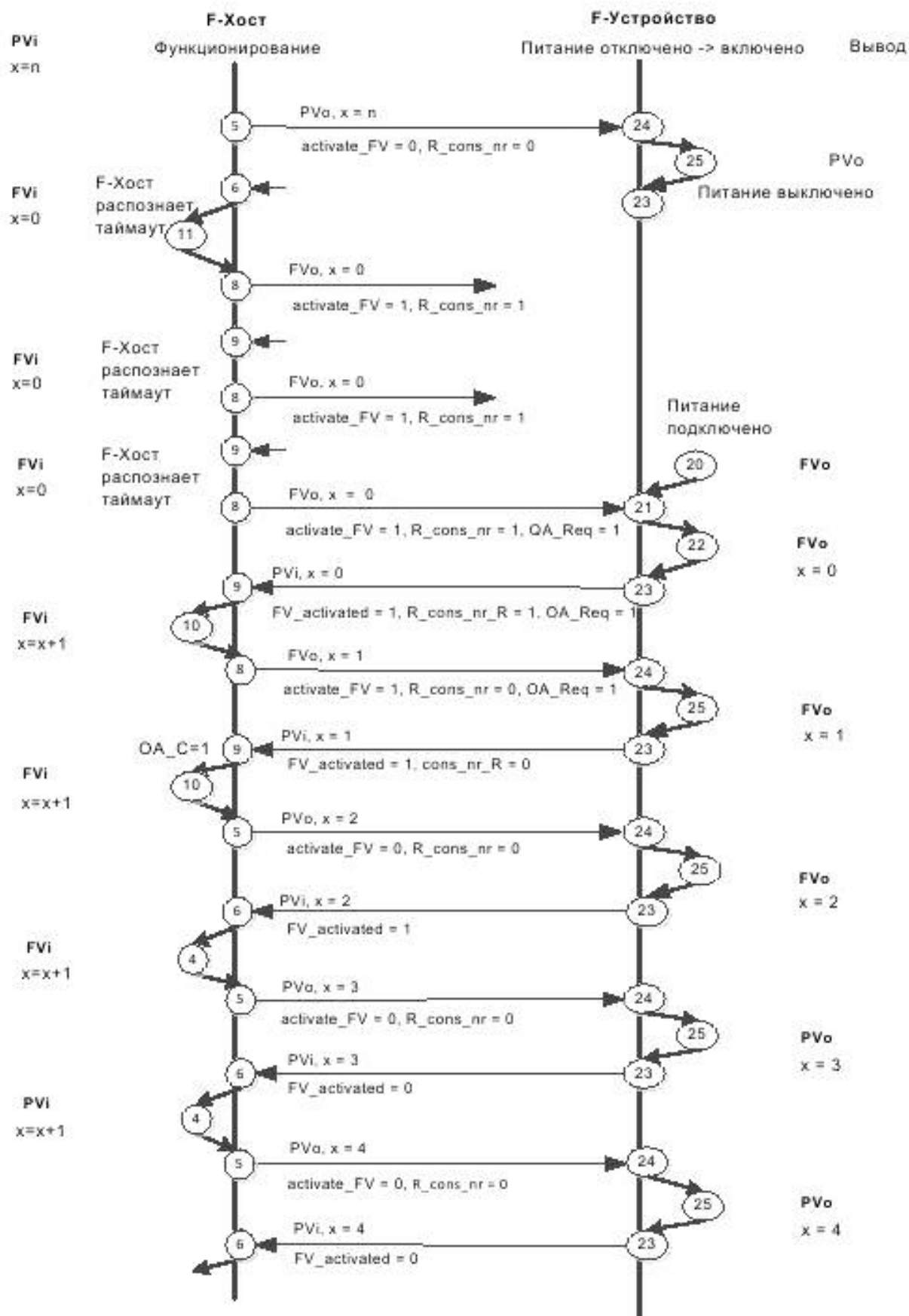
Рисунок 33 — Взаимодействие F-хоста / F-устройства во время отключения → включения питания
