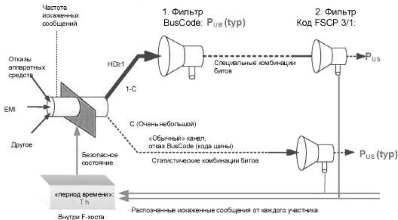
Рисунок 83 — Контроль искаженных сообщений
