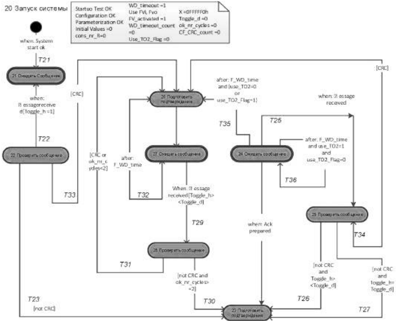
Рисунок 29 — Диаграмма состояний F-устройства
