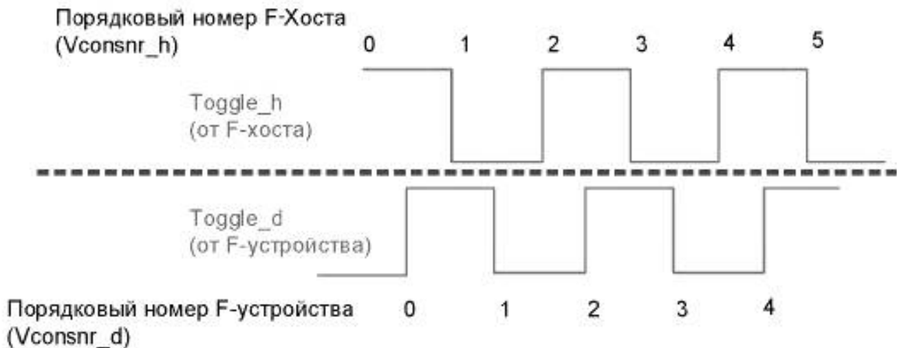
Рисунок 23 — Функция бита переключателя
