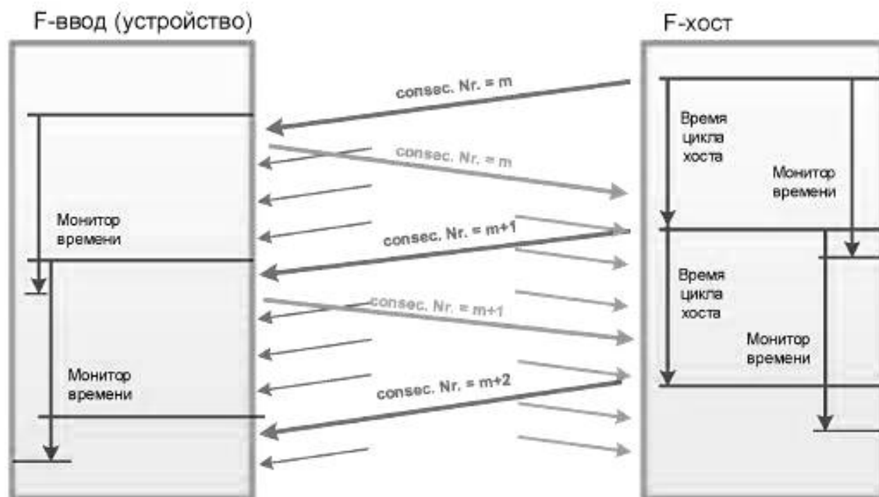
Рисунок 38 — Контроль времени передачи сообщения для передачи F-ввод ↔ F-хост
