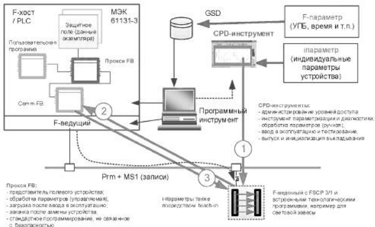
Рисунок 64 — Назначение F и параметров для сложных F-устройств
