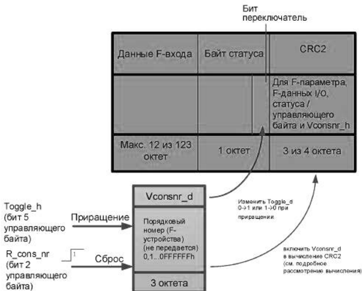
Рисунок 24 — Порядковый номер F-устройства
