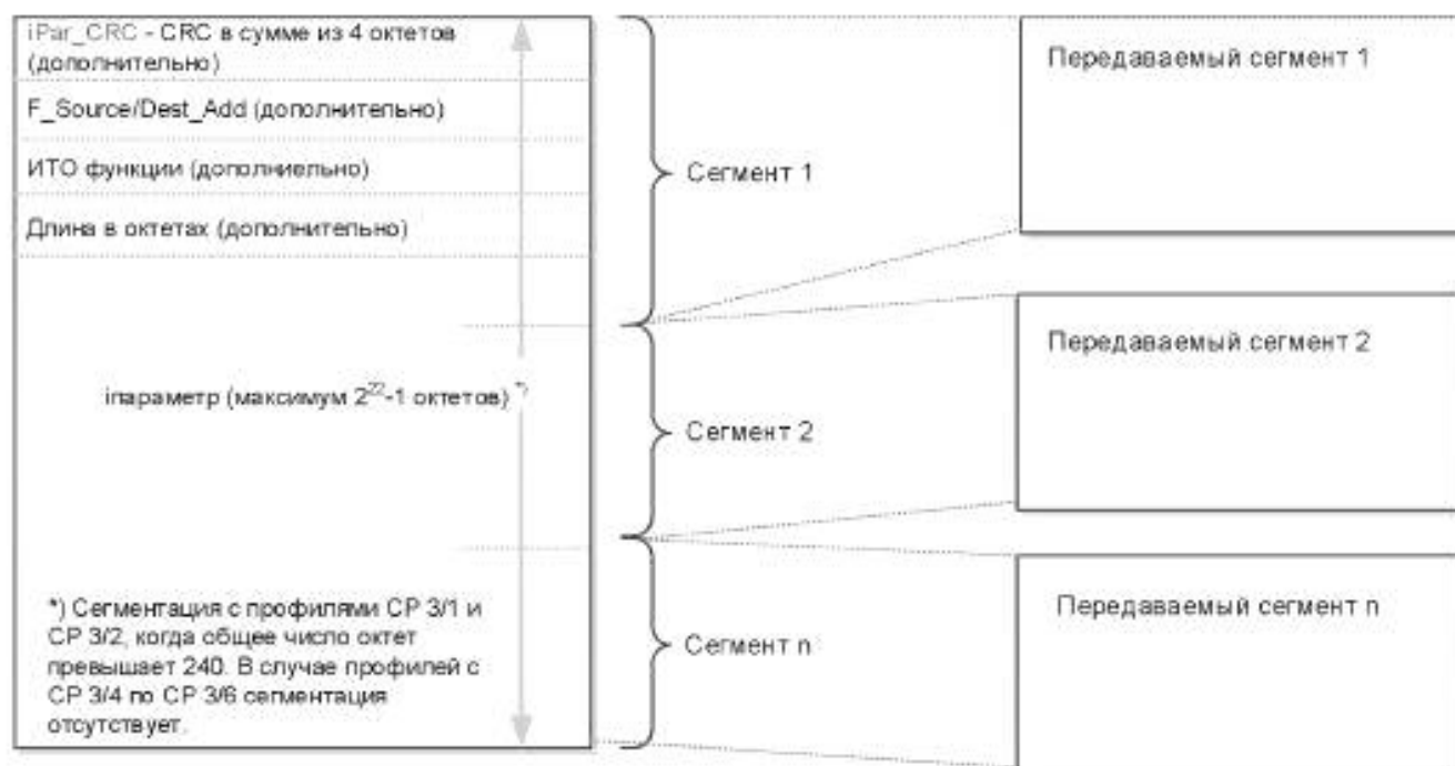
Рисунок 52 — Блок iпараметров
