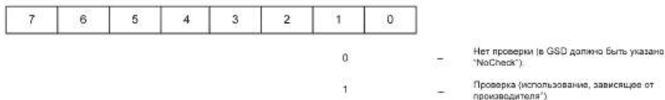
Рисунок 45 — F_Check_iPar
