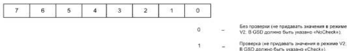
Рисунок 44 — F_Check_SeqNr
