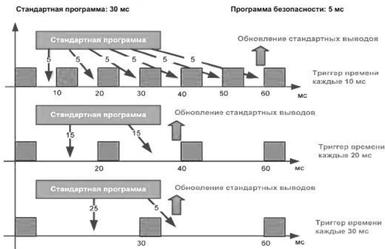
Рисунок A.3 — F-хост со стандартными и связанными с безопасностью прикладными программами
