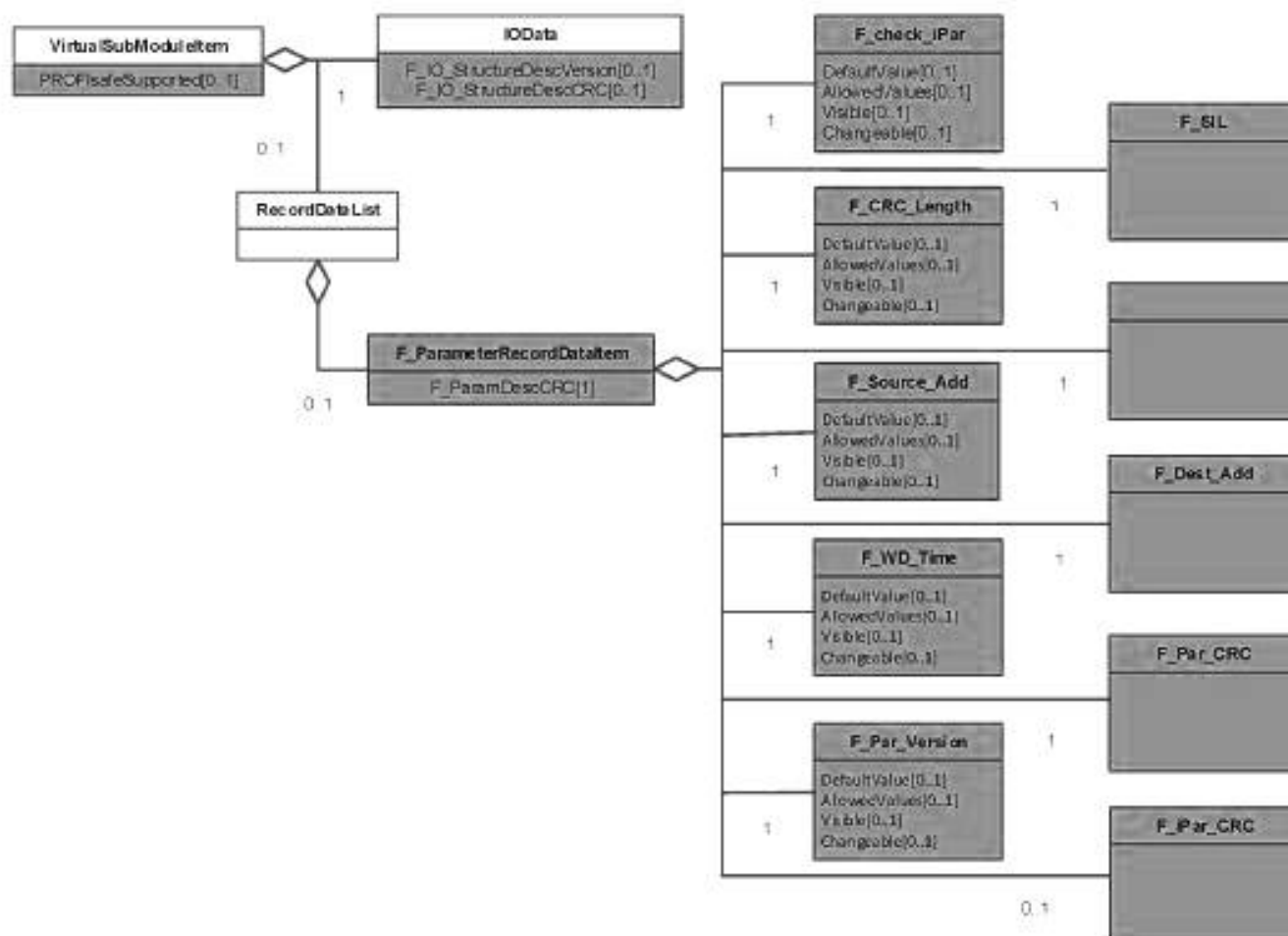
Рисунок 53 — Расширение F-параметра в спецификации GSDML
