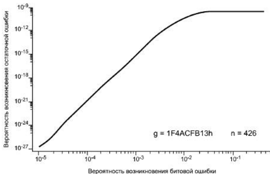
Рисунок 81 — Годность 32-битового полинома для 52 октетов
